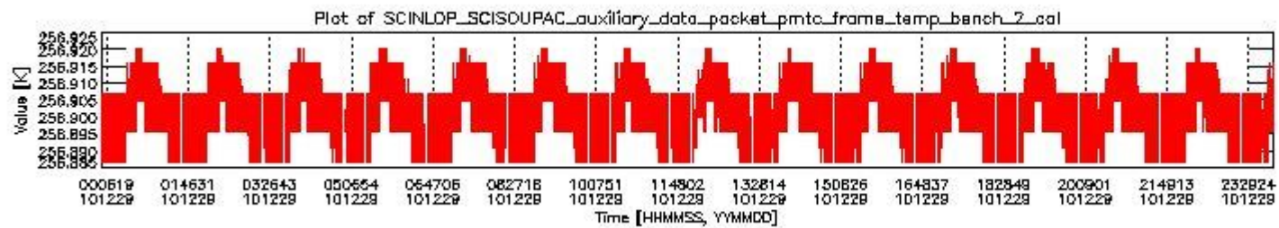
sciamachy_daily_report_level0_KSPT_L0_4504_N_20101229_1.PNG
