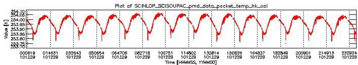
sciamachy_daily_report_level0_KSPT_L0_4504_N_20101229_3.PNG
