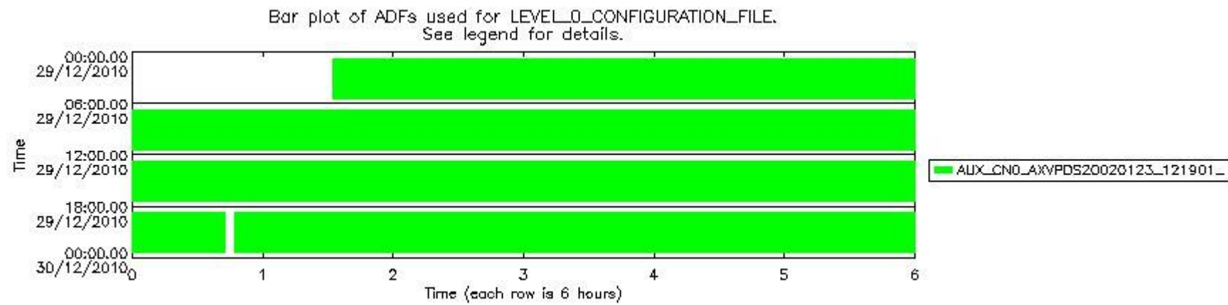
sciamachy_daily_report_level0_KSPT_L0_4504_N_20101229_6.PNG
