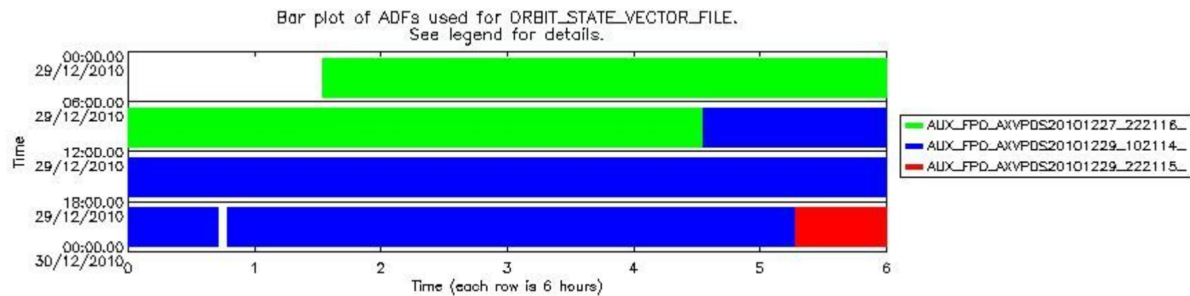
sciamachy_daily_report_level0_KSPT_L0_4504_N_20101229_7.PNG
