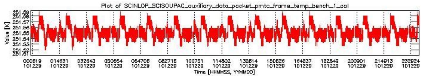
sciamachy_daily_report_level0_KSPT_L0_4504_N_20101229_0.PNG
