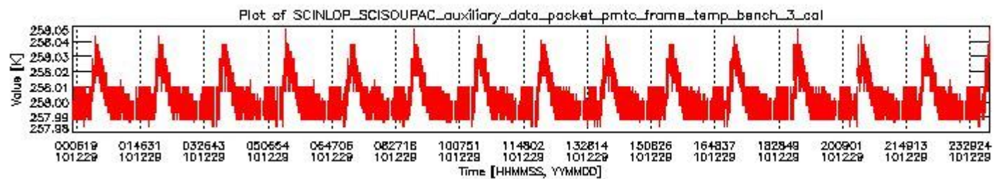
sciamachy_daily_report_level0_KSPT_L0_4504_N_20101229_2.PNG
