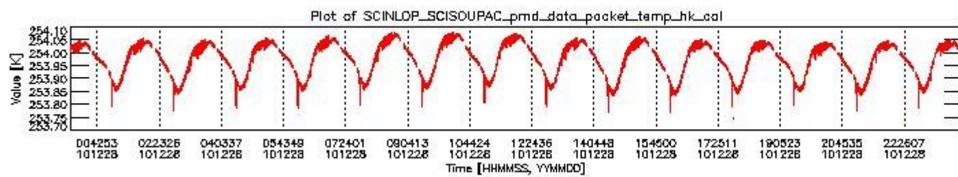
sciamachy_daily_report_level0_KSPT_L0_4504_N_20101228_3.PNG
