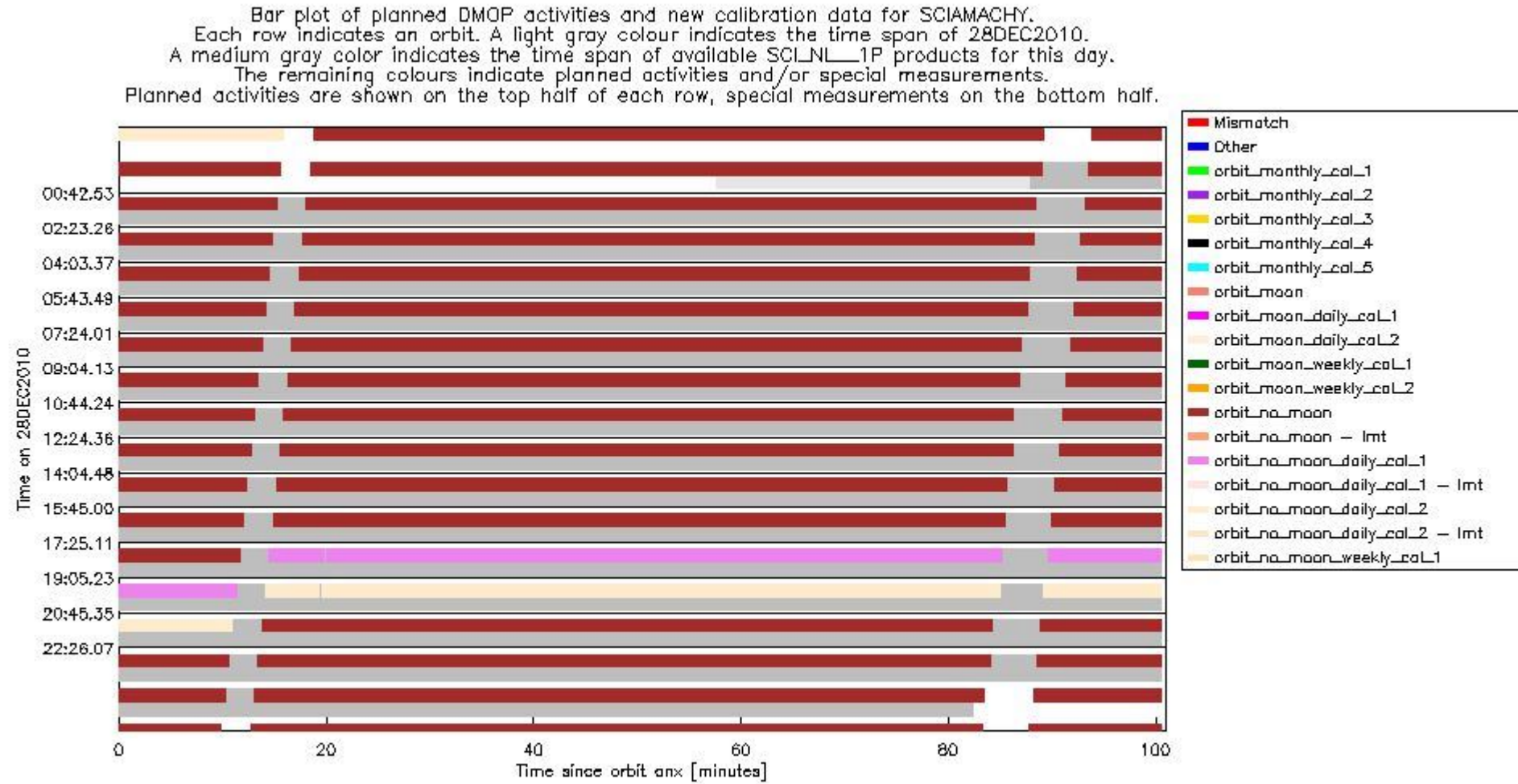
sciamachy_daily_report_level0_KSPT_L0_4504_N_20101228_5.PNG
