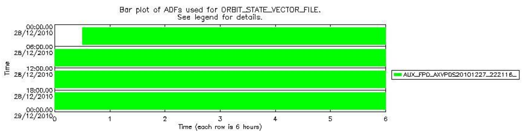
sciamachy_daily_report_level0_KSPT_L0_4504_N_20101228_7.PNG
