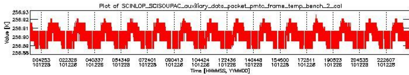
sciamachy_daily_report_level0_KSPT_L0_4504_N_20101228_1.PNG
