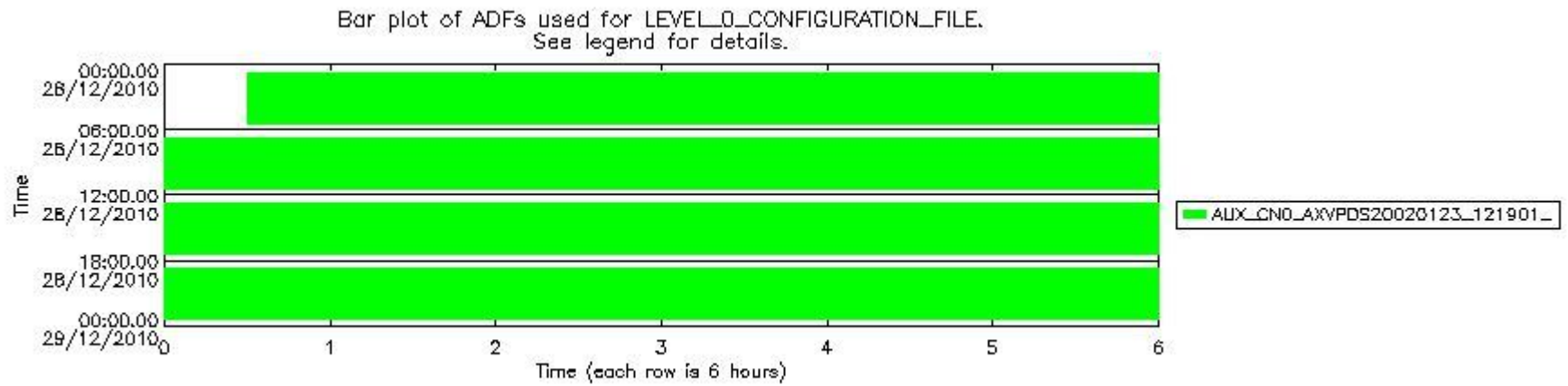
sciamachy_daily_report_level0_KSPT_L0_4504_N_20101228_6.PNG
