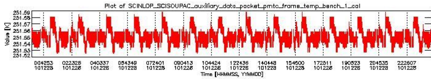
sciamachy_daily_report_level0_KSPT_L0_4504_N_20101228_0.PNG
