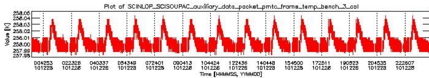
sciamachy_daily_report_level0_KSPT_L0_4504_N_20101228_2.PNG
