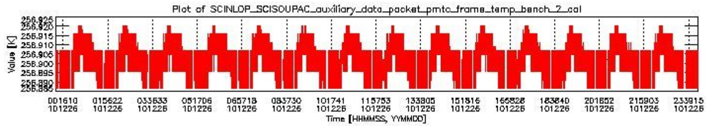
sciamachy_daily_report_level0_KSPT_L0_4504_N_20101226_1.PNG
