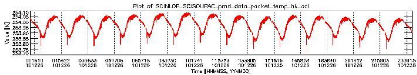
sciamachy_daily_report_level0_KSPT_L0_4504_N_20101226_3.PNG
