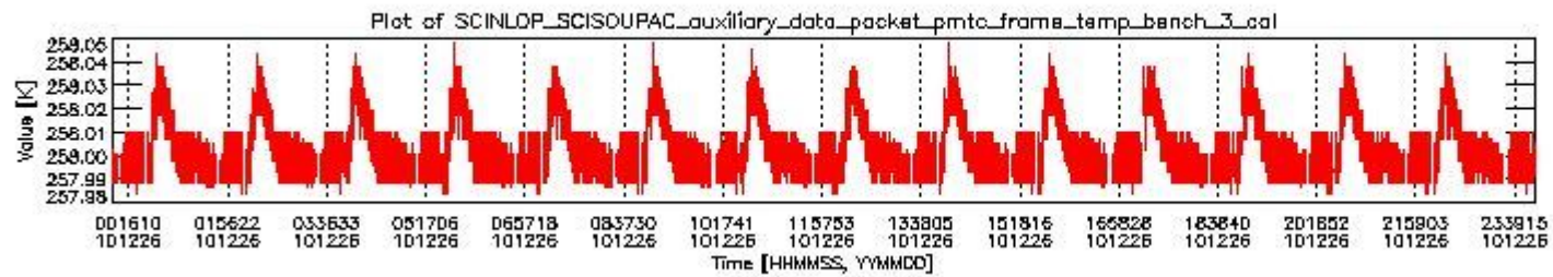
sciamachy_daily_report_level0_KSPT_L0_4504_N_20101226_2.PNG
