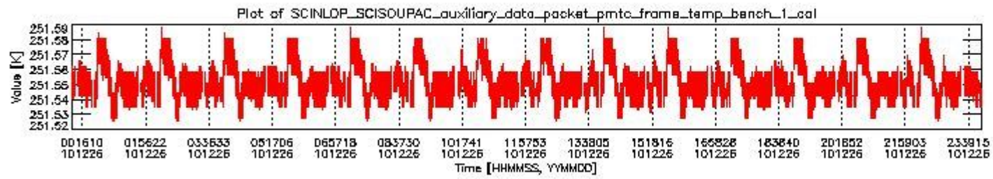
sciamachy_daily_report_level0_KSPT_L0_4504_N_20101226_0.PNG
