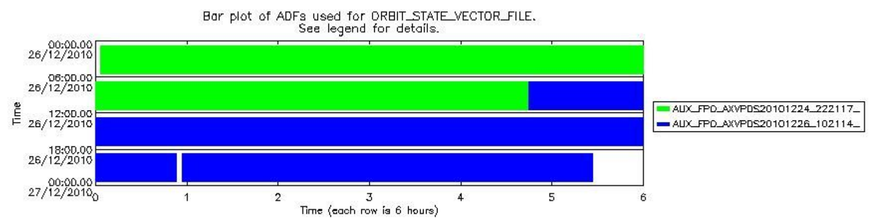
sciamachy_daily_report_level0_KSPT_L0_4504_N_20101226_7.PNG
