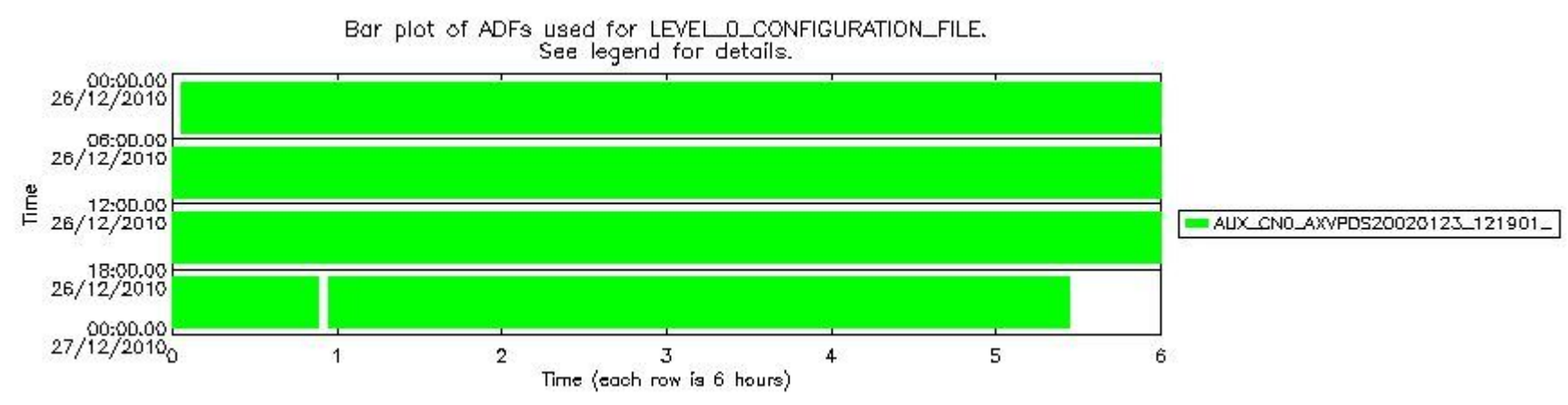
sciamachy_daily_report_level0_KSPT_L0_4504_N_20101226_6.PNG
