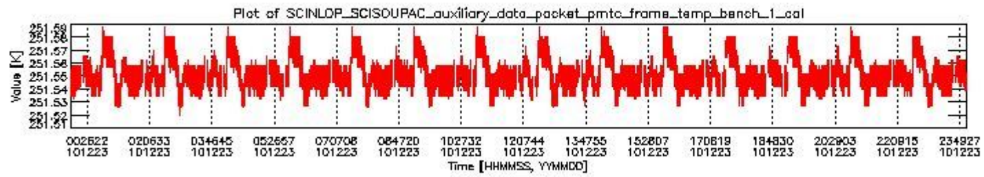
sciamachy_daily_report_level0_KSPT_L0_4504_N_20101223_0.PNG
