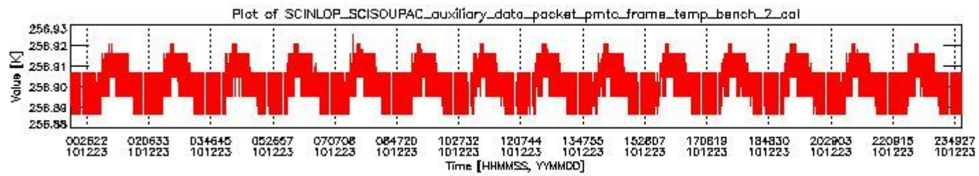
sciamachy_daily_report_level0_KSPT_L0_4504_N_20101223_1.PNG
