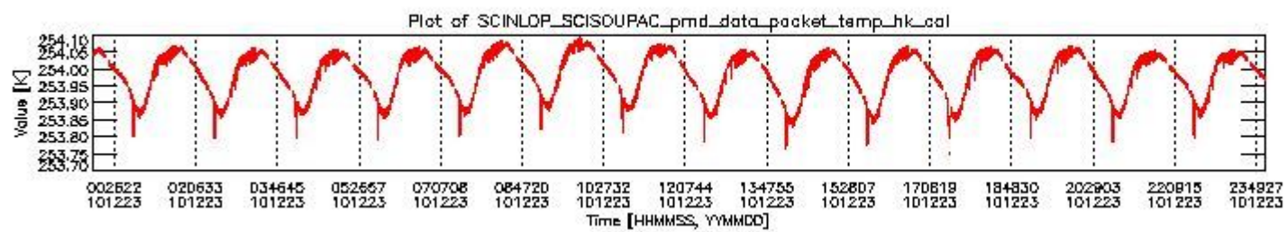
sciamachy_daily_report_level0_KSPT_L0_4504_N_20101223_3.PNG
