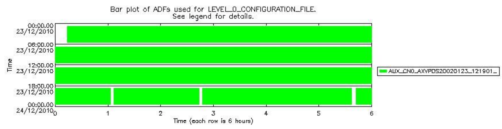
sciamachy_daily_report_level0_KSPT_L0_4504_N_20101223_6.PNG
