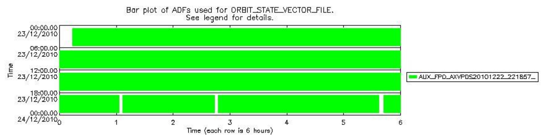
sciamachy_daily_report_level0_KSPT_L0_4504_N_20101223_7.PNG
