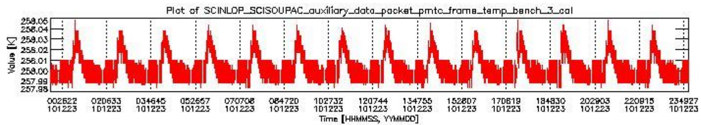
sciamachy_daily_report_level0_KSPT_L0_4504_N_20101223_2.PNG
