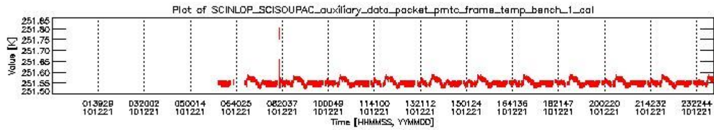
sciamachy_daily_report_level0_KSPT_L0_4504_N_20101221_0.PNG
