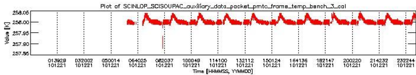
sciamachy_daily_report_level0_KSPT_L0_4504_N_20101221_2.PNG
