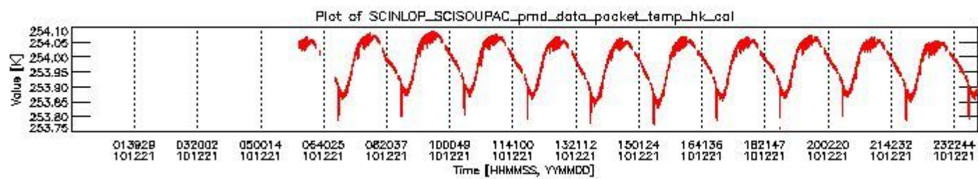
sciamachy_daily_report_level0_KSPT_L0_4504_N_20101221_3.PNG
