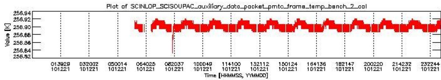
sciamachy_daily_report_level0_KSPT_L0_4504_N_20101221_1.PNG
