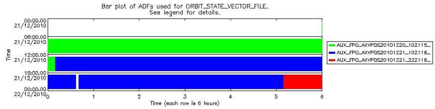
sciamachy_daily_report_level0_KSPT_L0_4504_N_20101221_7.PNG
