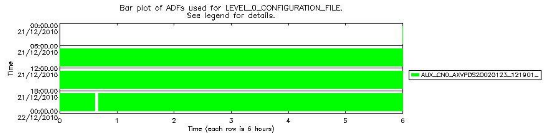
sciamachy_daily_report_level0_KSPT_L0_4504_N_20101221_6.PNG
