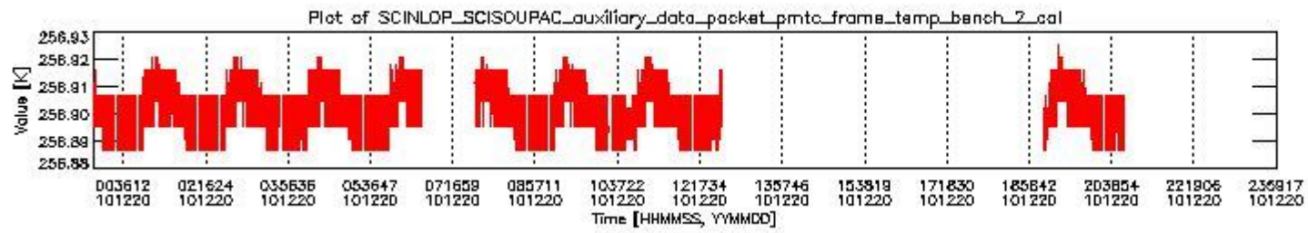
sciamachy_daily_report_level0_KSPT_L0_4504_N_20101220_1.PNG
