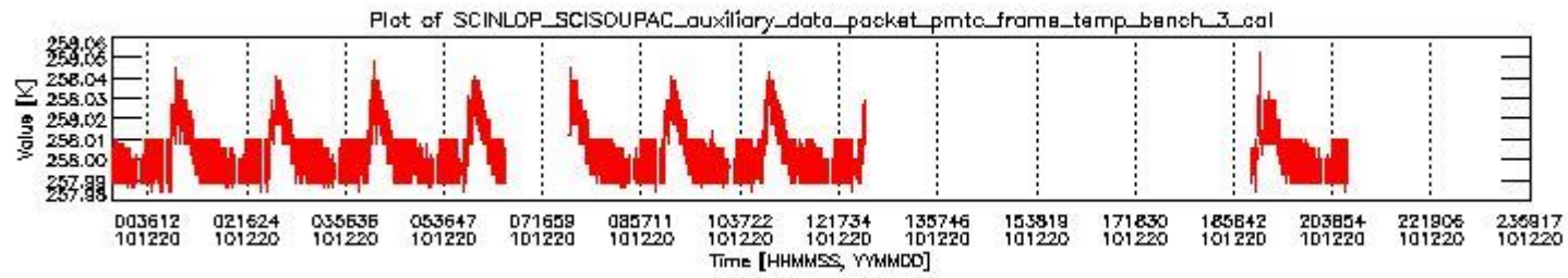
sciamachy_daily_report_level0_KSPT_L0_4504_N_20101220_2.PNG
