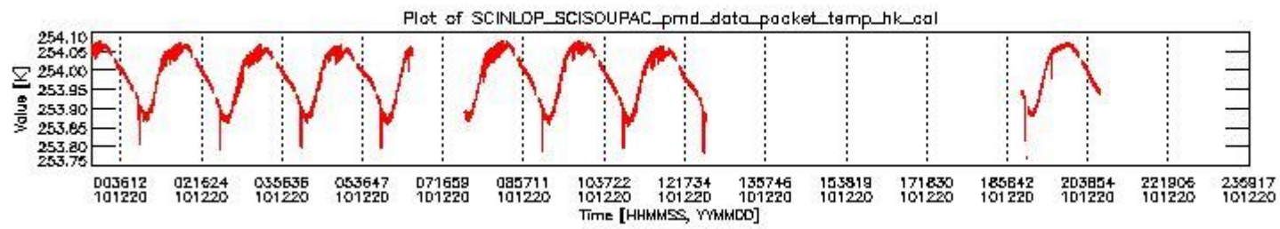
sciamachy_daily_report_level0_KSPT_L0_4504_N_20101220_3.PNG
