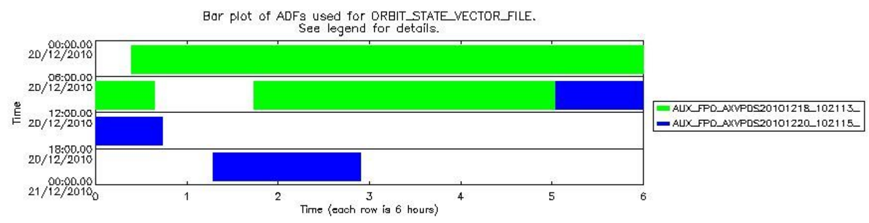
sciamachy_daily_report_level0_KSPT_L0_4504_N_20101220_7.PNG
