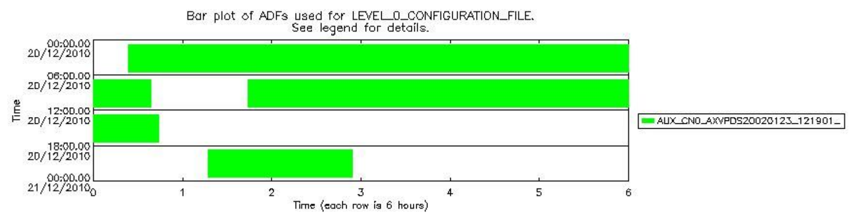
sciamachy_daily_report_level0_KSPT_L0_4504_N_20101220_6.PNG
