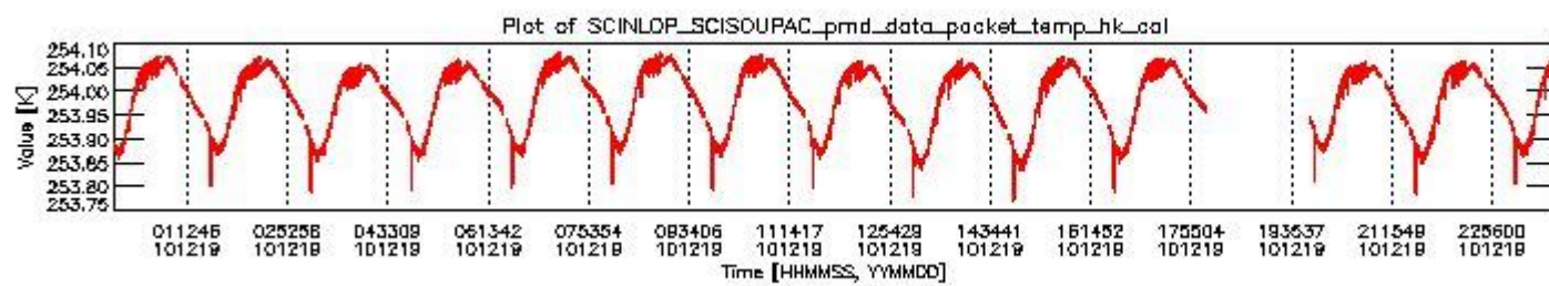
sciamachy_daily_report_level0_KSPT_L0_4504_N_20101219_3.PNG
