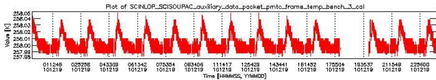
sciamachy_daily_report_level0_KSPT_L0_4504_N_20101219_2.PNG
