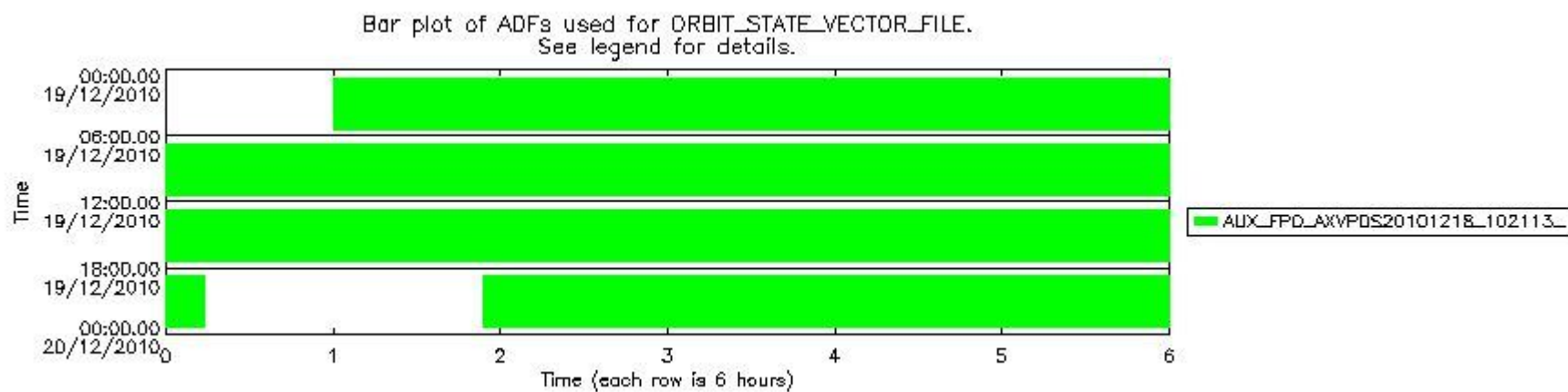
sciamachy_daily_report_level0_KSPT_L0_4504_N_20101219_6.PNG
