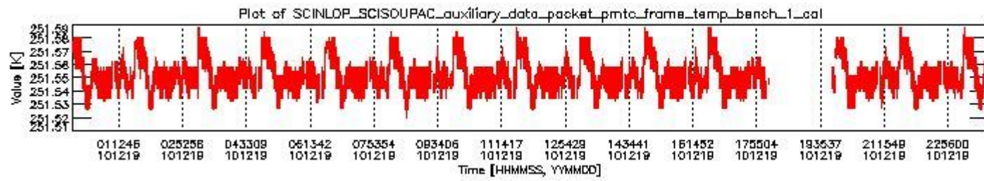
sciamachy_daily_report_level0_KSPT_L0_4504_N_20101219_0.PNG
