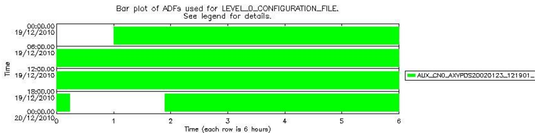
sciamachy_daily_report_level0_KSPT_L0_4504_N_20101219_5.PNG
