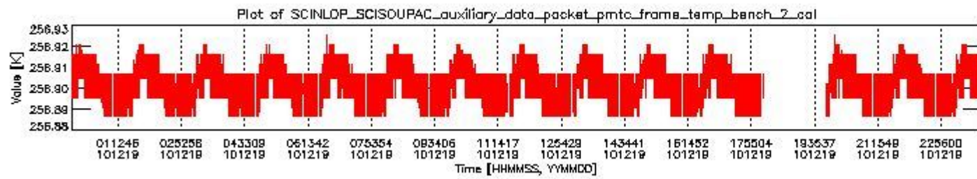
sciamachy_daily_report_level0_KSPT_L0_4504_N_20101219_1.PNG
