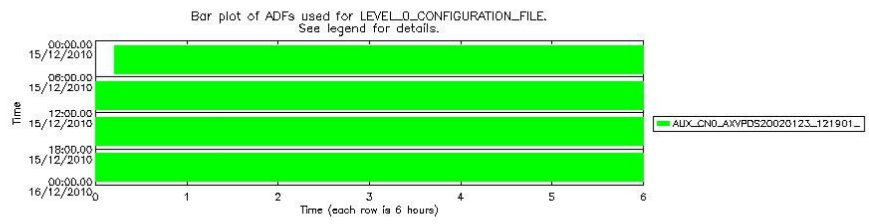
sciamachy_daily_report_level0_KSPT_L0_4504_N_20101215_6.PNG
