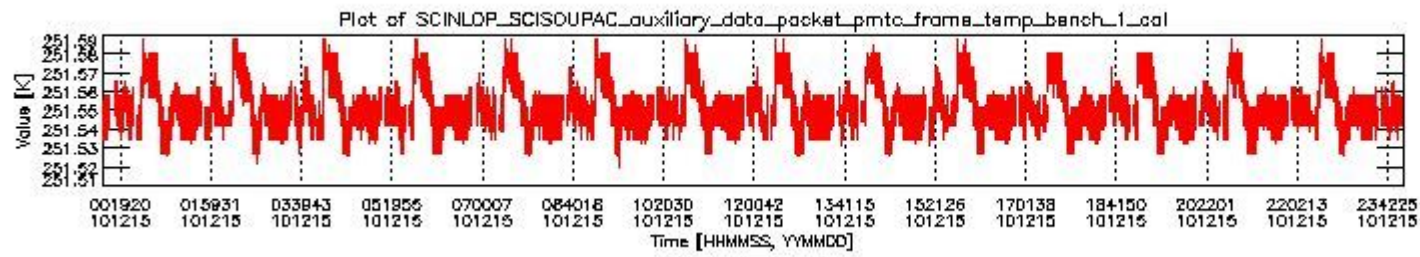
sciamachy_daily_report_level0_KSPT_L0_4504_N_20101215_0.PNG
