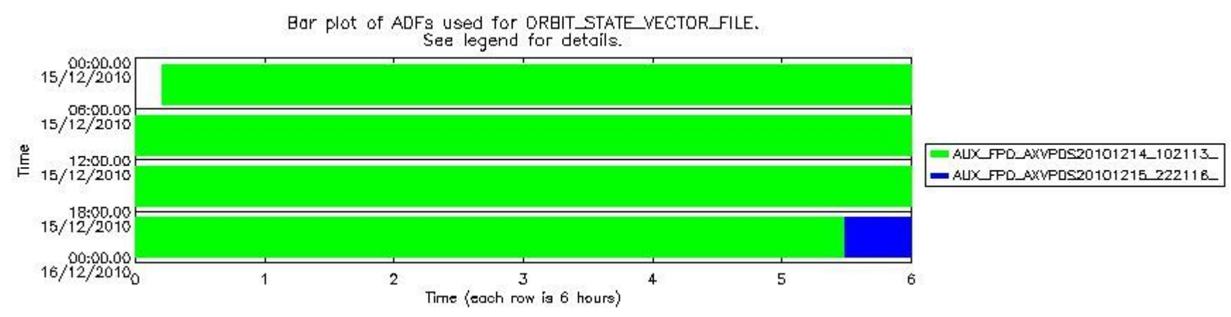
sciamachy_daily_report_level0_KSPT_L0_4504_N_20101215_7.PNG
