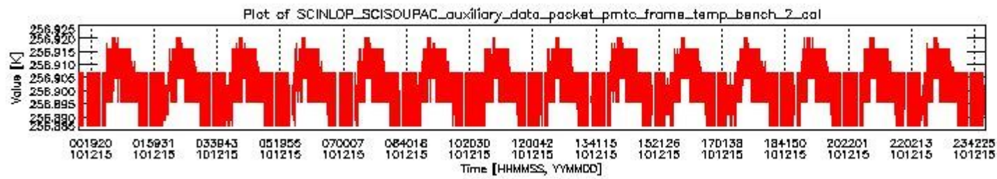
sciamachy_daily_report_level0_KSPT_L0_4504_N_20101215_1.PNG
