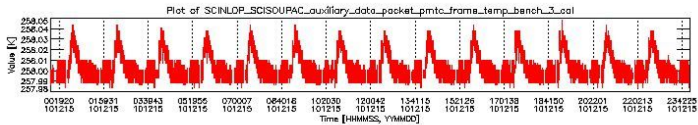
sciamachy_daily_report_level0_KSPT_L0_4504_N_20101215_2.PNG
