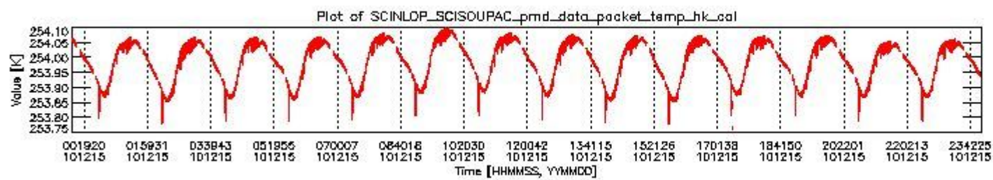
sciamachy_daily_report_level0_KSPT_L0_4504_N_20101215_3.PNG
