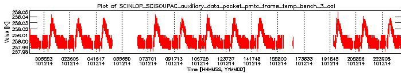
sciamachy_daily_report_level0_KSPT_L0_4504_N_20101214_2.PNG
