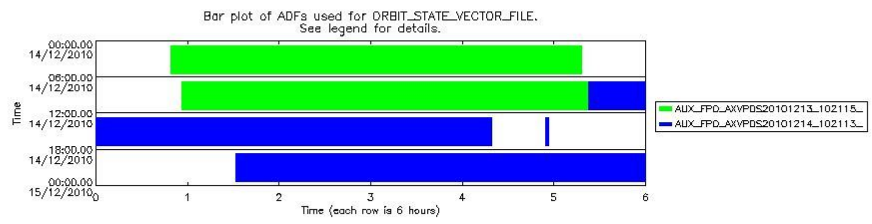
sciamachy_daily_report_level0_KSPT_L0_4504_N_20101214_8.PNG
