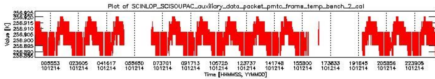
sciamachy_daily_report_level0_KSPT_L0_4504_N_20101214_1.PNG
