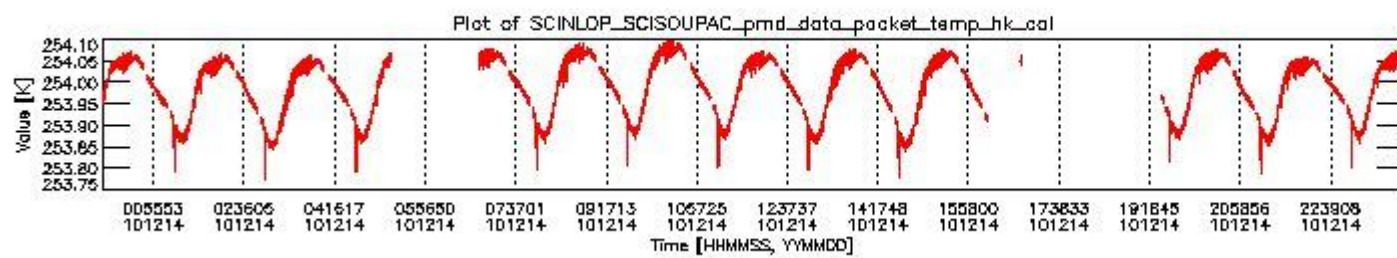
sciamachy_daily_report_level0_KSPT_L0_4504_N_20101214_3.PNG
