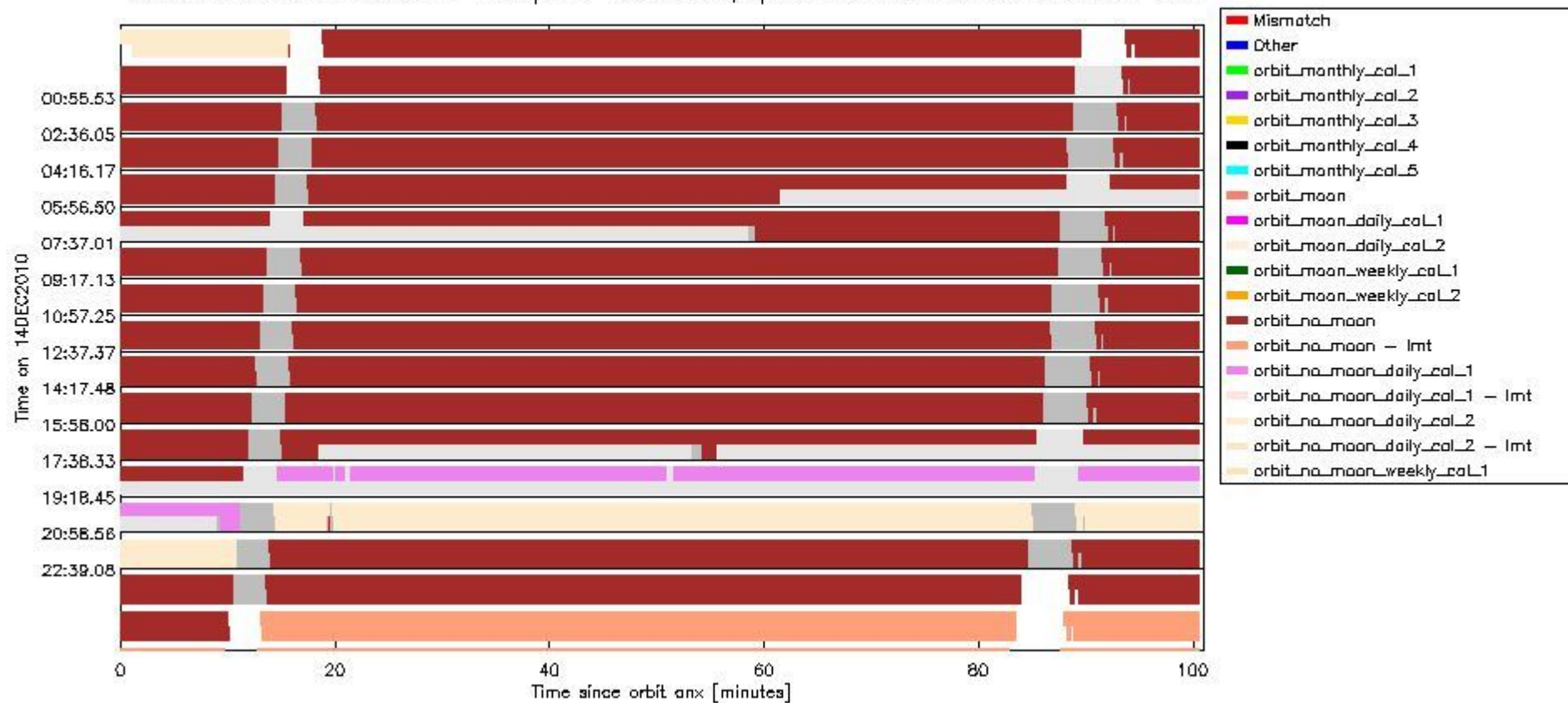
sciamachy_daily_report_level0_KSPT_L0_4504_N_20101214_6.PNG
