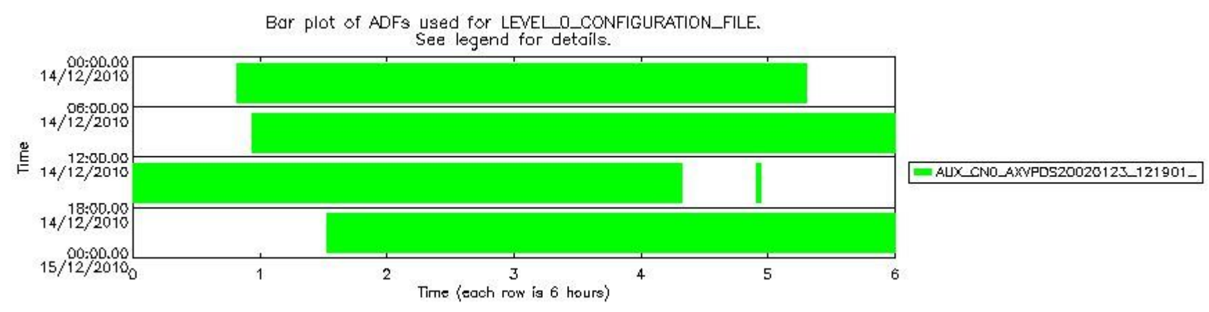
sciamachy_daily_report_level0_KSPT_L0_4504_N_20101214_7.PNG
