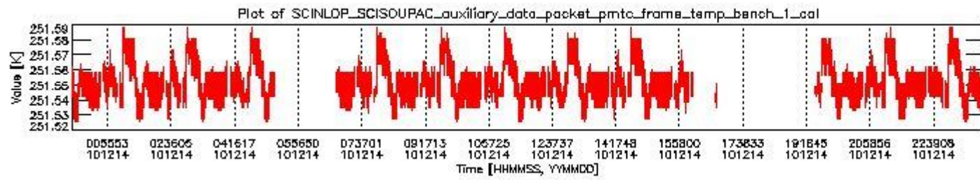
sciamachy_daily_report_level0_KSPT_L0_4504_N_20101214_0.PNG
