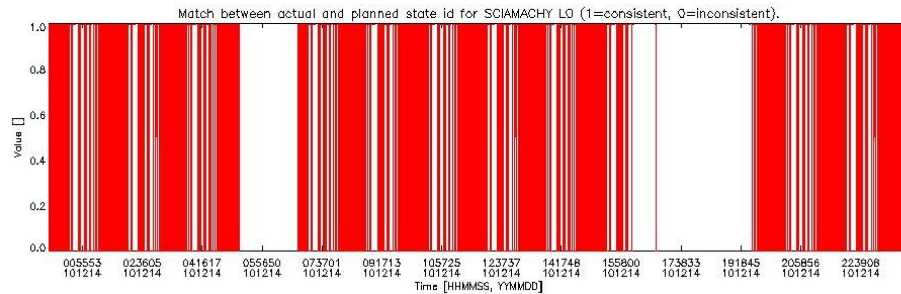
sciamachy_daily_report_level0_KSPT_L0_4504_N_20101214_5.PNG
