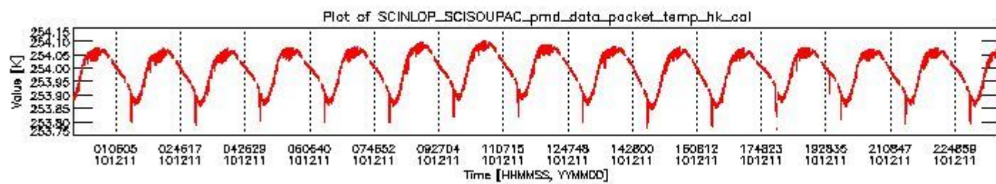
sciamachy_daily_report_level0_KSPT_L0_4504_N_20101211_3.PNG
