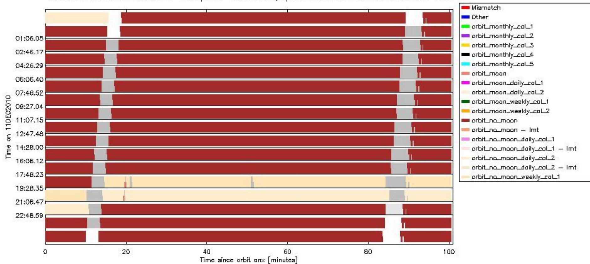
sciamachy_daily_report_level0_KSPT_L0_4504_N_20101211_6.PNG
