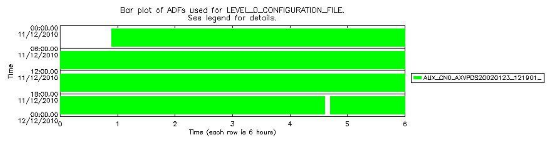
sciamachy_daily_report_level0_KSPT_L0_4504_N_20101211_7.PNG
