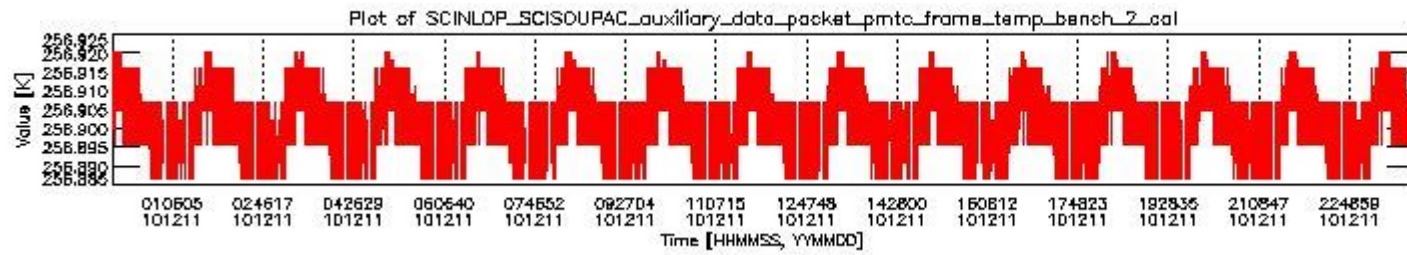
sciamachy_daily_report_level0_KSPT_L0_4504_N_20101211_1.PNG
