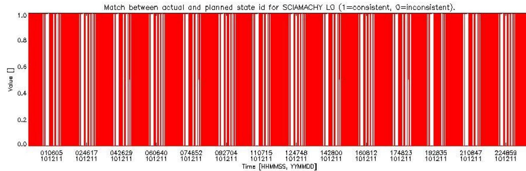
sciamachy_daily_report_level0_KSPT_L0_4504_N_20101211_5.PNG
