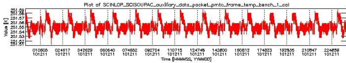
sciamachy_daily_report_level0_KSPT_L0_4504_N_20101211_0.PNG
