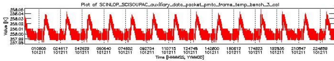
sciamachy_daily_report_level0_KSPT_L0_4504_N_20101211_2.PNG
