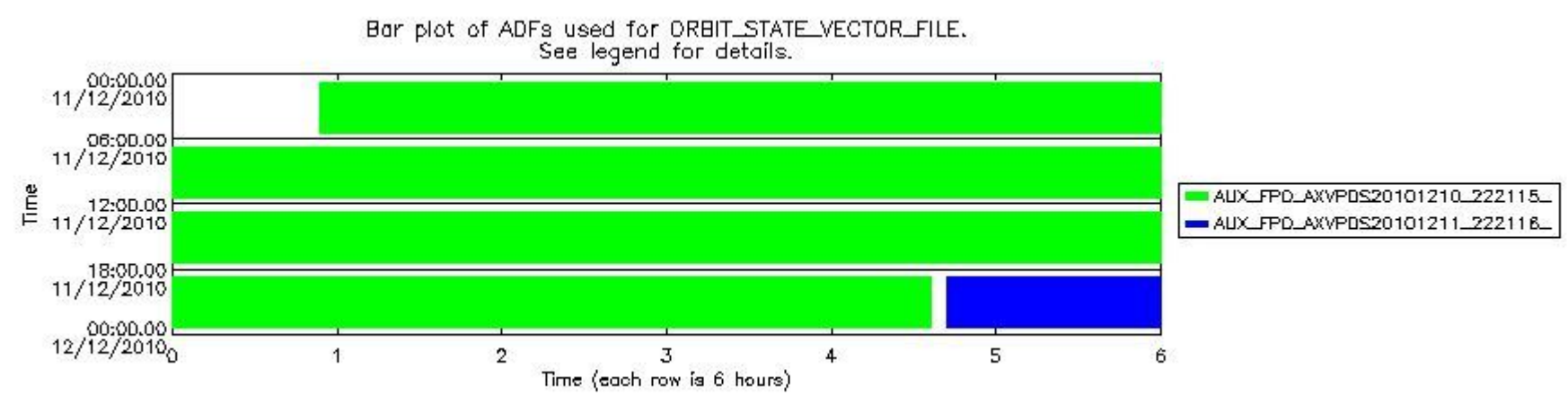
sciamachy_daily_report_level0_KSPT_L0_4504_N_20101211_8.PNG
