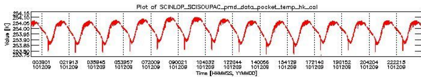
sciamachy_daily_report_level0_KSPT_L0_4504_N_20101209_3.PNG
