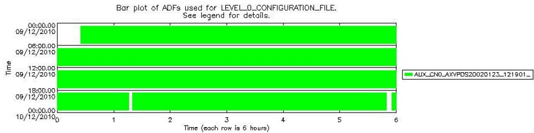
sciamachy_daily_report_level0_KSPT_L0_4504_N_20101209_7.PNG
