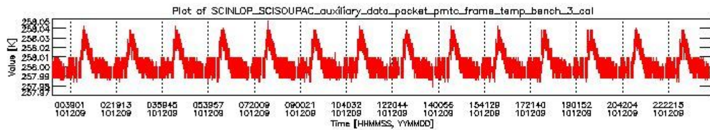
sciamachy_daily_report_level0_KSPT_L0_4504_N_20101209_2.PNG
