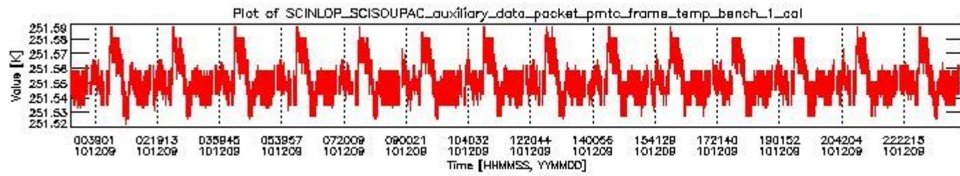
sciamachy_daily_report_level0_KSPT_L0_4504_N_20101209_0.PNG
