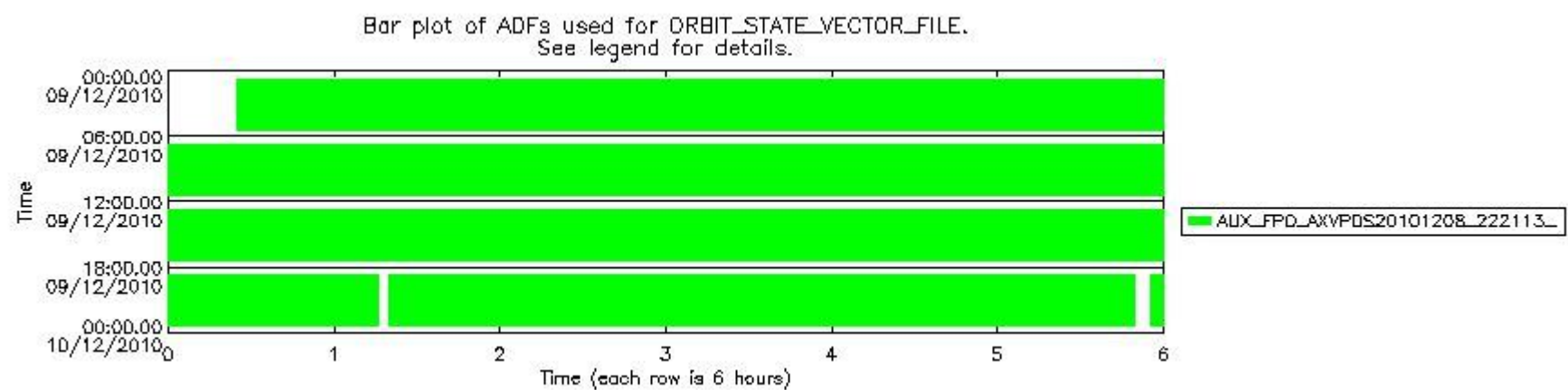
sciamachy_daily_report_level0_KSPT_L0_4504_N_20101209_8.PNG
