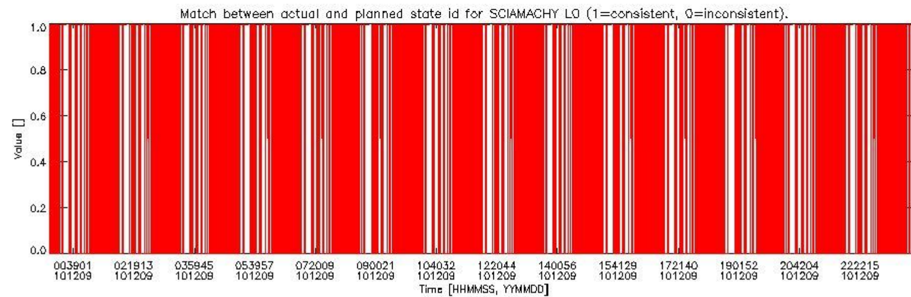
sciamachy_daily_report_level0_KSPT_L0_4504_N_20101209_5.PNG
