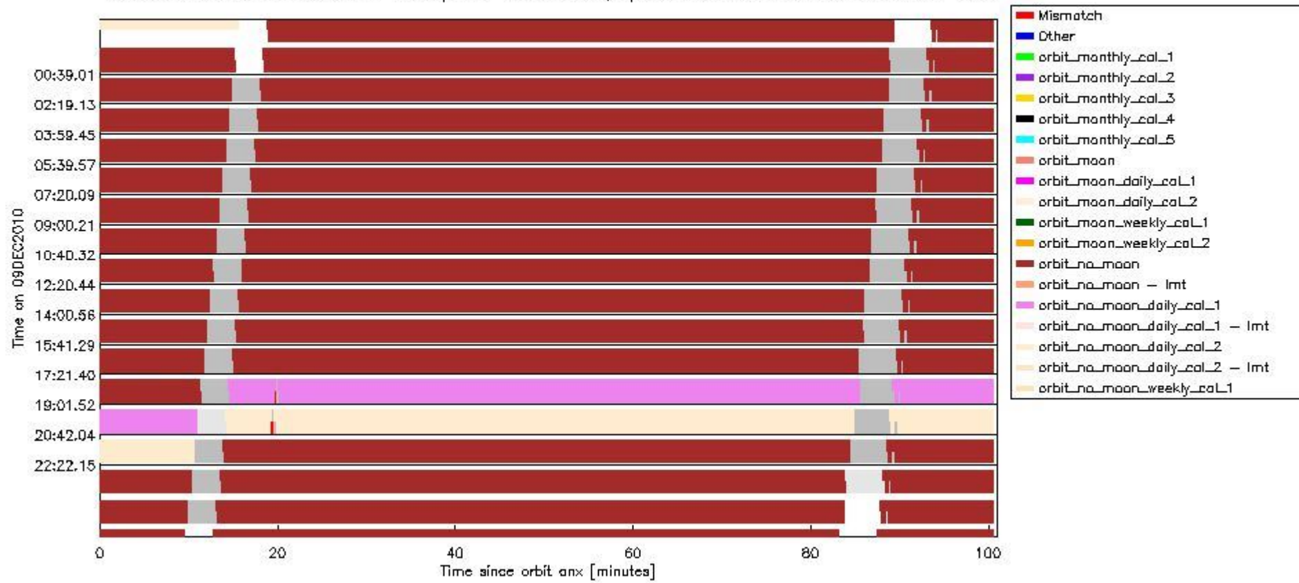
sciamachy_daily_report_level0_KSPT_L0_4504_N_20101209_6.PNG
