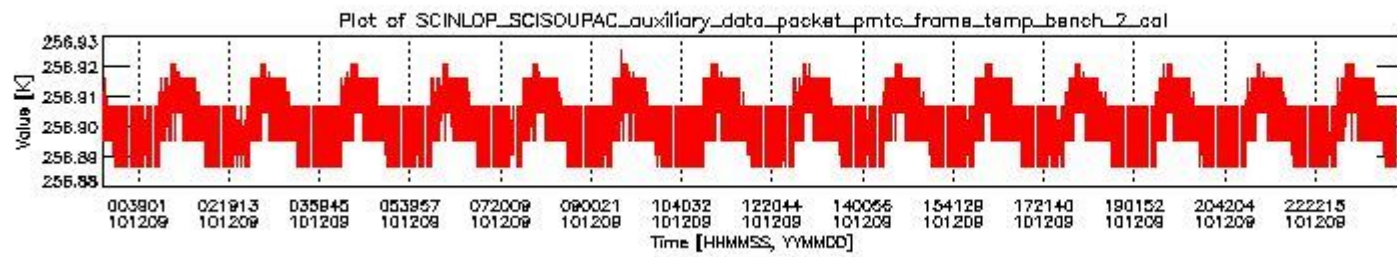
sciamachy_daily_report_level0_KSPT_L0_4504_N_20101209_1.PNG
