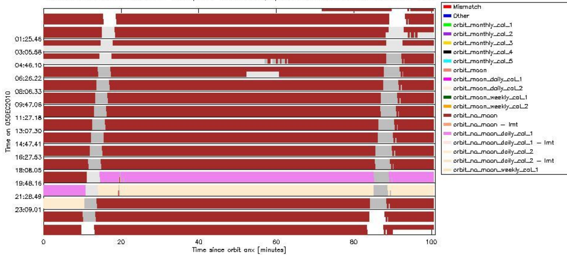
sciamachy_daily_report_level0_KSPT_L0_4504_N_20101205_6.PNG
