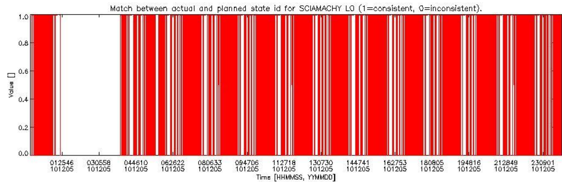
sciamachy_daily_report_level0_KSPT_L0_4504_N_20101205_5.PNG
