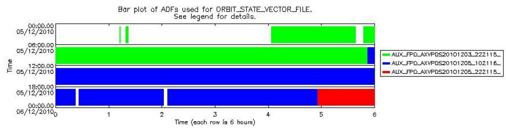
sciamachy_daily_report_level0_KSPT_L0_4504_N_20101205_8.PNG
