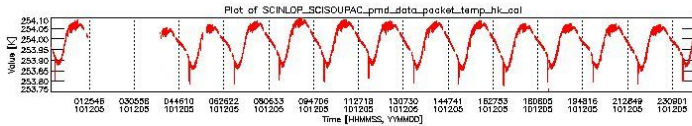
sciamachy_daily_report_level0_KSPT_L0_4504_N_20101205_3.PNG
