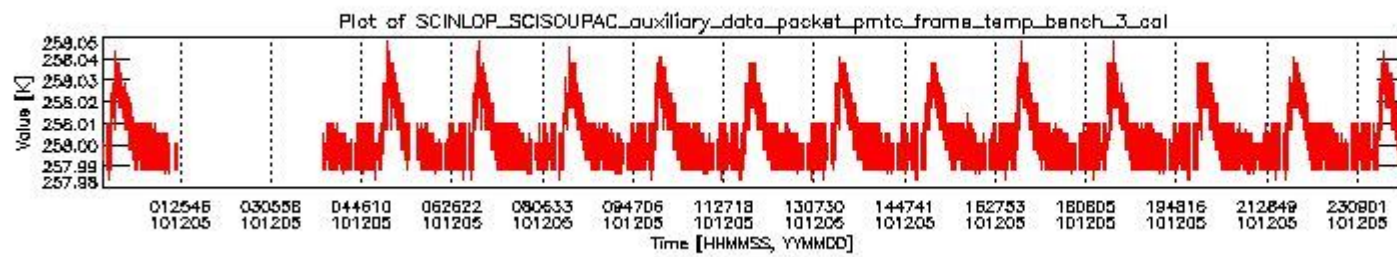
sciamachy_daily_report_level0_KSPT_L0_4504_N_20101205_2.PNG
