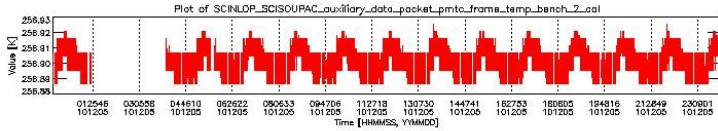
sciamachy_daily_report_level0_KSPT_L0_4504_N_20101205_1.PNG
