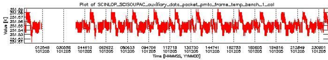
sciamachy_daily_report_level0_KSPT_L0_4504_N_20101205_0.PNG
