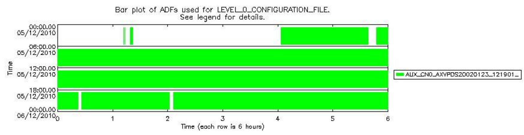
sciamachy_daily_report_level0_KSPT_L0_4504_N_20101205_7.PNG
