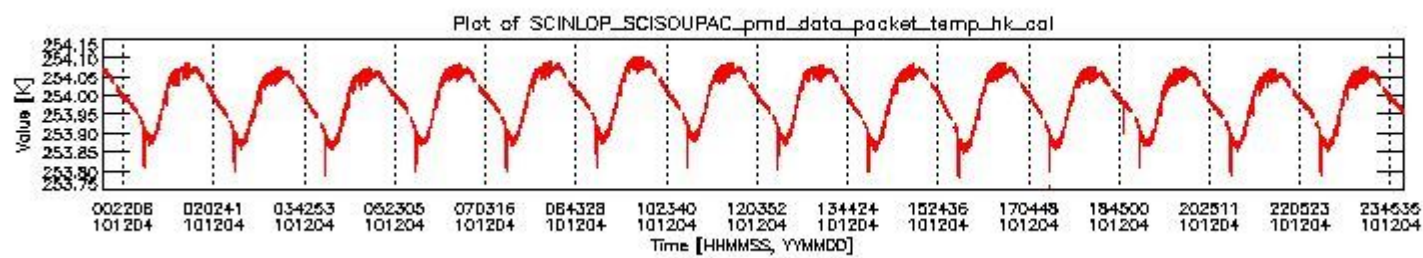
sciamachy_daily_report_level0_KSPT_L0_4504_N_20101204_3.PNG
