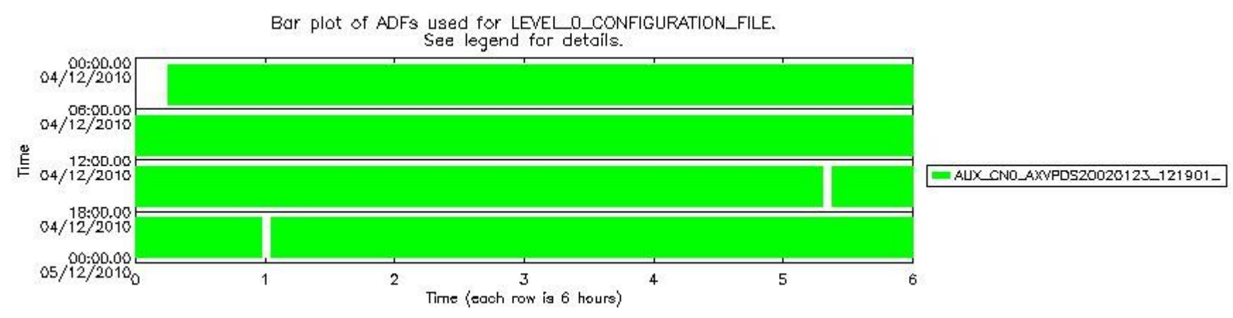
sciamachy_daily_report_level0_KSPT_L0_4504_N_20101204_7.PNG
