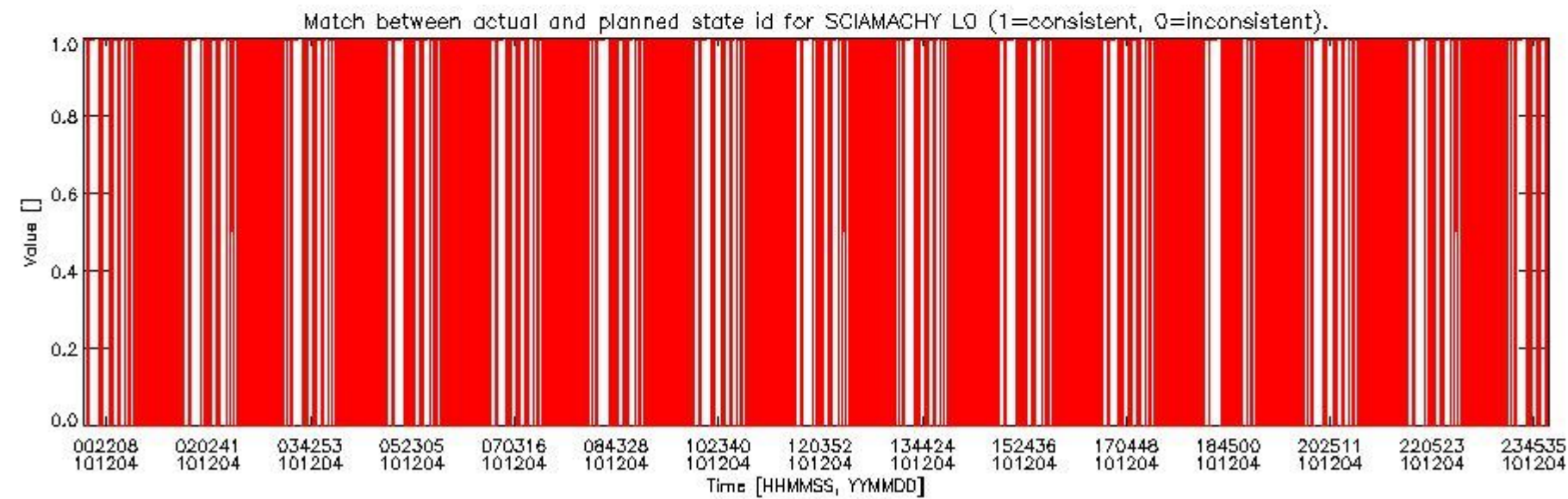
sciamachy_daily_report_level0_KSPT_L0_4504_N_20101204_5.PNG
