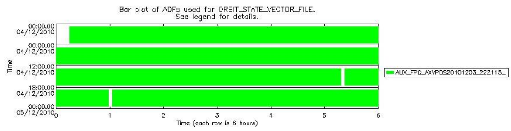
sciamachy_daily_report_level0_KSPT_L0_4504_N_20101204_8.PNG
