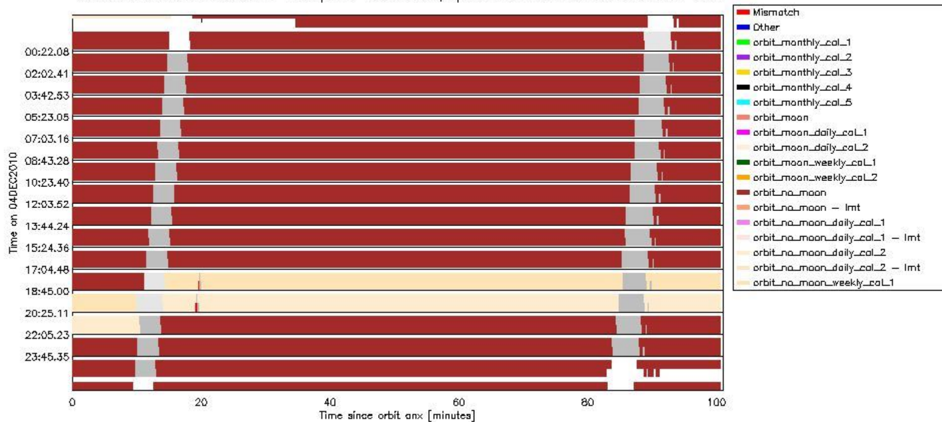
sciamachy_daily_report_level0_KSPT_L0_4504_N_20101204_6.PNG
