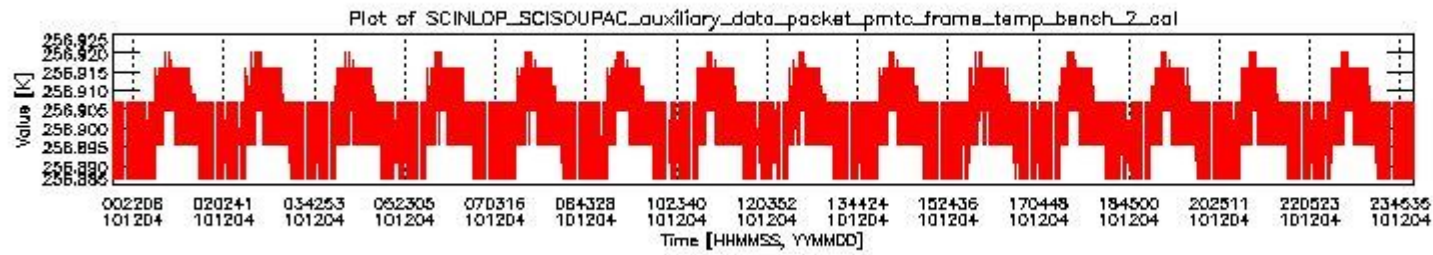
sciamachy_daily_report_level0_KSPT_L0_4504_N_20101204_1.PNG
