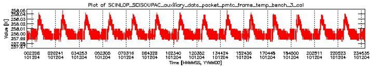
sciamachy_daily_report_level0_KSPT_L0_4504_N_20101204_2.PNG
