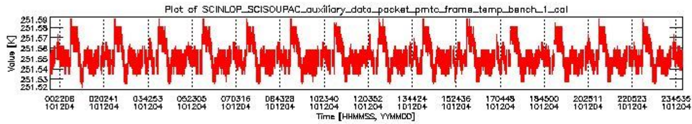
sciamachy_daily_report_level0_KSPT_L0_4504_N_20101204_0.PNG
