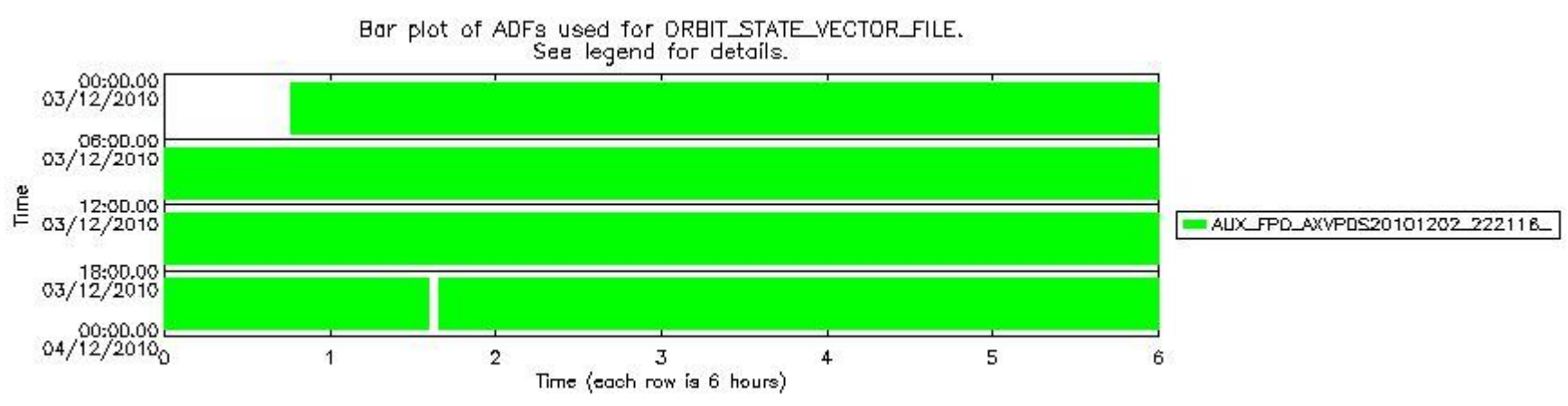
sciamachy_daily_report_level0_KSPT_L0_4504_N_20101203_8.PNG
