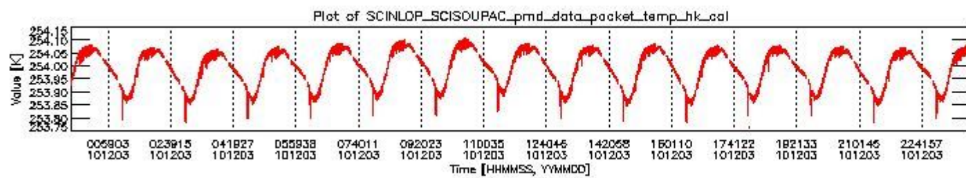
sciamachy_daily_report_level0_KSPT_L0_4504_N_20101203_3.PNG
