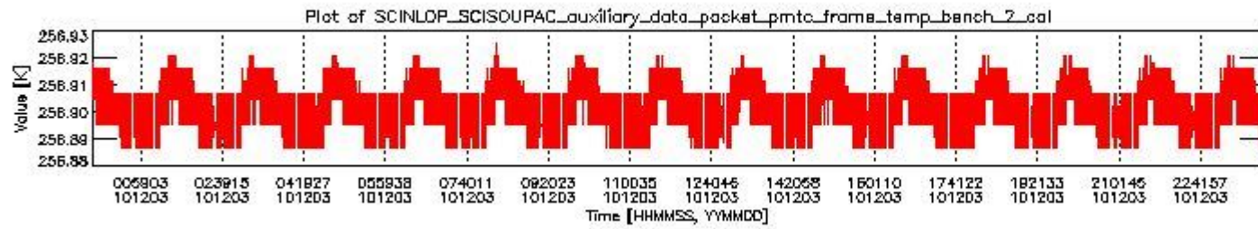
sciamachy_daily_report_level0_KSPT_L0_4504_N_20101203_1.PNG
