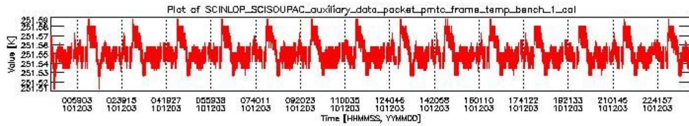
sciamachy_daily_report_level0_KSPT_L0_4504_N_20101203_0.PNG
