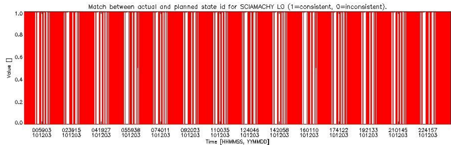
sciamachy_daily_report_level0_KSPT_L0_4504_N_20101203_5.PNG
