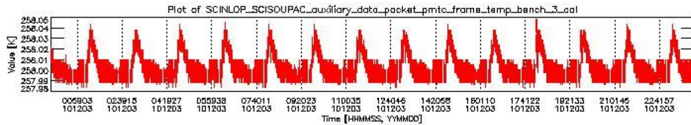
sciamachy_daily_report_level0_KSPT_L0_4504_N_20101203_2.PNG
