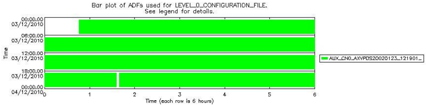
sciamachy_daily_report_level0_KSPT_L0_4504_N_20101203_7.PNG
