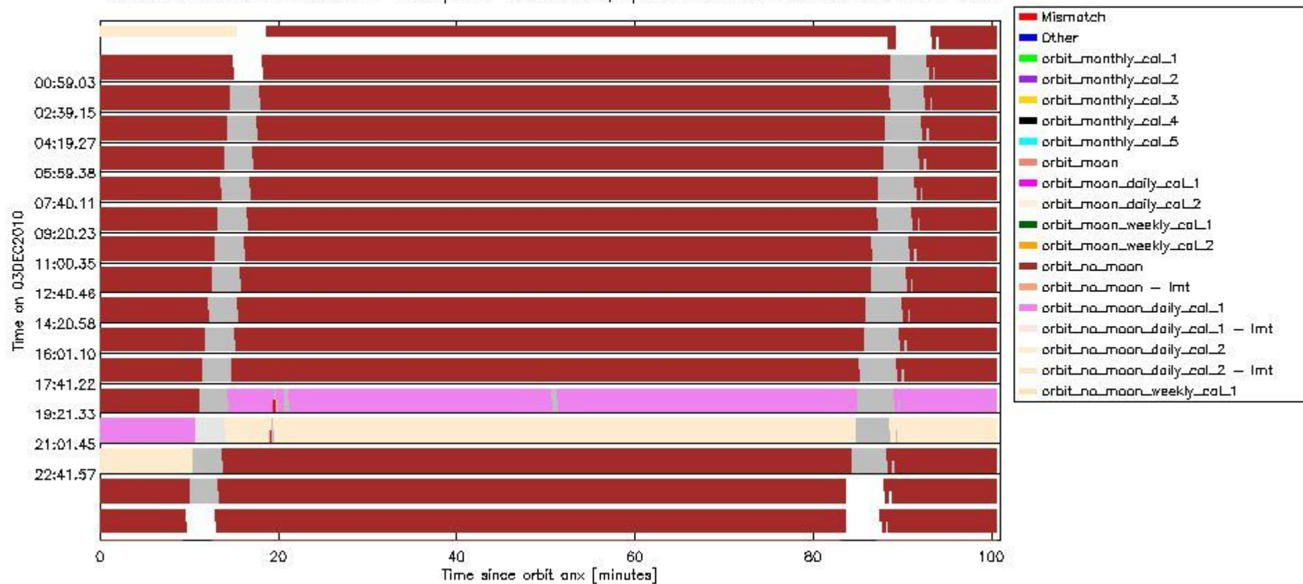
sciamachy_daily_report_level0_KSPT_L0_4504_N_20101203_6.PNG
