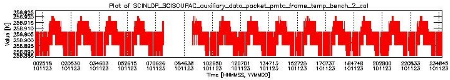
sciamachy_daily_report_level0_KSPT_L0_4504_N_20101123_1.PNG
