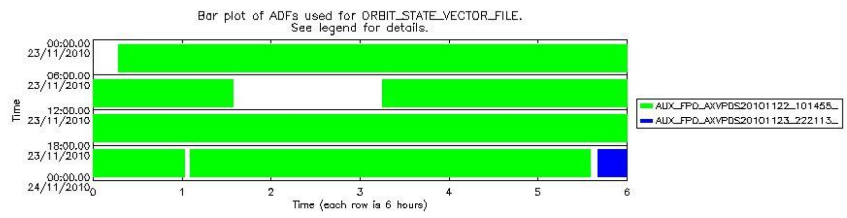
sciamachy_daily_report_level0_KSPT_L0_4504_N_20101123_8.PNG
