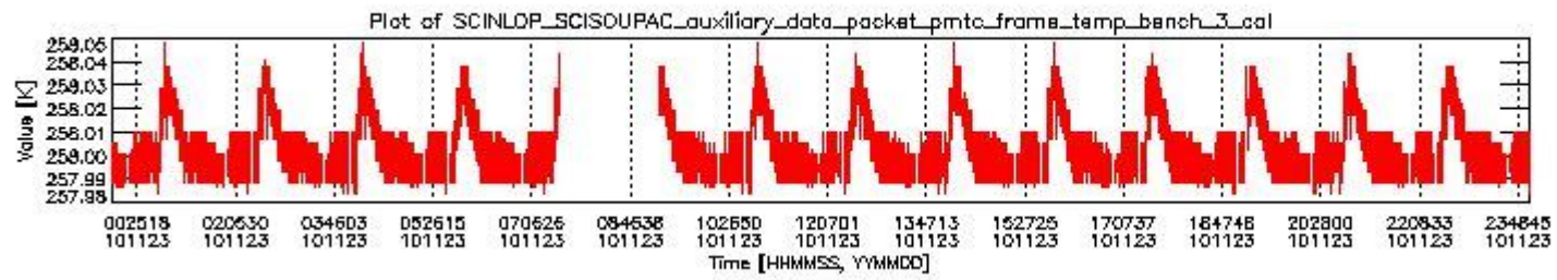
sciamachy_daily_report_level0_KSPT_L0_4504_N_20101123_2.PNG
