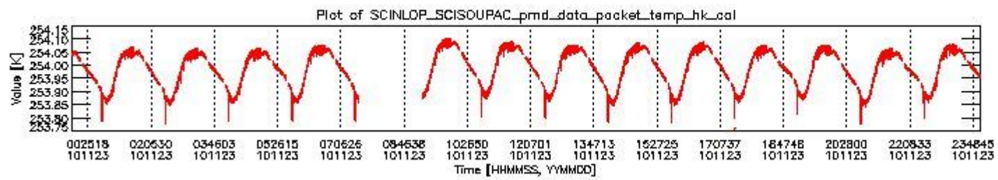
sciamachy_daily_report_level0_KSPT_L0_4504_N_20101123_3.PNG
