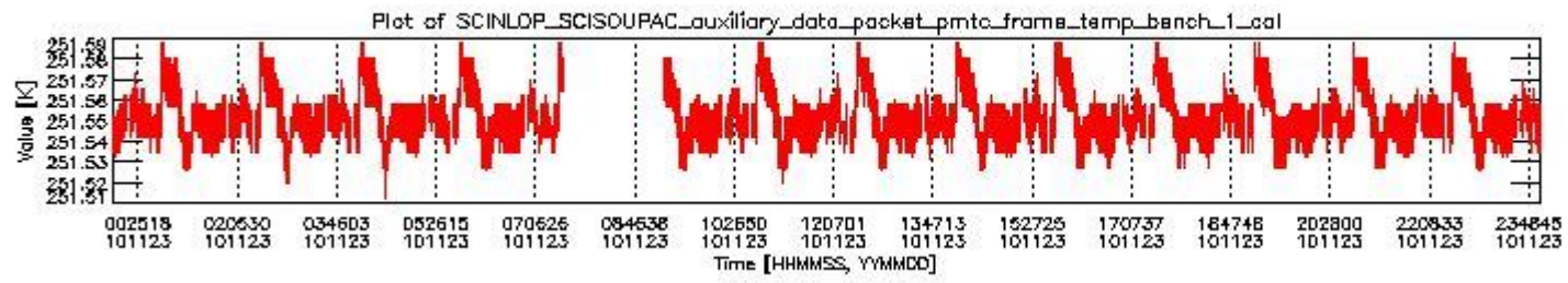
sciamachy_daily_report_level0_KSPT_L0_4504_N_20101123_0.PNG
