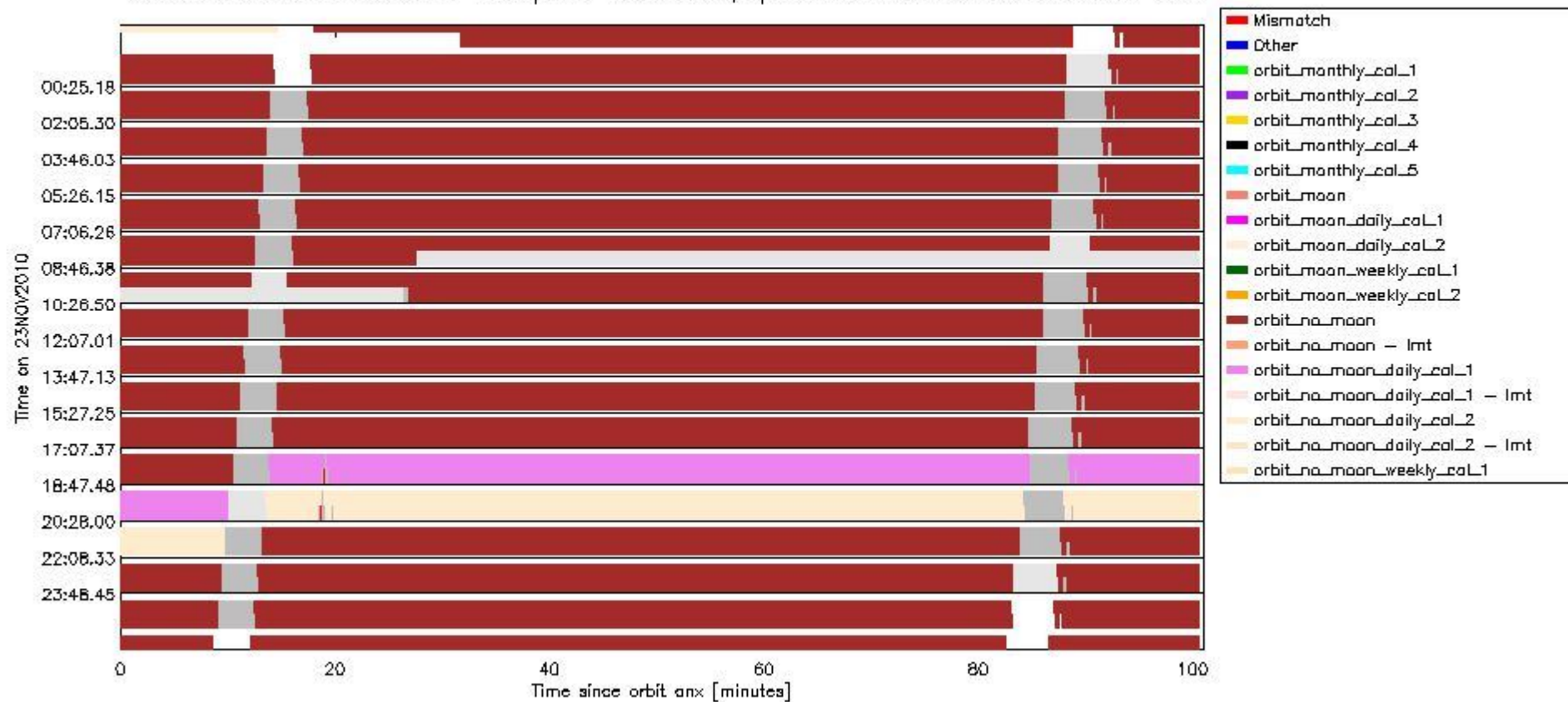
sciamachy_daily_report_level0_KSPT_L0_4504_N_20101123_6.PNG
