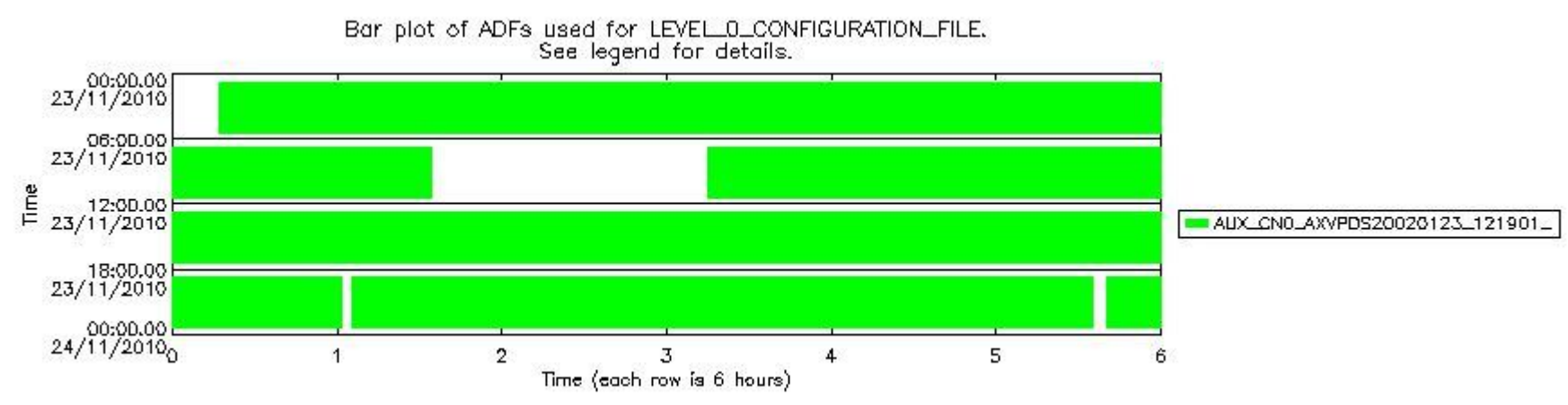
sciamachy_daily_report_level0_KSPT_L0_4504_N_20101123_7.PNG
