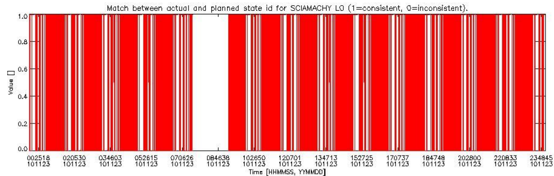
sciamachy_daily_report_level0_KSPT_L0_4504_N_20101123_5.PNG
