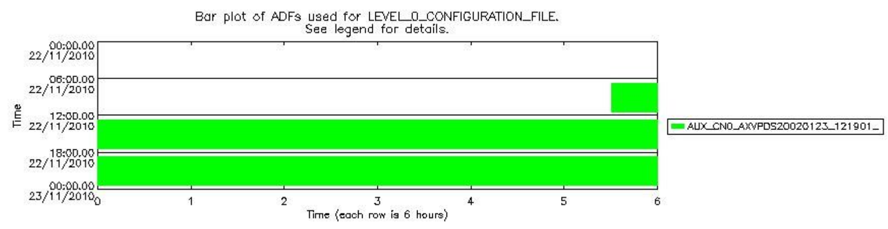
sciamachy_daily_report_level0_KSPT_L0_4504_N_20101122_7.PNG
