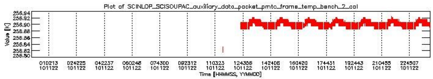
sciamachy_daily_report_level0_KSPT_L0_4504_N_20101122_1.PNG
