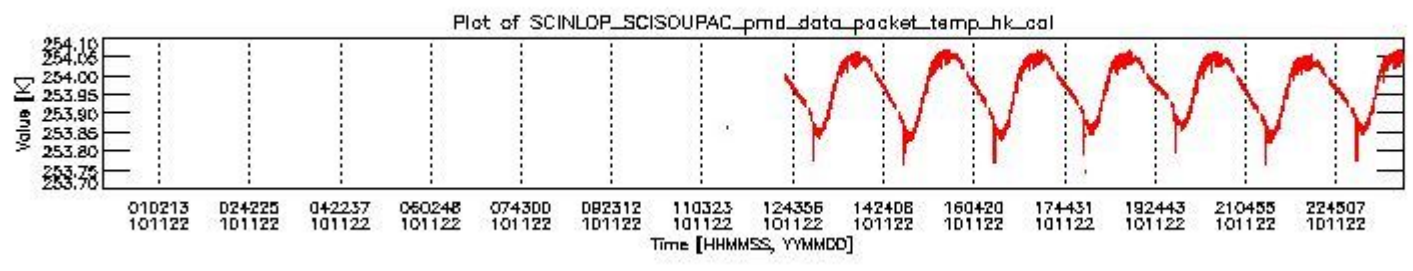
sciamachy_daily_report_level0_KSPT_L0_4504_N_20101122_3.PNG
