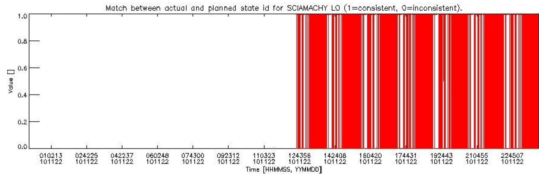
sciamachy_daily_report_level0_KSPT_L0_4504_N_20101122_5.PNG
