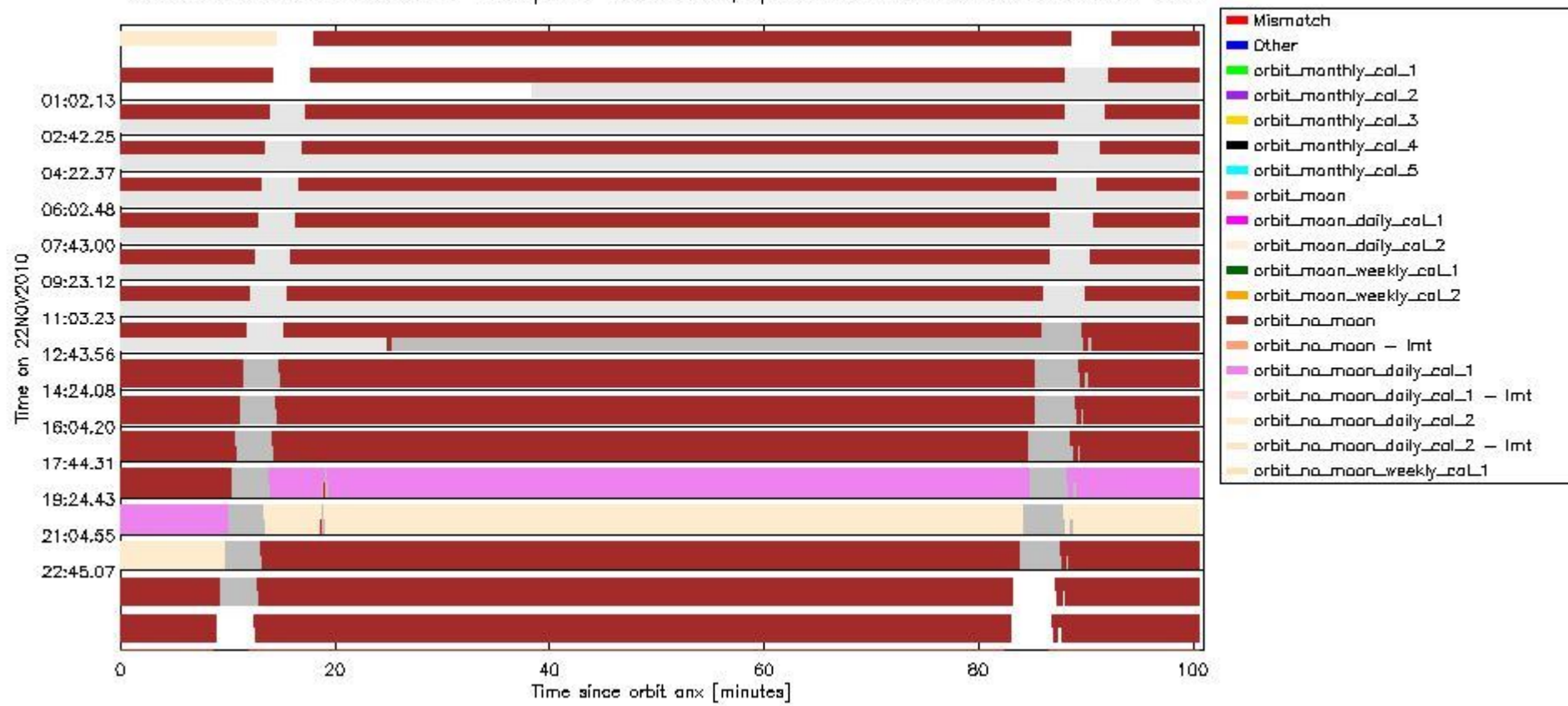
sciamachy_daily_report_level0_KSPT_L0_4504_N_20101122_6.PNG
