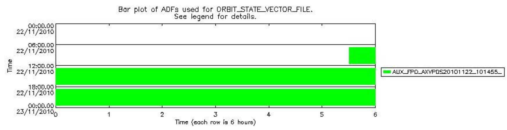
sciamachy_daily_report_level0_KSPT_L0_4504_N_20101122_8.PNG
