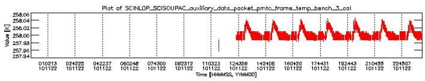
sciamachy_daily_report_level0_KSPT_L0_4504_N_20101122_2.PNG
