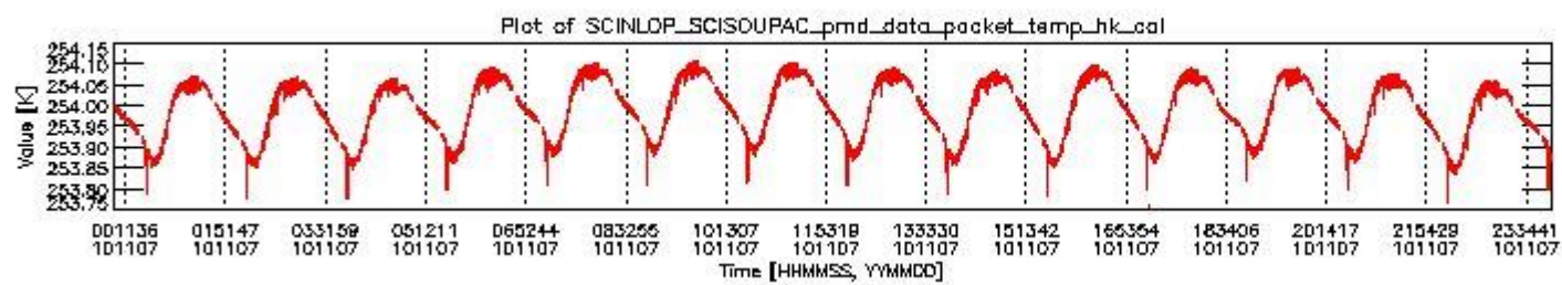
sciamachy_daily_report_level0_KSPT_L0_4504_N_20101107_3.PNG
