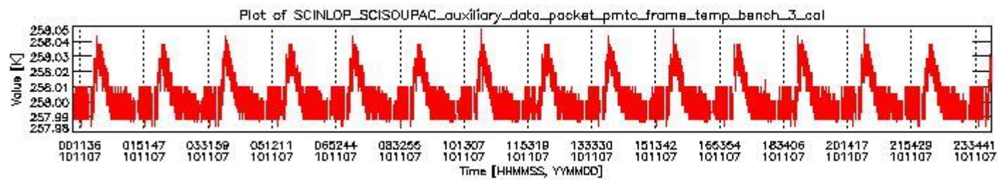
sciamachy_daily_report_level0_KSPT_L0_4504_N_20101107_2.PNG
