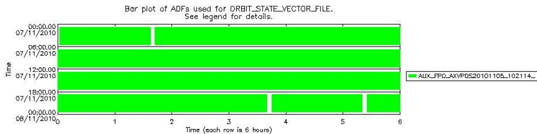
sciamachy_daily_report_level0_KSPT_L0_4504_N_20101107_8.PNG
