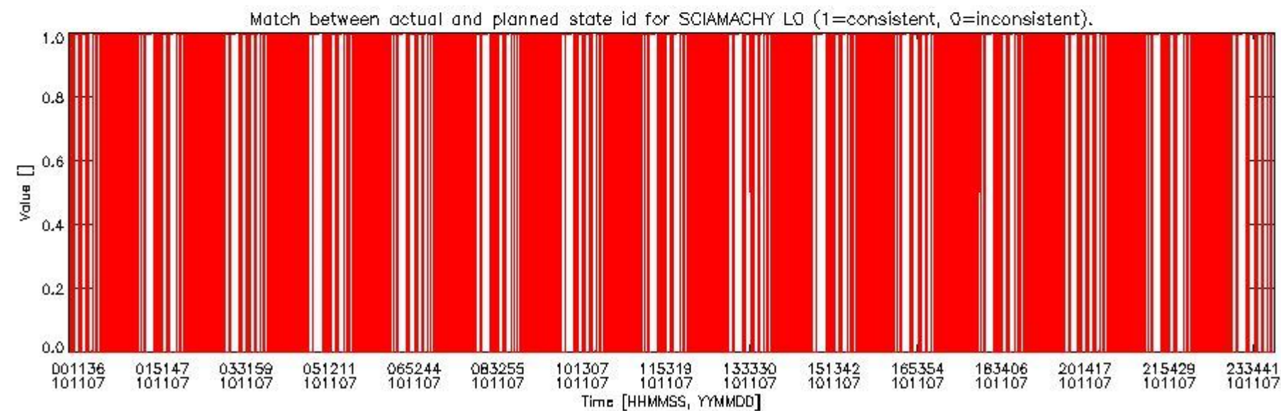
sciamachy_daily_report_level0_KSPT_L0_4504_N_20101107_5.PNG
