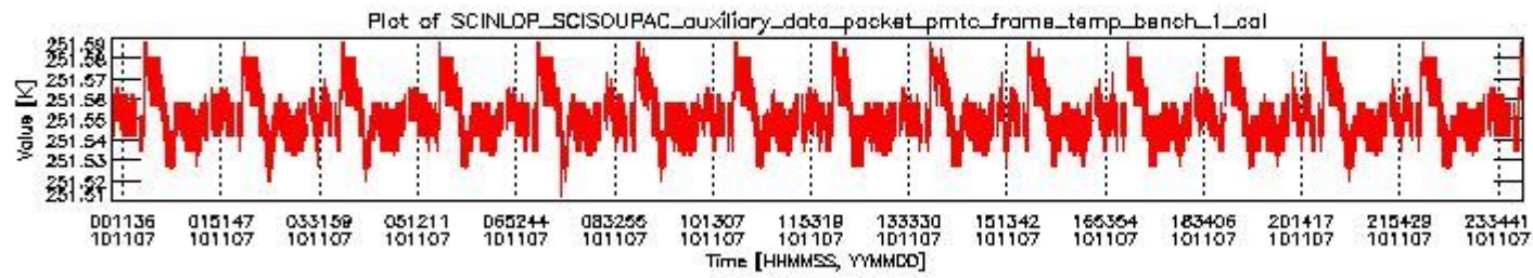
sciamachy_daily_report_level0_KSPT_L0_4504_N_20101107_0.PNG
