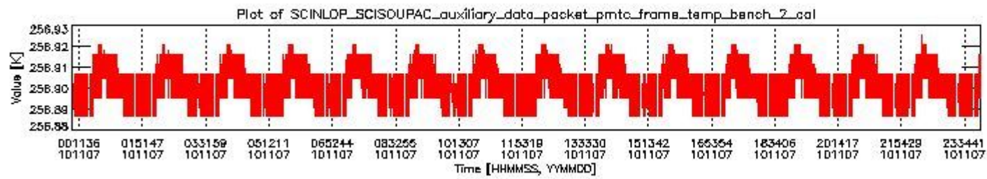
sciamachy_daily_report_level0_KSPT_L0_4504_N_20101107_1.PNG
