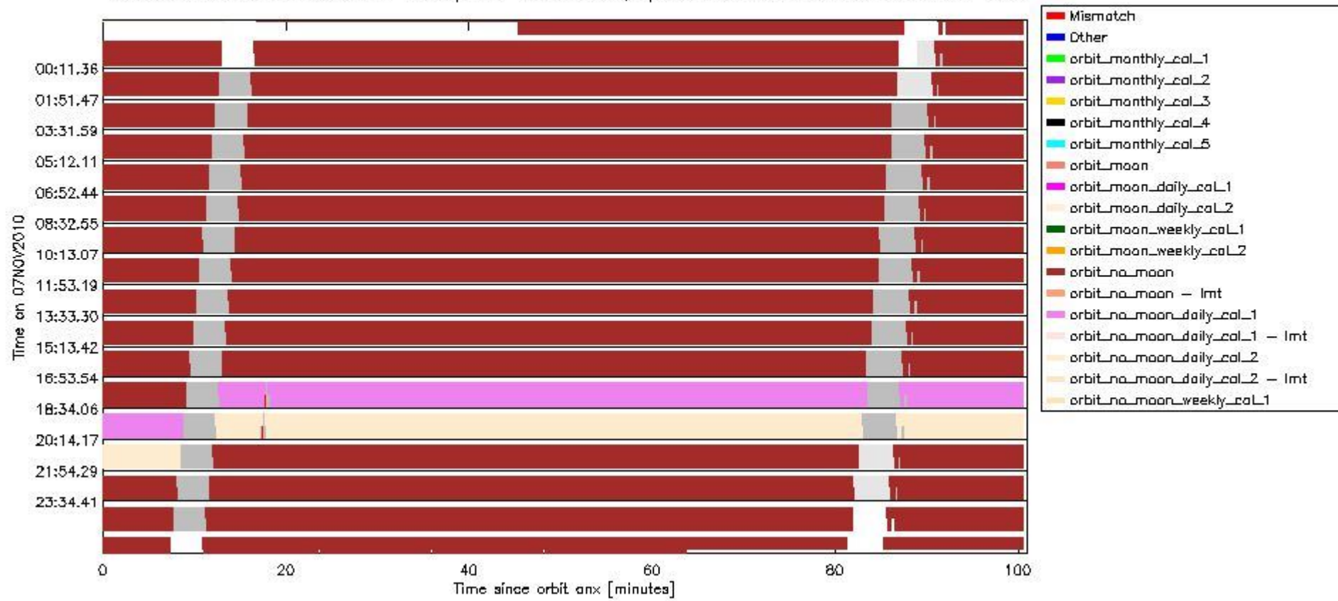
sciamachy_daily_report_level0_KSPT_L0_4504_N_20101107_6.PNG
