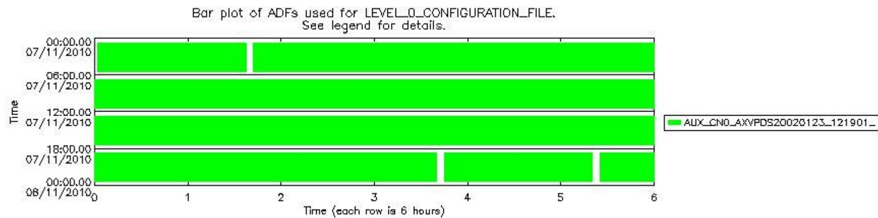
sciamachy_daily_report_level0_KSPT_L0_4504_N_20101107_7.PNG
