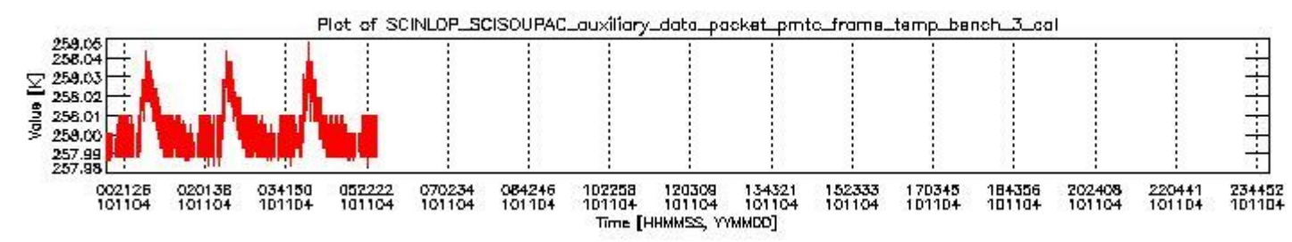
sciamachy_daily_report_level0_KSPT_L0_4504_N_20101104_2.PNG
