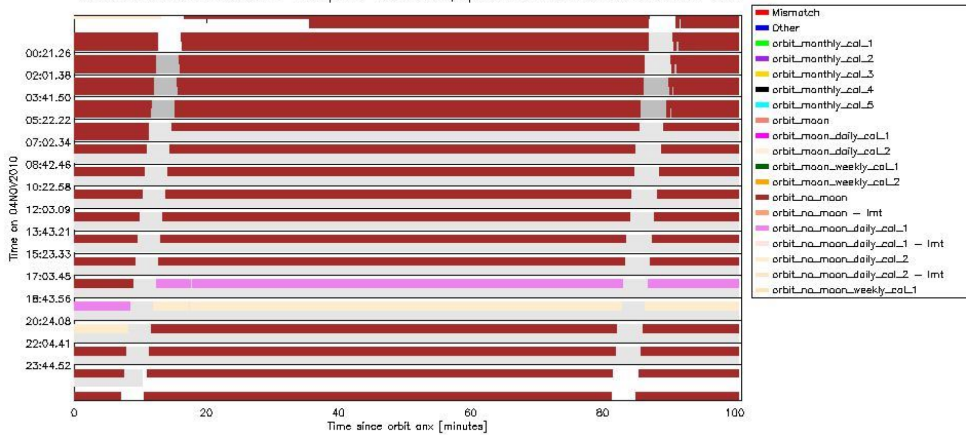
sciamachy_daily_report_level0_KSPT_L0_4504_N_20101104_6.PNG
