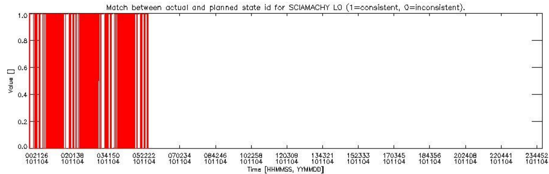
sciamachy_daily_report_level0_KSPT_L0_4504_N_20101104_5.PNG
