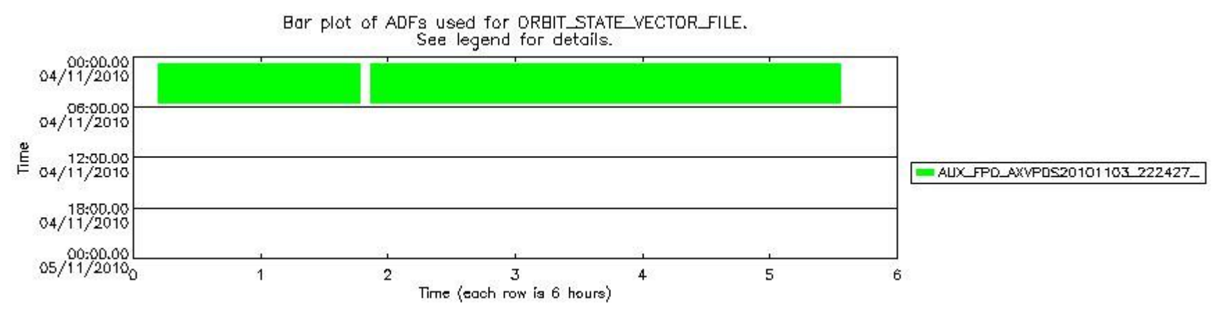
sciamachy_daily_report_level0_KSPT_L0_4504_N_20101104_8.PNG
