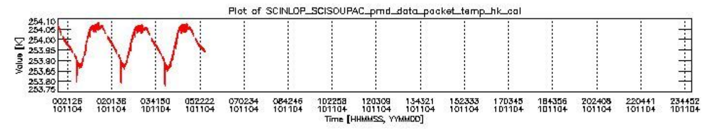
sciamachy_daily_report_level0_KSPT_L0_4504_N_20101104_3.PNG
