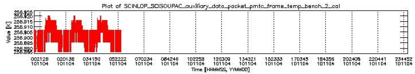
sciamachy_daily_report_level0_KSPT_L0_4504_N_20101104_1.PNG
