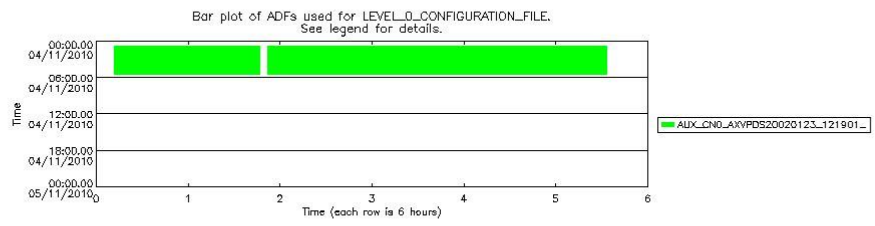
sciamachy_daily_report_level0_KSPT_L0_4504_N_20101104_7.PNG
