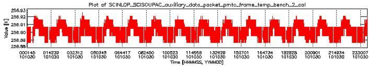
sciamachy_daily_report_level0_KSPT_L0_4504_N_20101030_1.PNG
