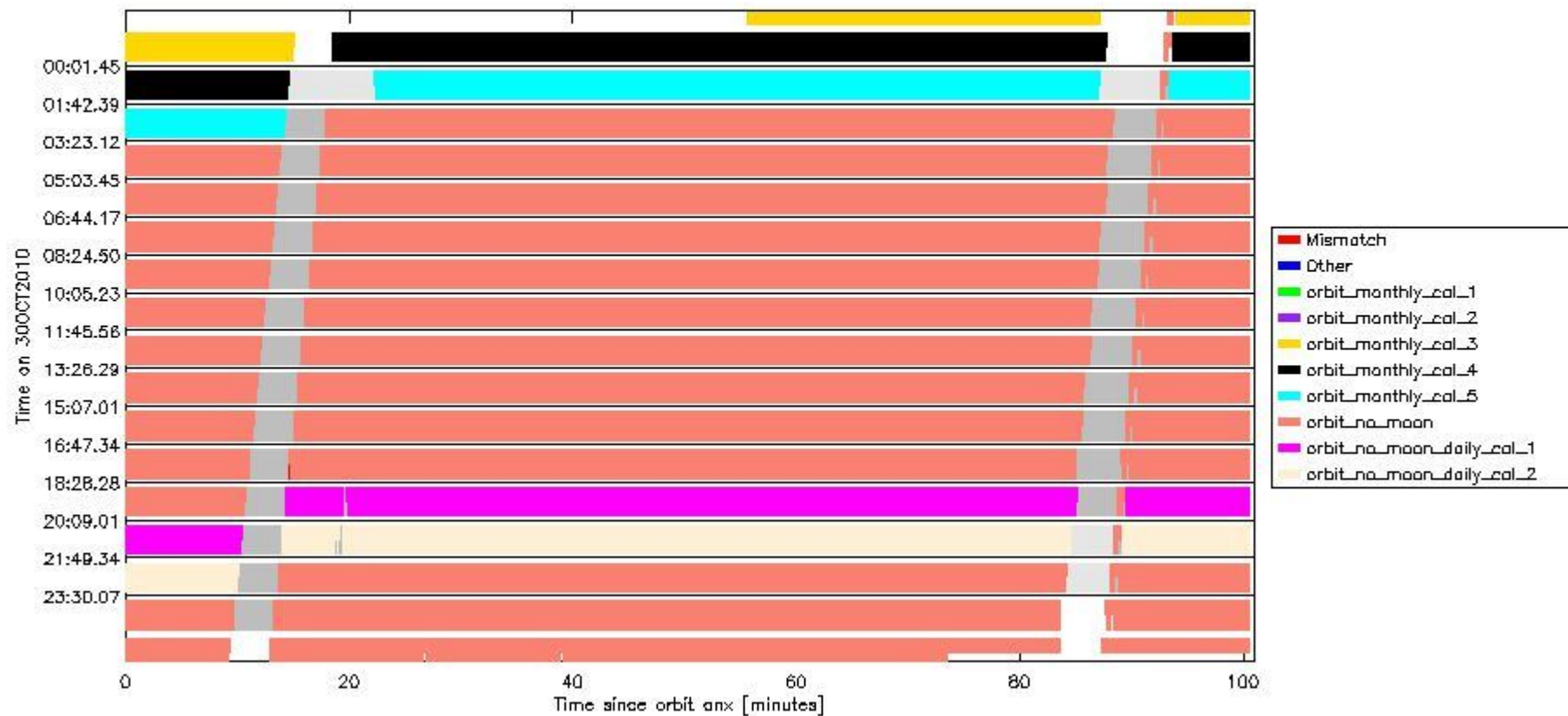
sciamachy_daily_report_level0_KSPT_L0_4504_N_20101030_6.PNG
