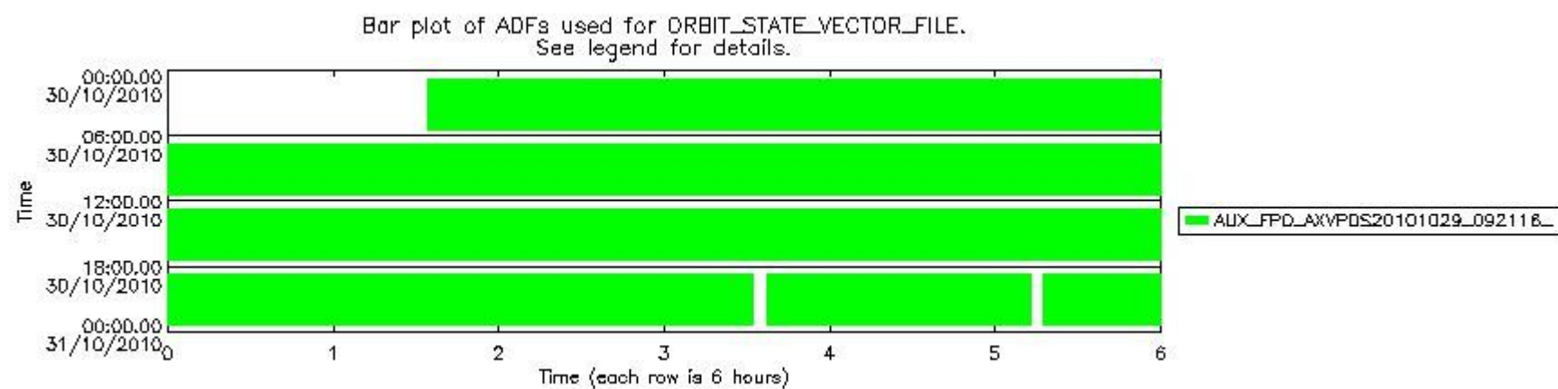
sciamachy_daily_report_level0_KSPT_L0_4504_N_20101030_8.PNG
