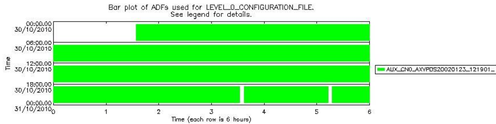
sciamachy_daily_report_level0_KSPT_L0_4504_N_20101030_7.PNG
