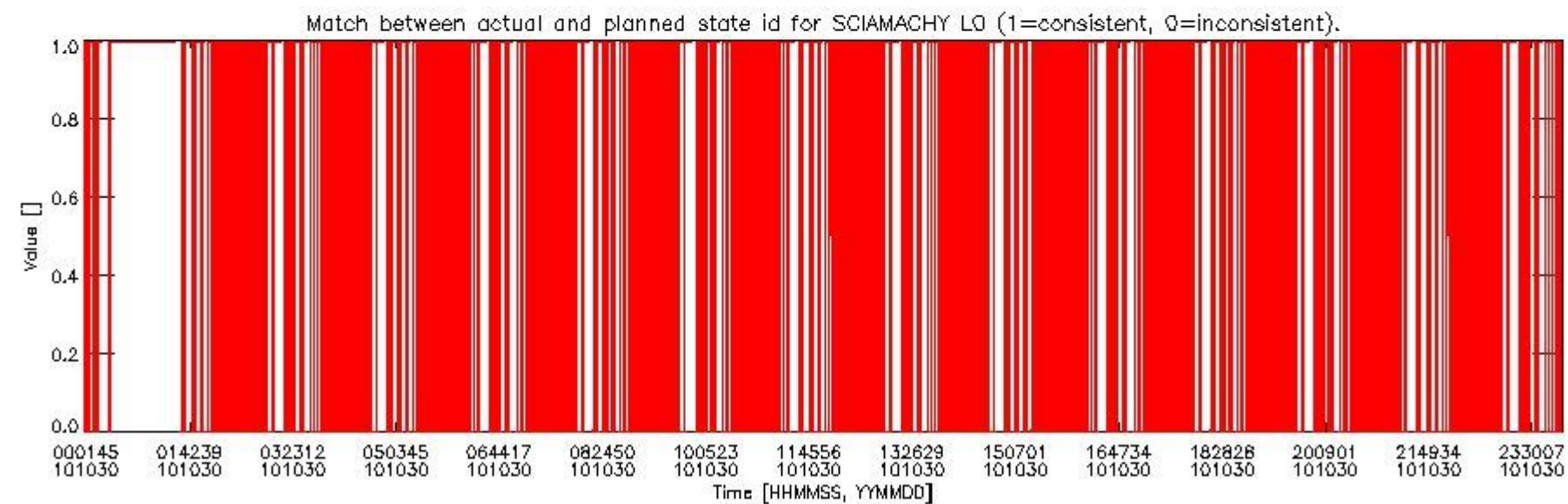
sciamachy_daily_report_level0_KSPT_L0_4504_N_20101030_5.PNG
