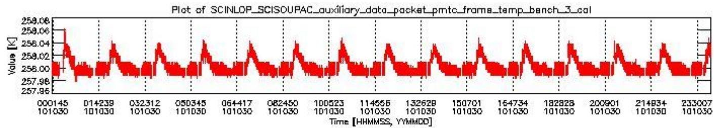
sciamachy_daily_report_level0_KSPT_L0_4504_N_20101030_2.PNG
