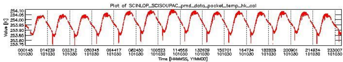
sciamachy_daily_report_level0_KSPT_L0_4504_N_20101030_3.PNG
