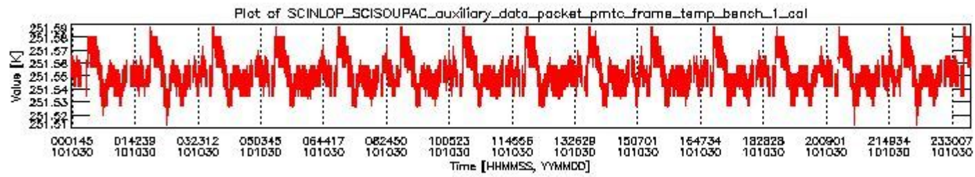
sciamachy_daily_report_level0_KSPT_L0_4504_N_20101030_0.PNG
