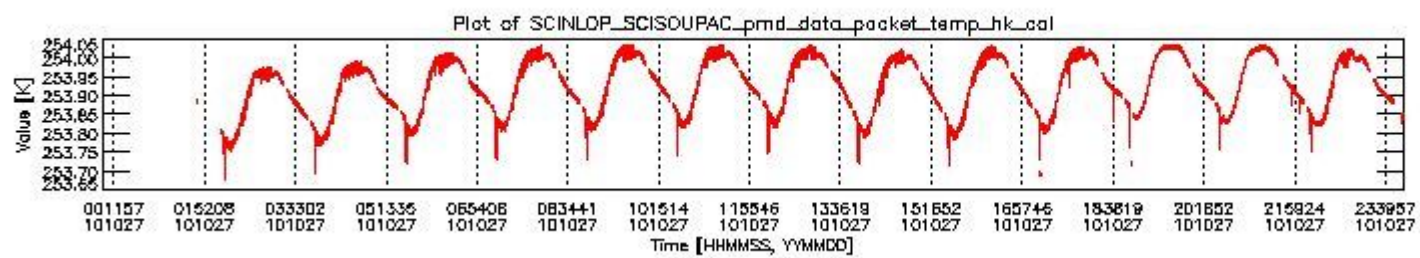
sciamachy_daily_report_level0_KSPT_L0_4504_N_20101027_3.PNG
