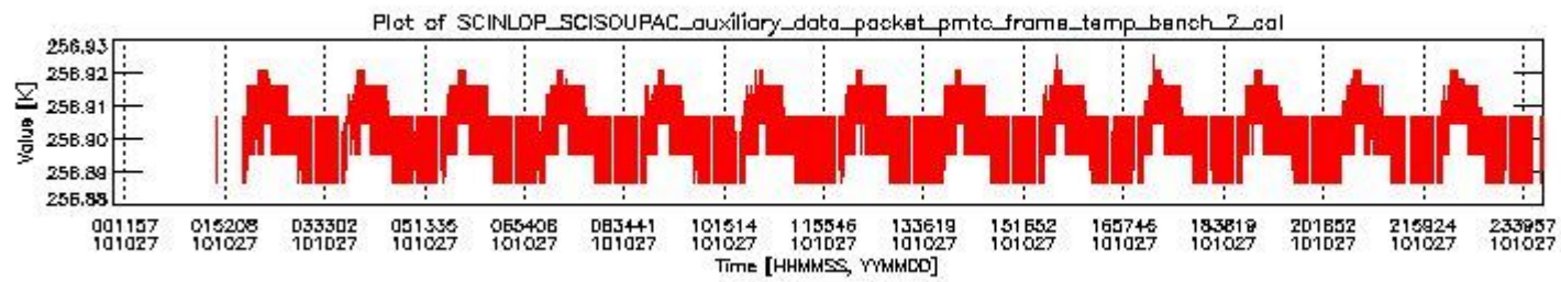
sciamachy_daily_report_level0_KSPT_L0_4504_N_20101027_1.PNG
