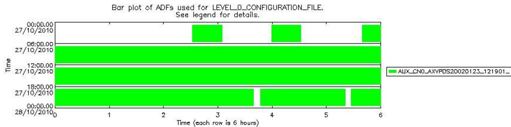
sciamachy_daily_report_level0_KSPT_L0_4504_N_20101027_7.PNG
