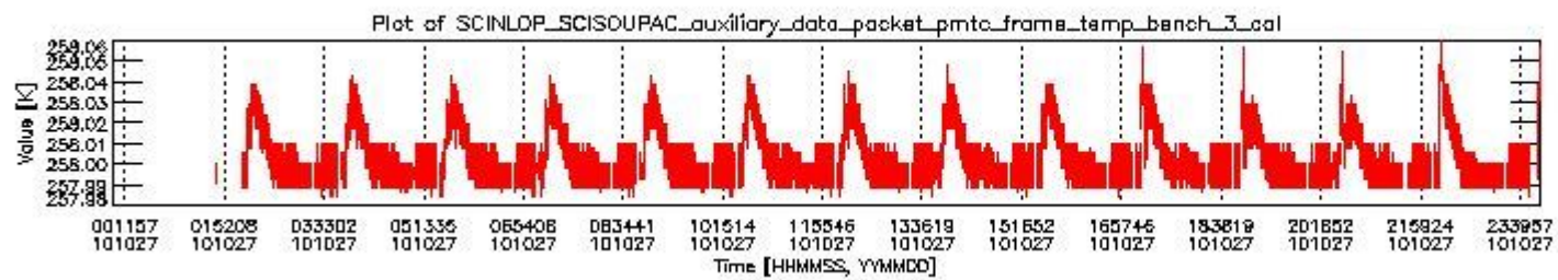
sciamachy_daily_report_level0_KSPT_L0_4504_N_20101027_2.PNG
