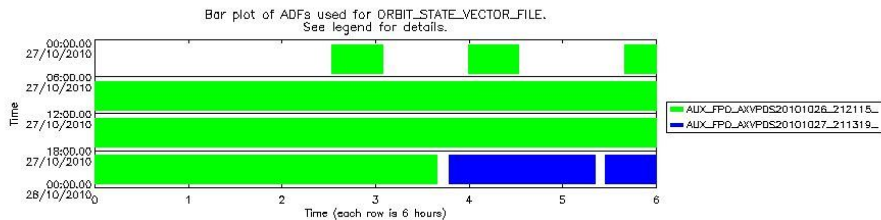
sciamachy_daily_report_level0_KSPT_L0_4504_N_20101027_8.PNG
