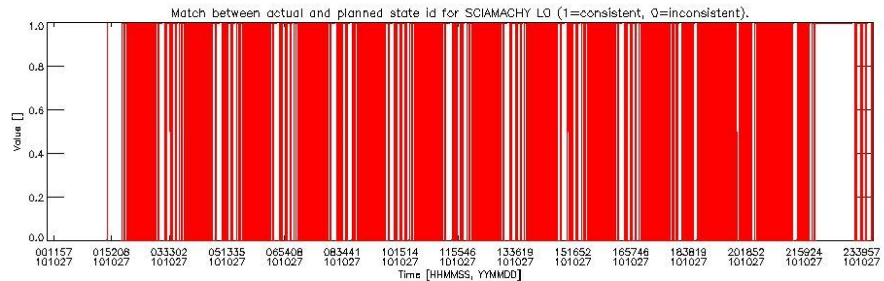
sciamachy_daily_report_level0_KSPT_L0_4504_N_20101027_5.PNG
