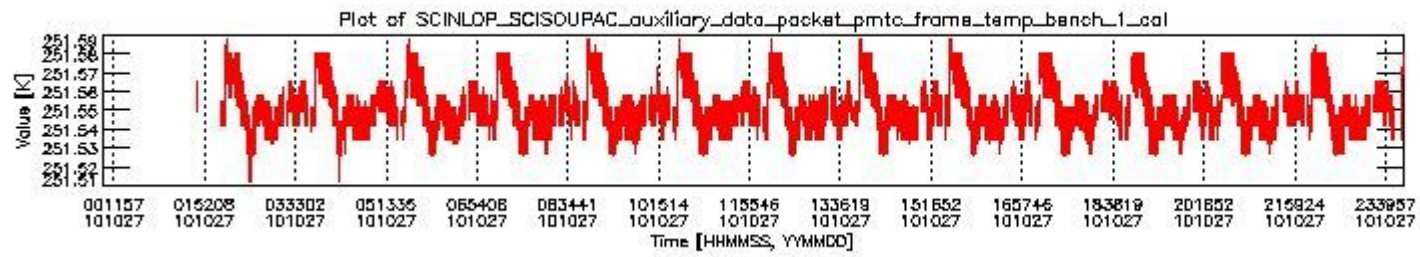
sciamachy_daily_report_level0_KSPT_L0_4504_N_20101027_0.PNG
