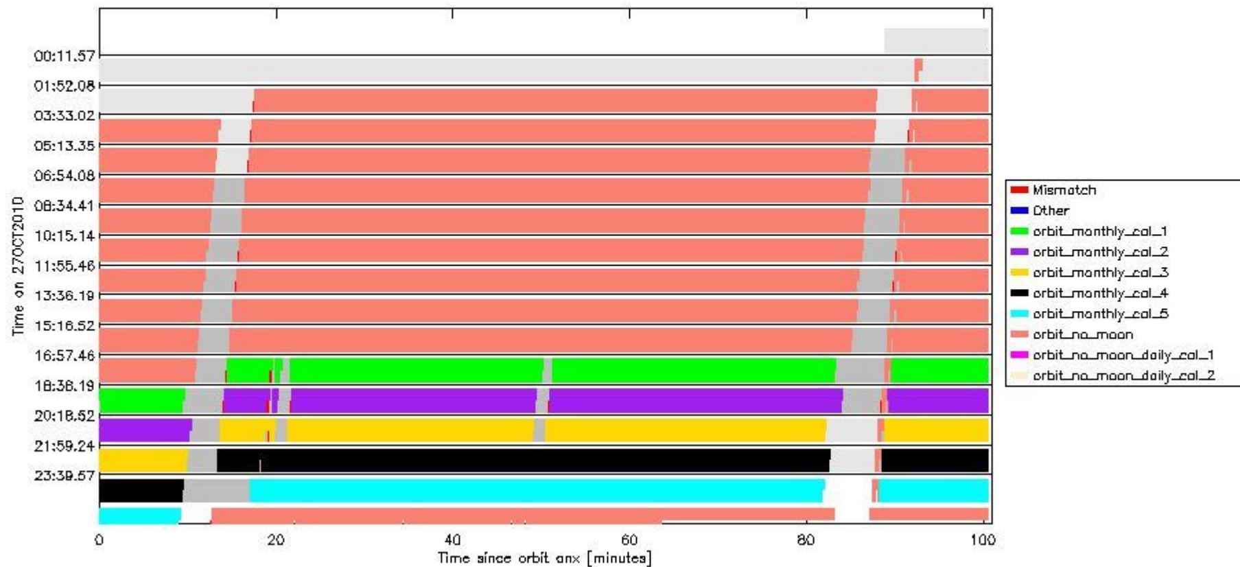
sciamachy_daily_report_level0_KSPT_L0_4504_N_20101027_6.PNG
