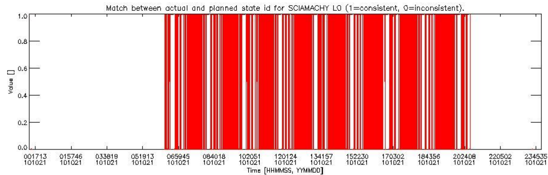
sciamachy_daily_report_level0_KSPT_L0_4504_N_20101021_5.PNG
