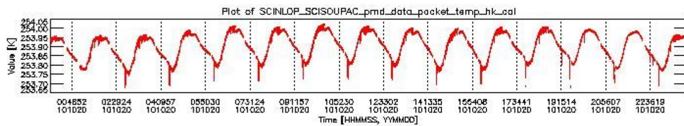
sciamachy_daily_report_level0_Any_version_20101020_3.PNG
