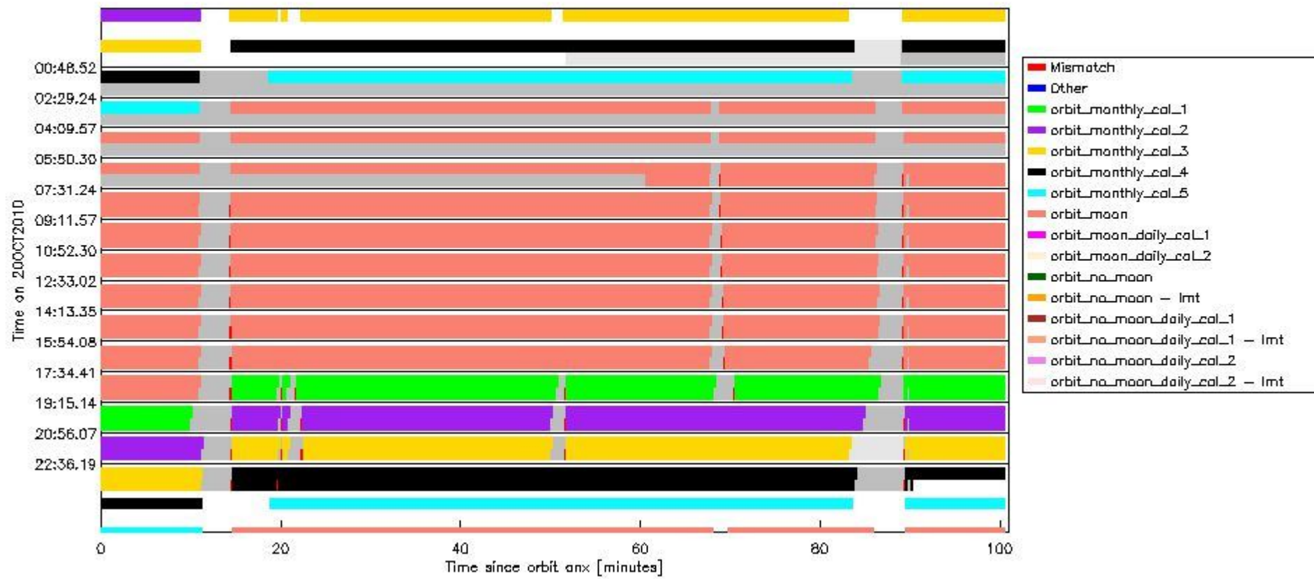
sciamachy_daily_report_level0_Any_version_20101020_6.PNG
