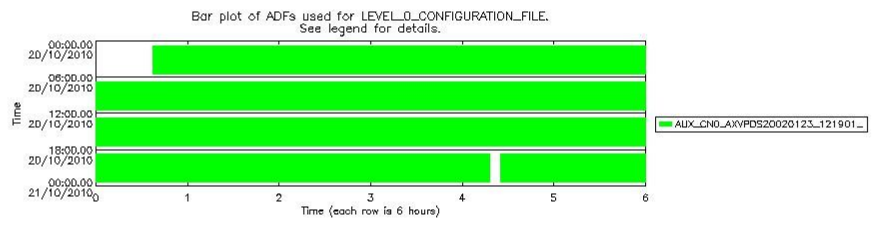
sciamachy_daily_report_level0_Any_version_20101020_7.PNG
