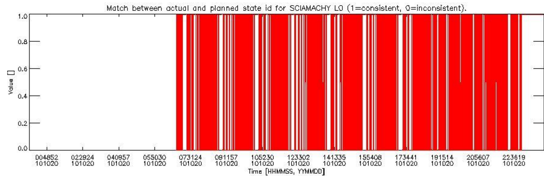
sciamachy_daily_report_level0_Any_version_20101020_5.PNG
