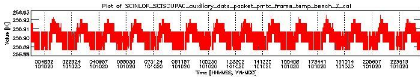
sciamachy_daily_report_level0_Any_version_20101020_1.PNG
