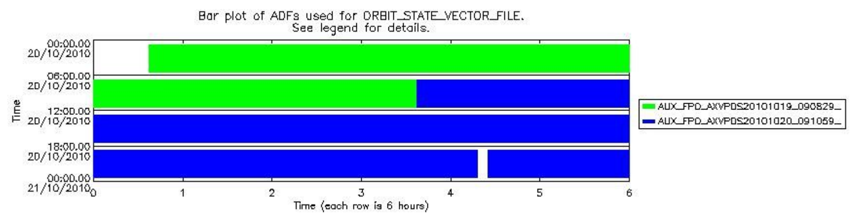
sciamachy_daily_report_level0_Any_version_20101020_8.PNG
