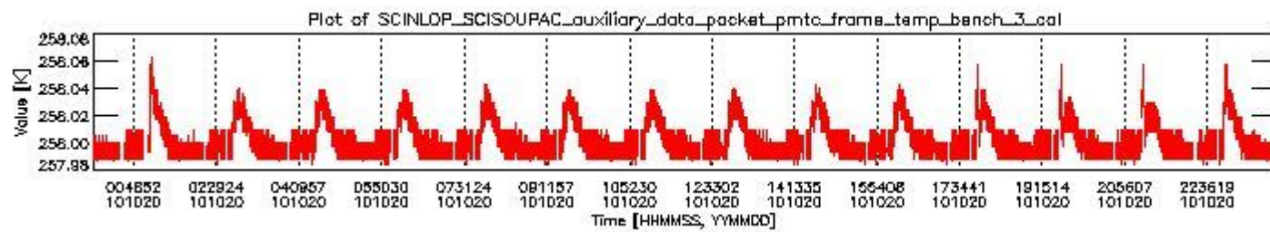
sciamachy_daily_report_level0_Any_version_20101020_2.PNG
