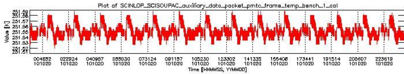
sciamachy_daily_report_level0_Any_version_20101020_0.PNG
