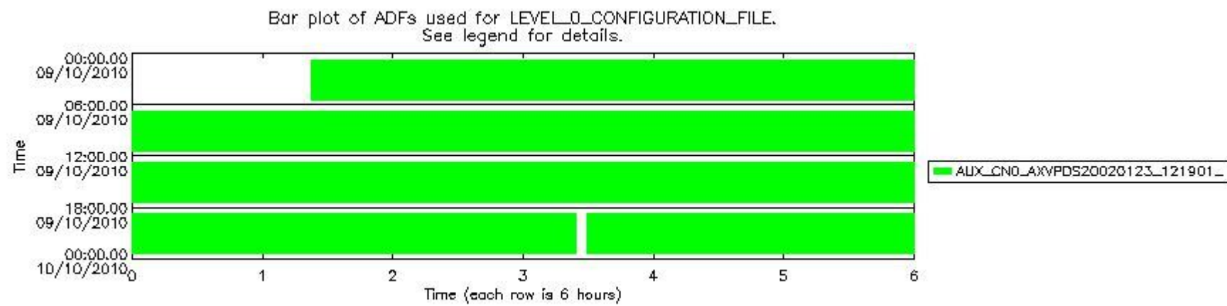
sciamachy_daily_report_level0_Any_version_20101009_7.PNG
