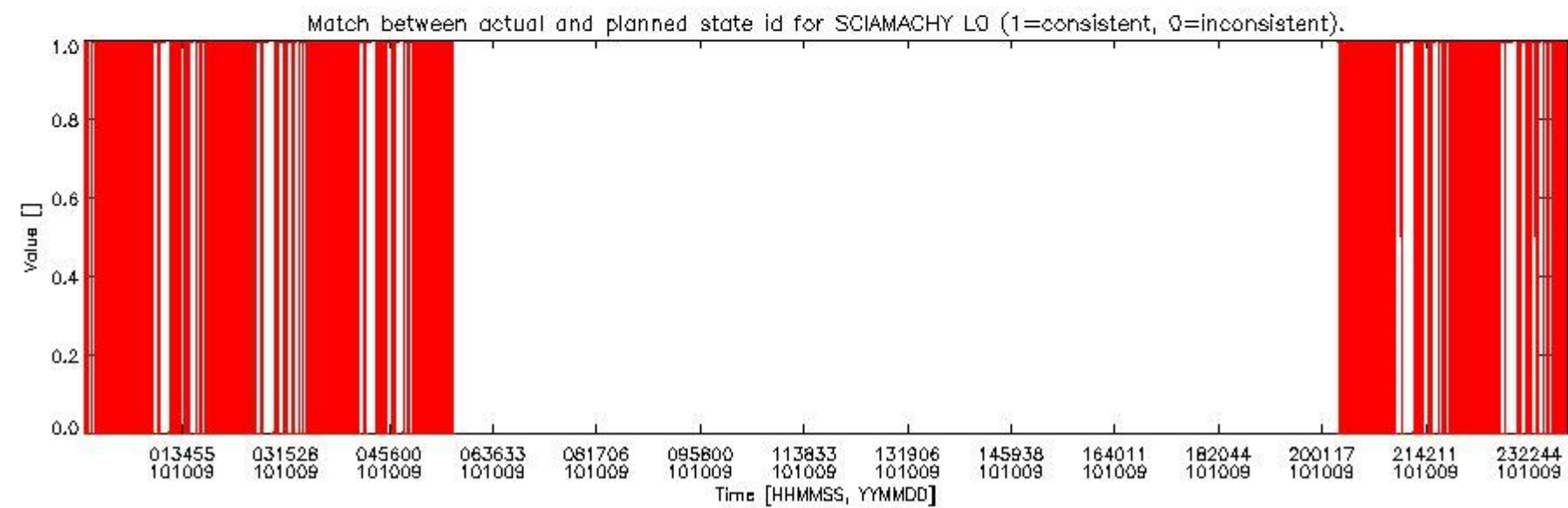
sciamachy_daily_report_level0_Any_version_20101009_5.PNG
