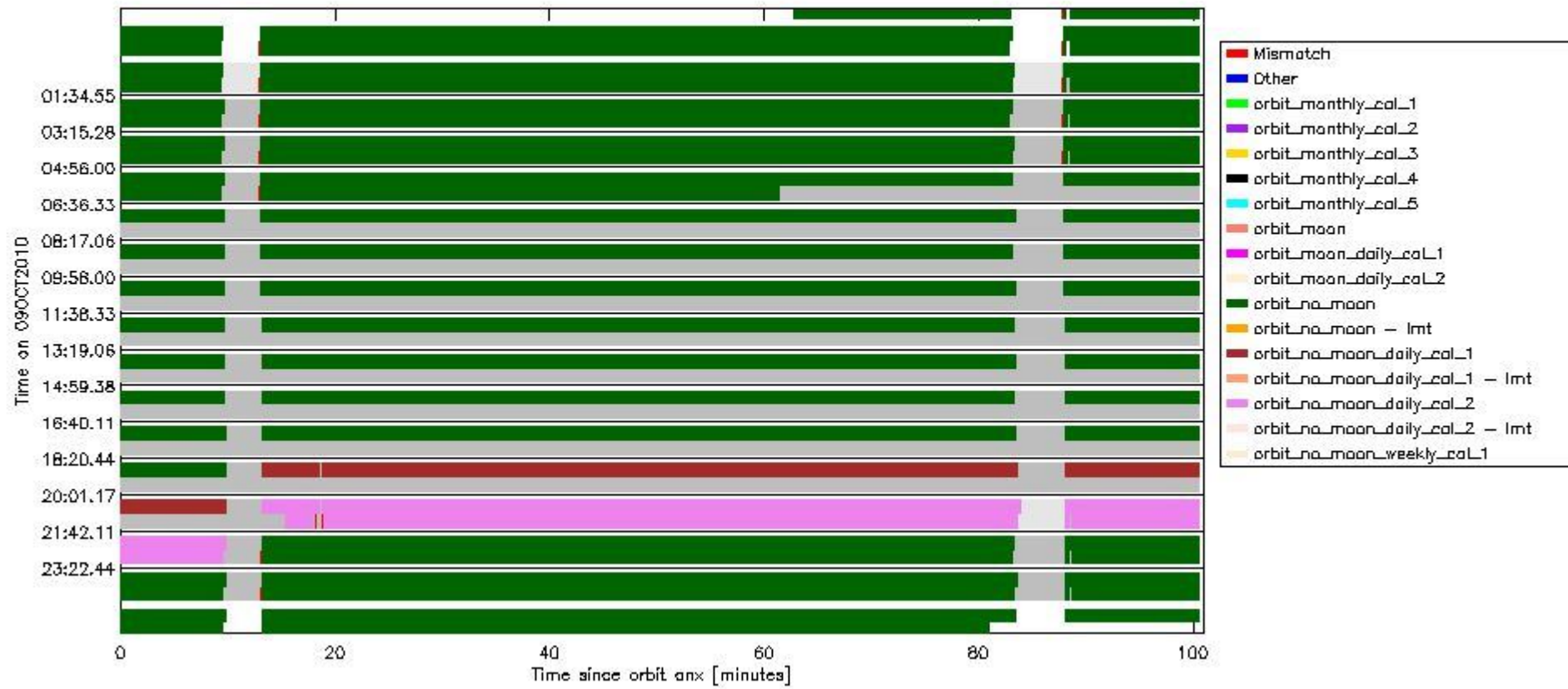
sciamachy_daily_report_level0_Any_version_20101009_6.PNG
