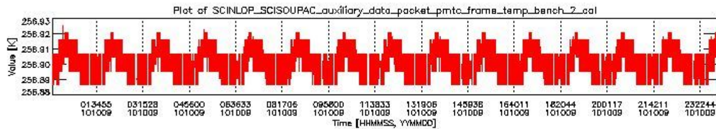
sciamachy_daily_report_level0_Any_version_20101009_1.PNG
