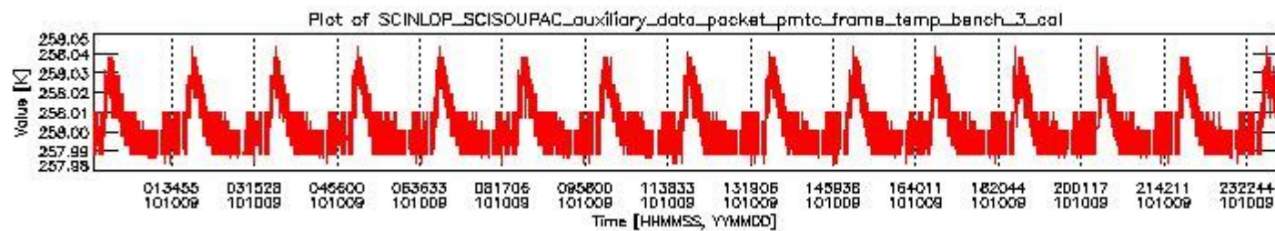
sciamachy_daily_report_level0_Any_version_20101009_2.PNG
