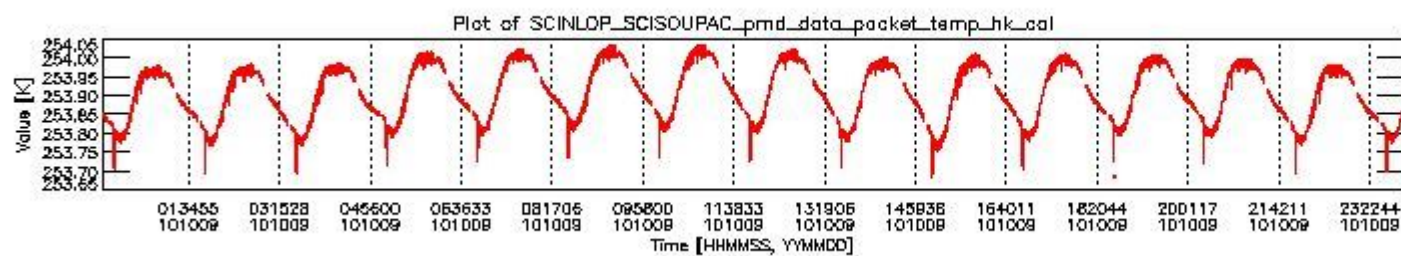
sciamachy_daily_report_level0_Any_version_20101009_3.PNG
