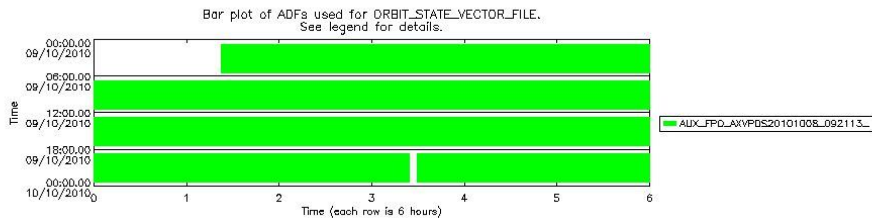
sciamachy_daily_report_level0_Any_version_20101009_8.PNG
