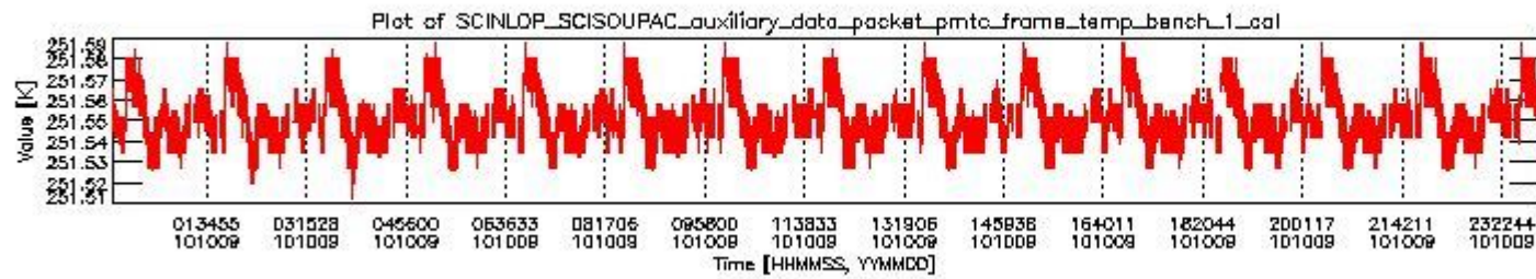
sciamachy_daily_report_level0_Any_version_20101009_0.PNG
