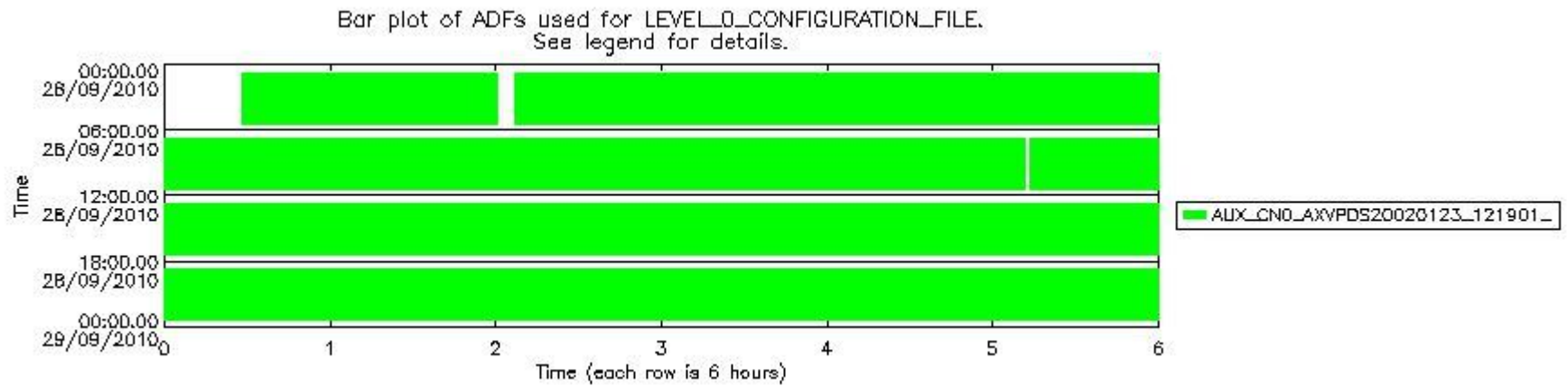
sciamachy_daily_report_level0_Any_version_20100928_7.PNG
