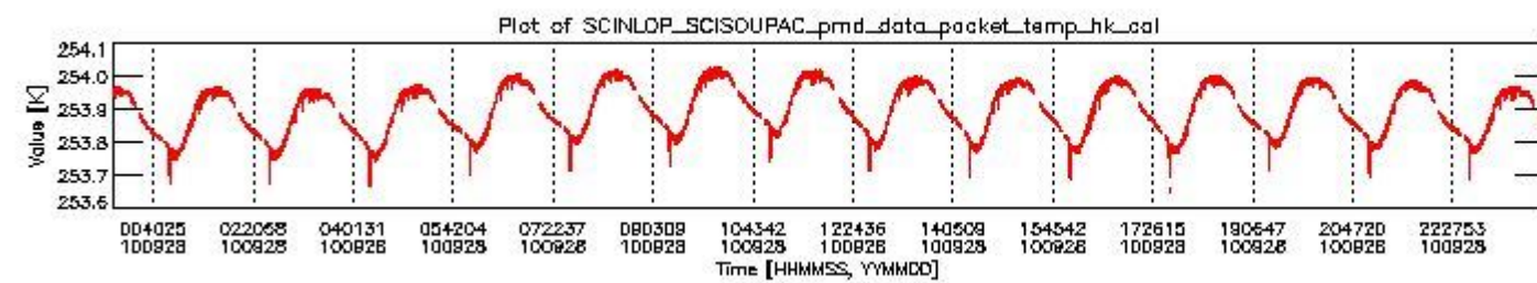
sciamachy_daily_report_level0_Any_version_20100928_3.PNG
