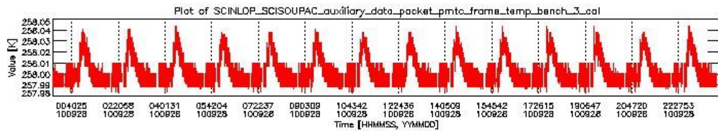
sciamachy_daily_report_level0_Any_version_20100928_2.PNG
