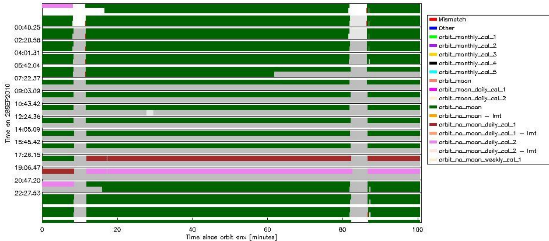
sciamachy_daily_report_level0_Any_version_20100928_6.PNG
