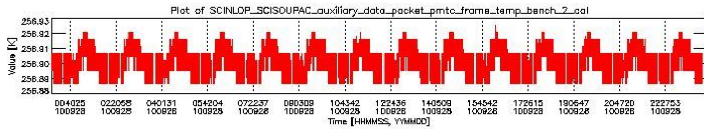
sciamachy_daily_report_level0_Any_version_20100928_1.PNG
