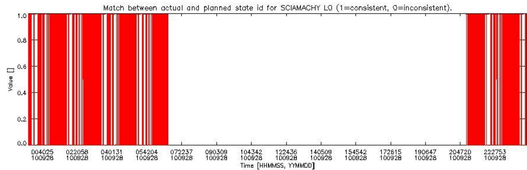
sciamachy_daily_report_level0_Any_version_20100928_5.PNG
