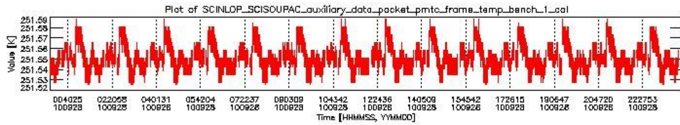
sciamachy_daily_report_level0_Any_version_20100928_0.PNG
