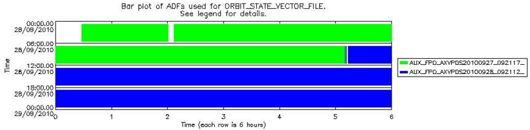
sciamachy_daily_report_level0_Any_version_20100928_8.PNG
