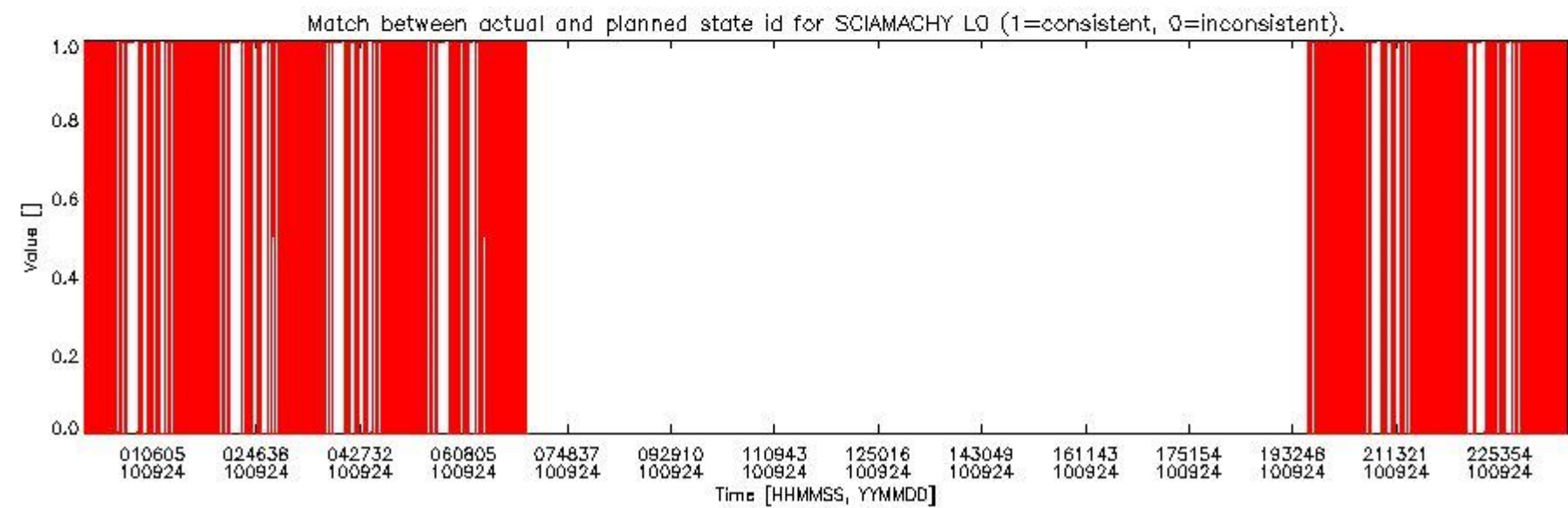
sciamachy_daily_report_level0_Any_version_20100924_5.PNG
