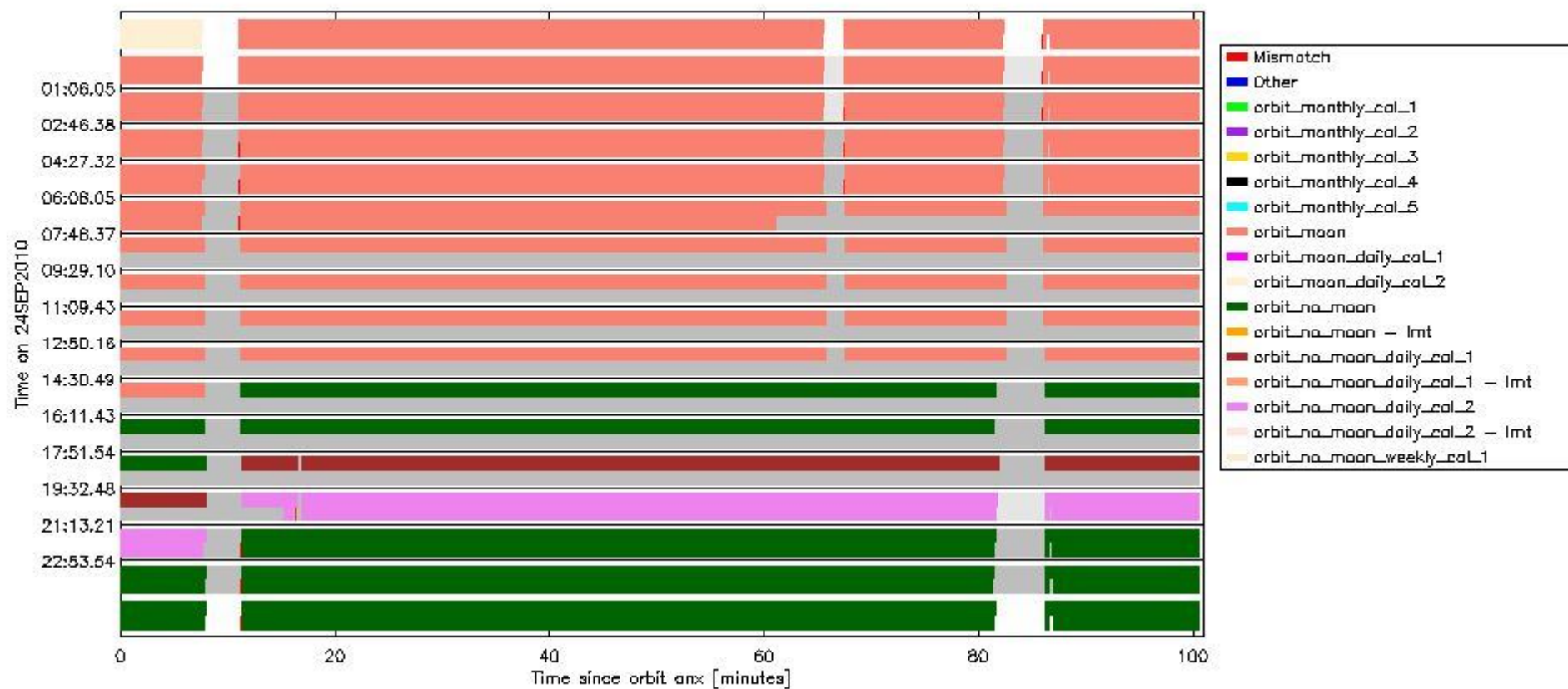
sciamachy_daily_report_level0_Any_version_20100924_6.PNG
