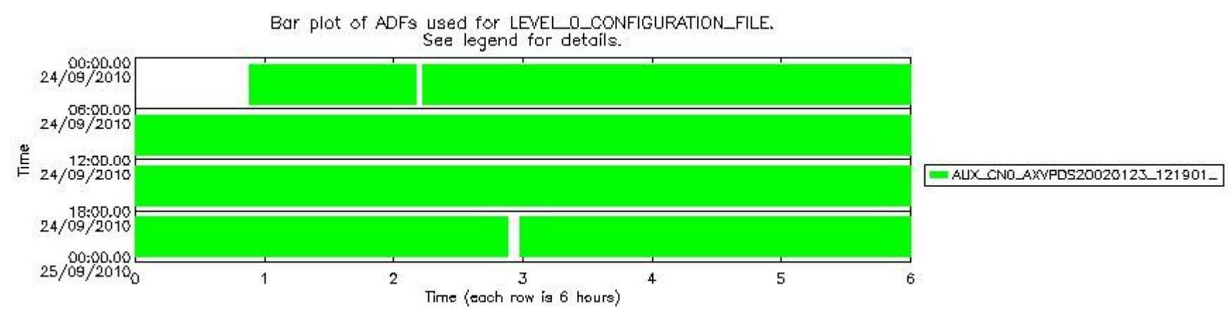
sciamachy_daily_report_level0_Any_version_20100924_7.PNG
