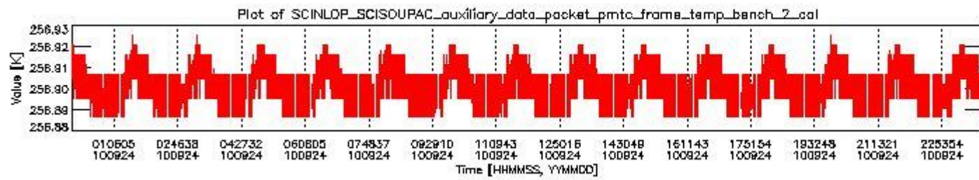
sciamachy_daily_report_level0_Any_version_20100924_1.PNG
