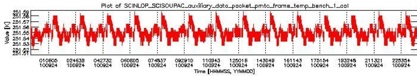
sciamachy_daily_report_level0_Any_version_20100924_0.PNG
