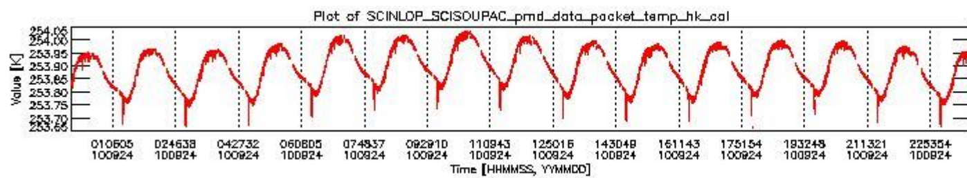
sciamachy_daily_report_level0_Any_version_20100924_3.PNG
