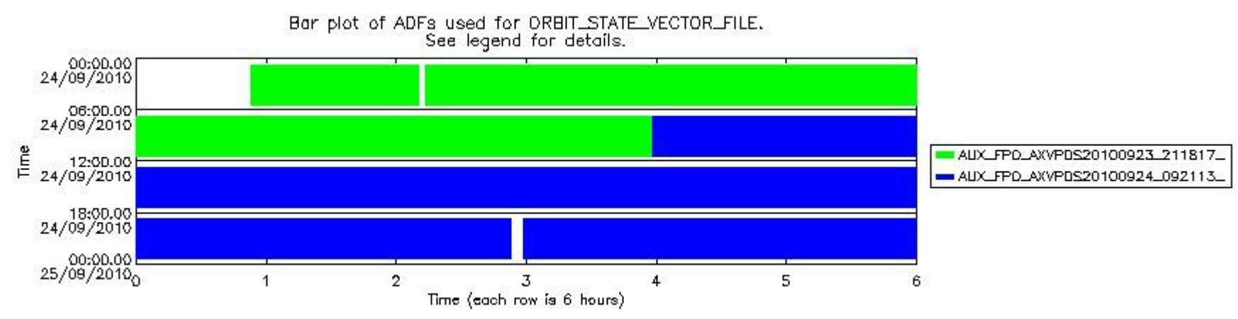
sciamachy_daily_report_level0_Any_version_20100924_8.PNG
