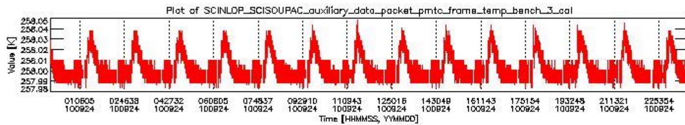
sciamachy_daily_report_level0_Any_version_20100924_2.PNG
