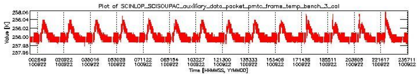
sciamachy_daily_report_level0_Any_version_20100922_2.PNG
