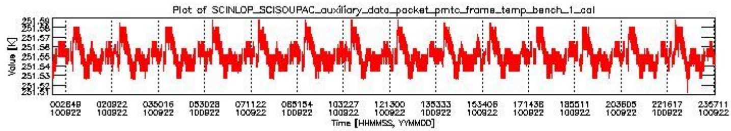
sciamachy_daily_report_level0_Any_version_20100922_0.PNG
