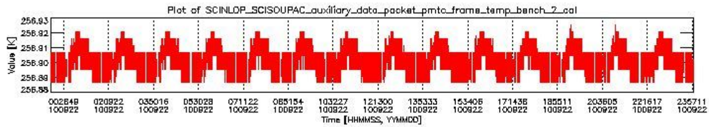
sciamachy_daily_report_level0_Any_version_20100922_1.PNG
