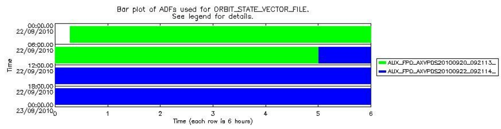
sciamachy_daily_report_level0_Any_version_20100922_7.PNG
