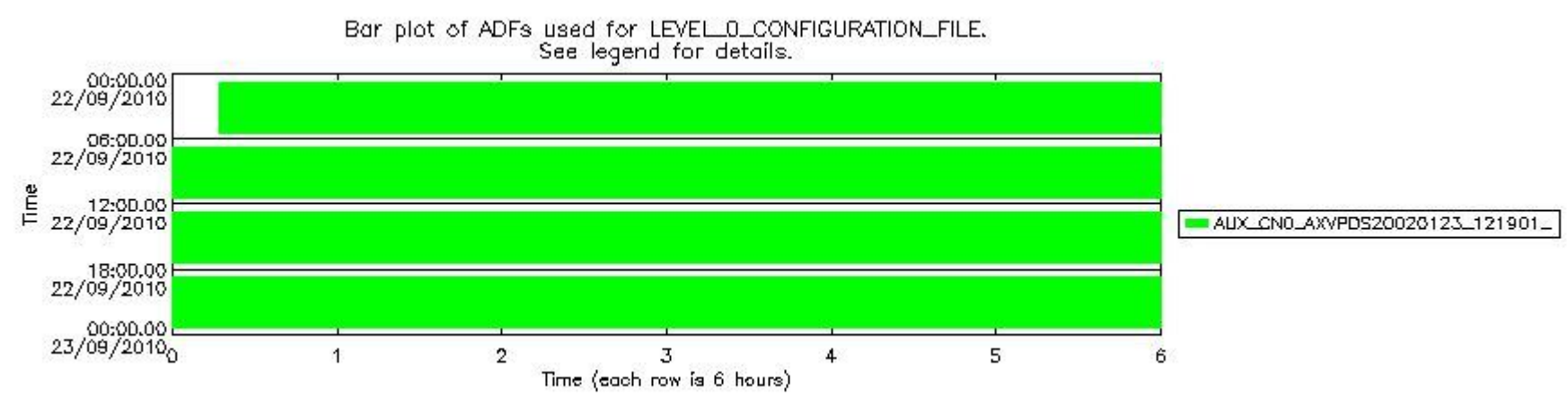
sciamachy_daily_report_level0_Any_version_20100922_6.PNG
