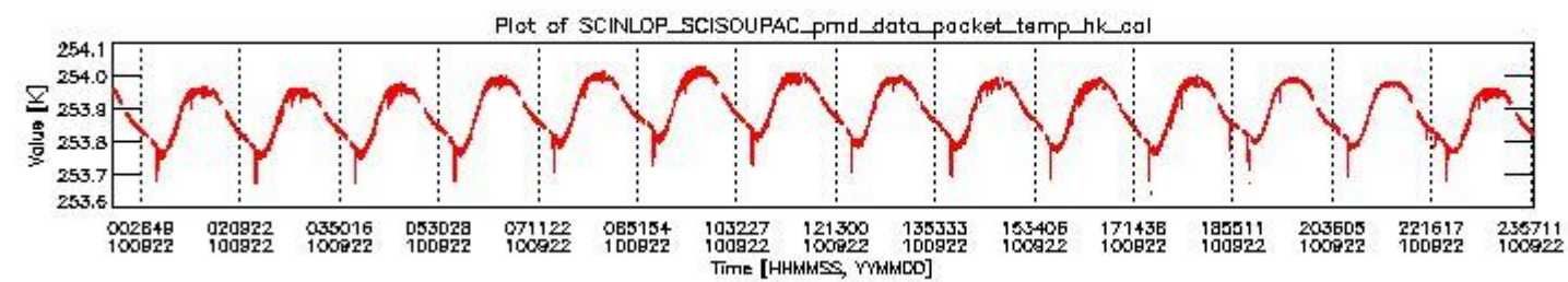
sciamachy_daily_report_level0_Any_version_20100922_3.PNG
