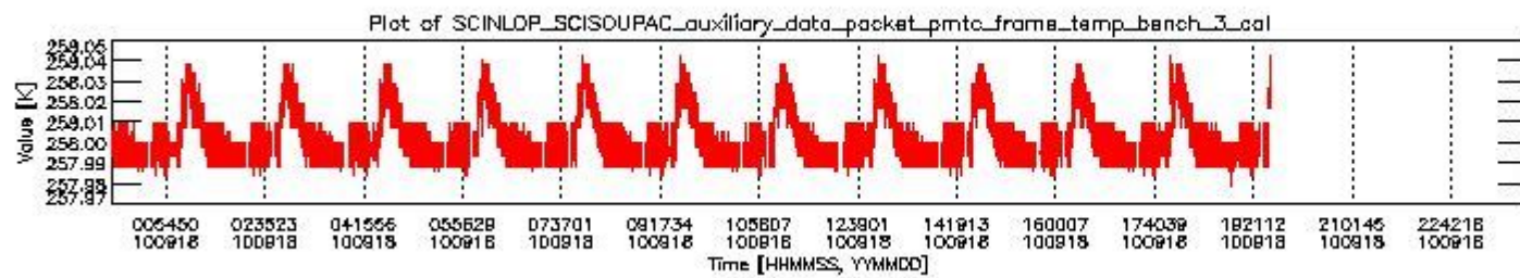
sciamachy_daily_report_level0_Any_version_20100918_2.PNG
