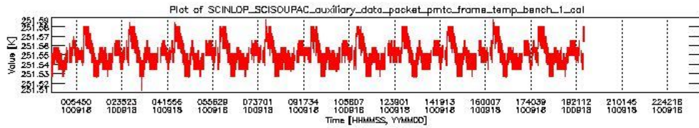
sciamachy_daily_report_level0_Any_version_20100918_0.PNG
