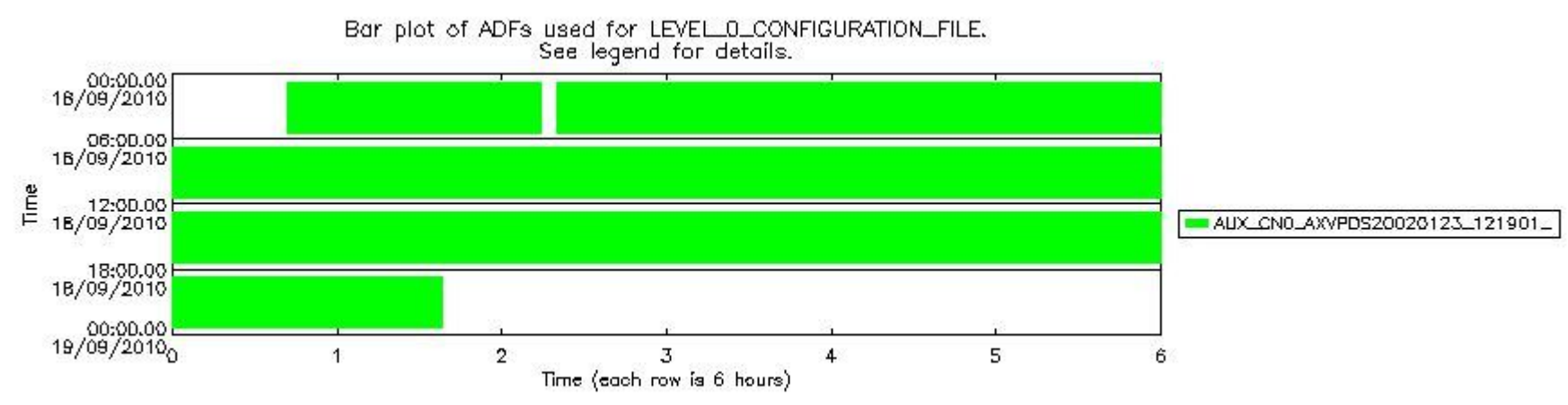
sciamachy_daily_report_level0_Any_version_20100918_6.PNG
