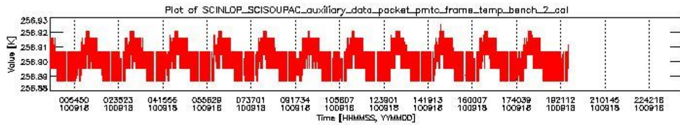
sciamachy_daily_report_level0_Any_version_20100918_1.PNG
