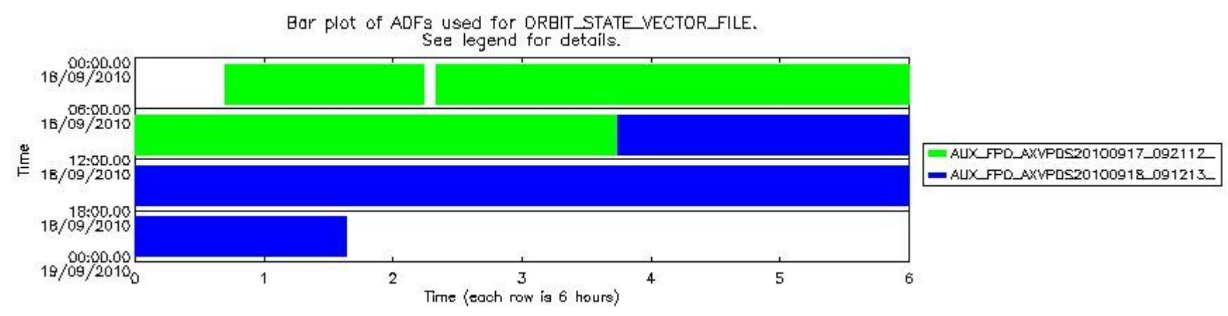
sciamachy_daily_report_level0_Any_version_20100918_7.PNG
