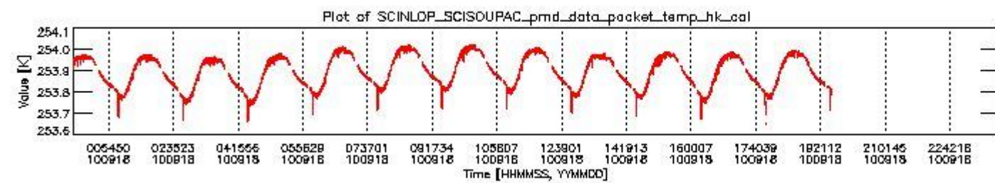
sciamachy_daily_report_level0_Any_version_20100918_3.PNG
