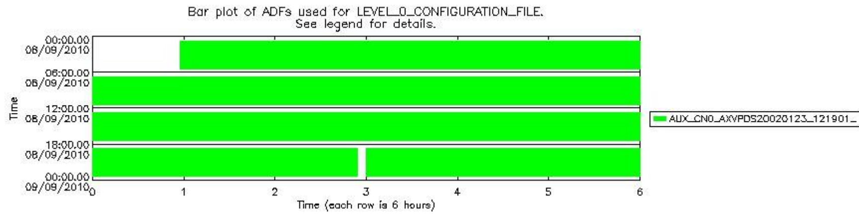
sciamachy_daily_report_level0_Any_version_20100908_6.PNG
