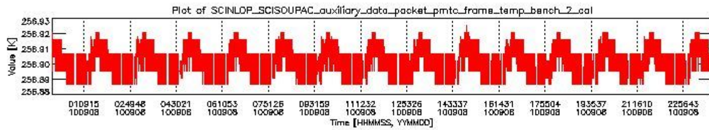
sciamachy_daily_report_level0_Any_version_20100908_1.PNG
