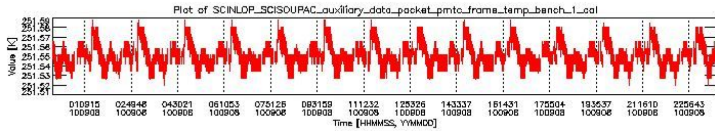
sciamachy_daily_report_level0_Any_version_20100908_0.PNG
