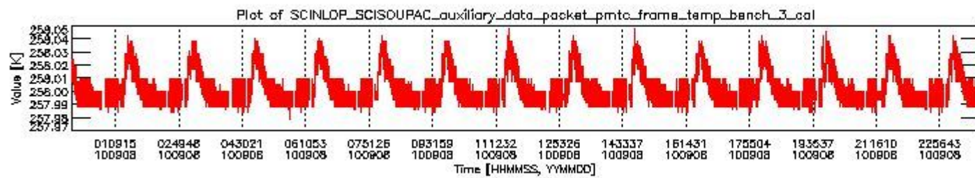
sciamachy_daily_report_level0_Any_version_20100908_2.PNG
