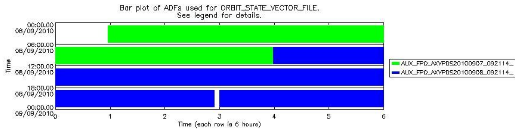
sciamachy_daily_report_level0_Any_version_20100908_7.PNG
