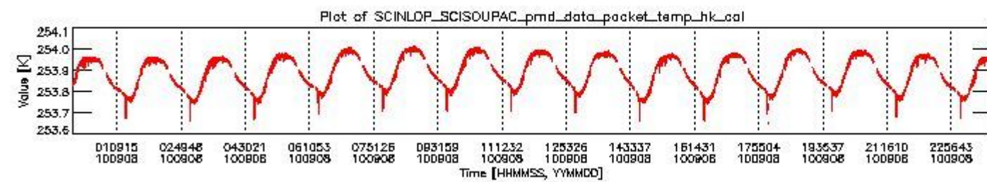
sciamachy_daily_report_level0_Any_version_20100908_3.PNG
