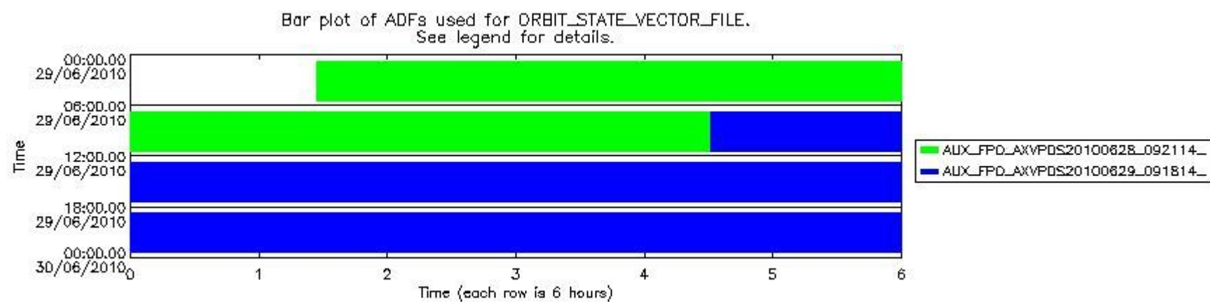
sciamachy_daily_report_level0_Any_version_20100629_7.PNG
