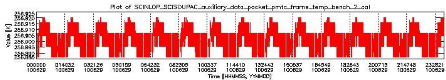
sciamachy_daily_report_level0_Any_version_20100629_1.PNG
