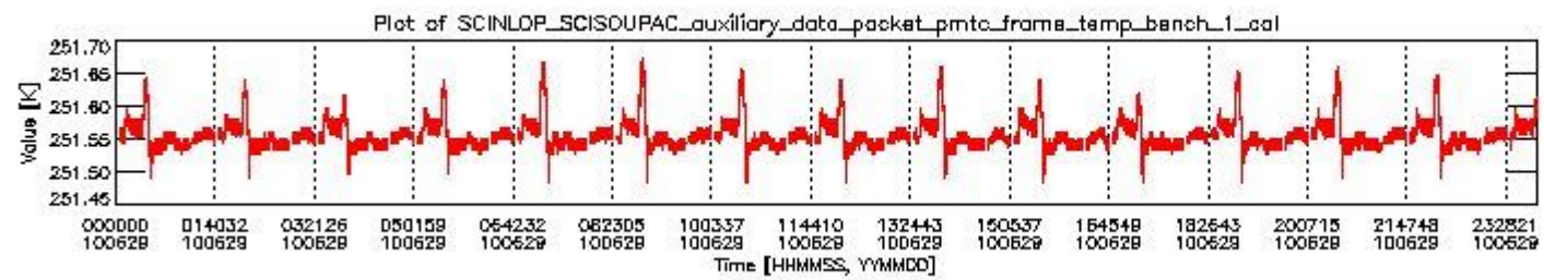
sciamachy_daily_report_level0_Any_version_20100629_0.PNG
