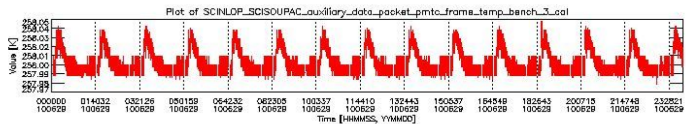
sciamachy_daily_report_level0_Any_version_20100629_2.PNG
