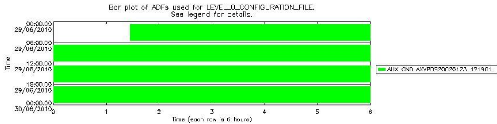
sciamachy_daily_report_level0_Any_version_20100629_6.PNG
