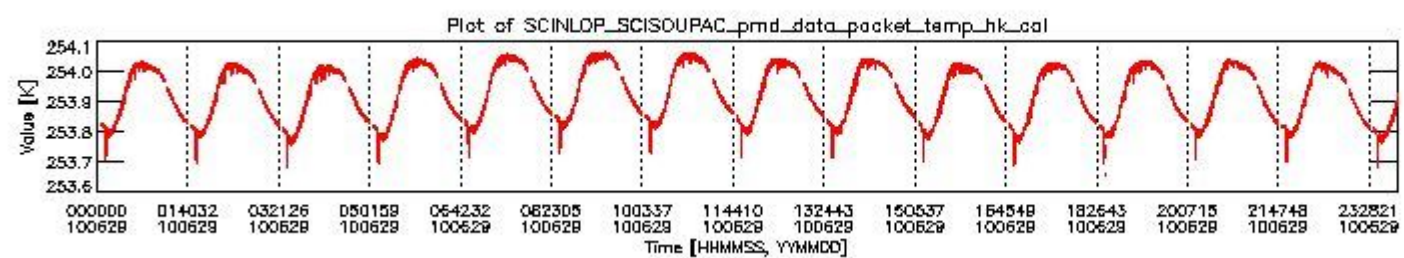
sciamachy_daily_report_level0_Any_version_20100629_3.PNG
