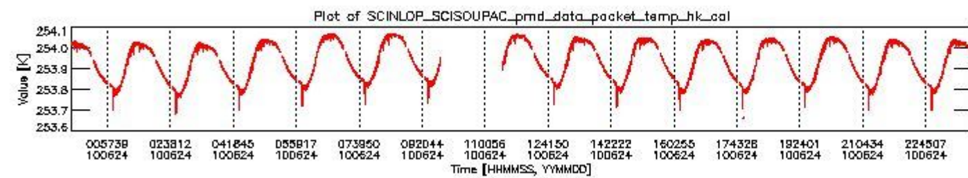
sciamachy_daily_report_level0_Any_version_20100624_3.PNG
