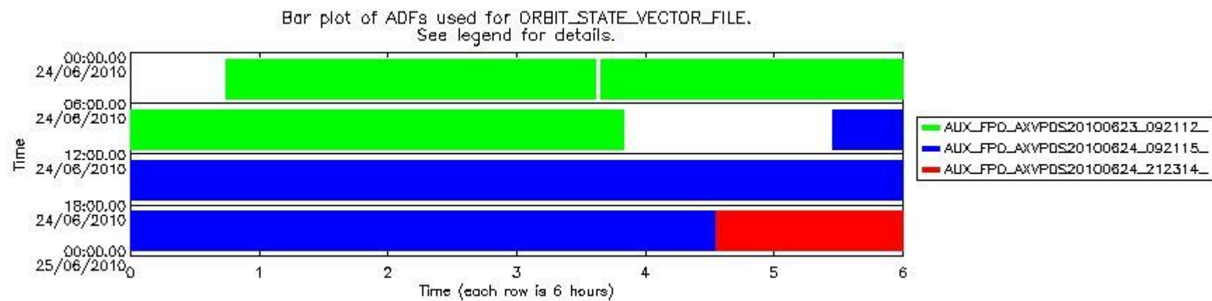
sciamachy_daily_report_level0_Any_version_20100624_7.PNG
