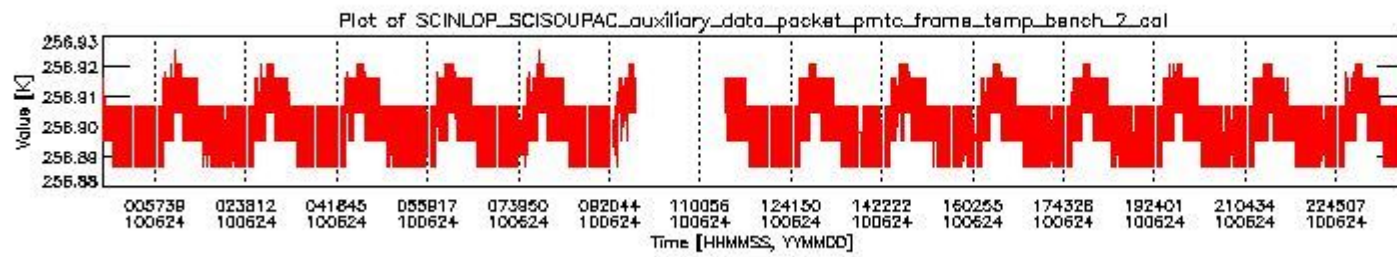
sciamachy_daily_report_level0_Any_version_20100624_1.PNG
