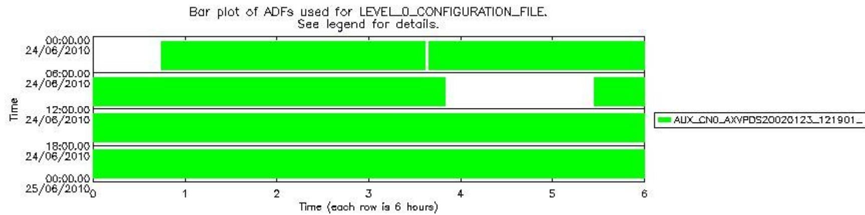
sciamachy_daily_report_level0_Any_version_20100624_6.PNG
