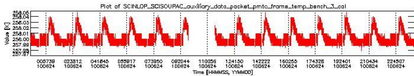
sciamachy_daily_report_level0_Any_version_20100624_2.PNG
