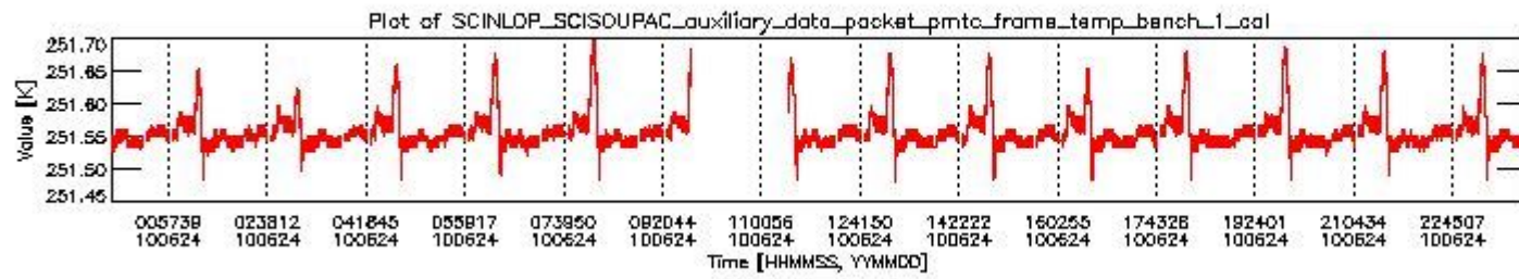
sciamachy_daily_report_level0_Any_version_20100624_0.PNG
