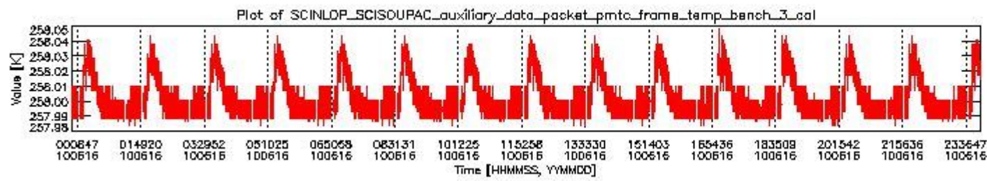
sciamachy_daily_report_level0_Any_version_20100616_2.PNG
