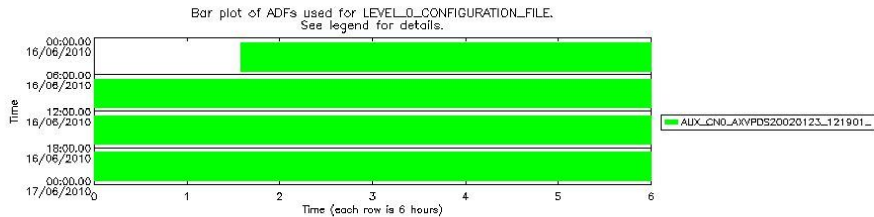
sciamachy_daily_report_level0_Any_version_20100616_6.PNG
