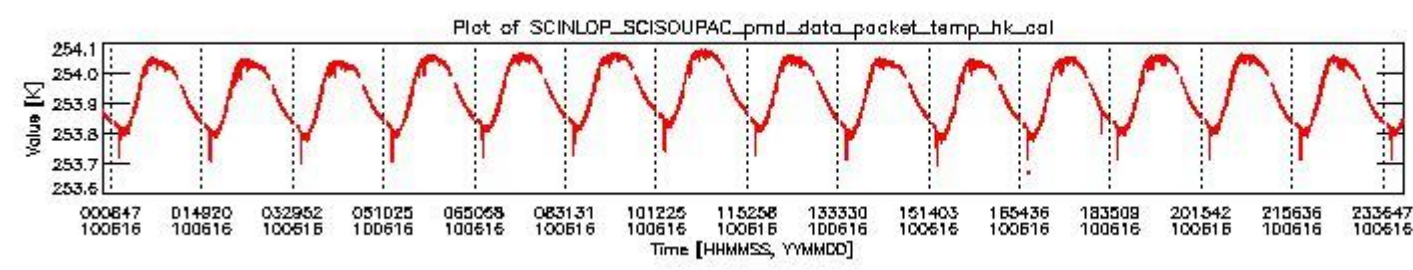
sciamachy_daily_report_level0_Any_version_20100616_3.PNG
