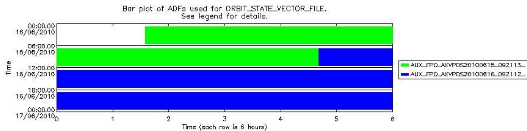
sciamachy_daily_report_level0_Any_version_20100616_7.PNG
