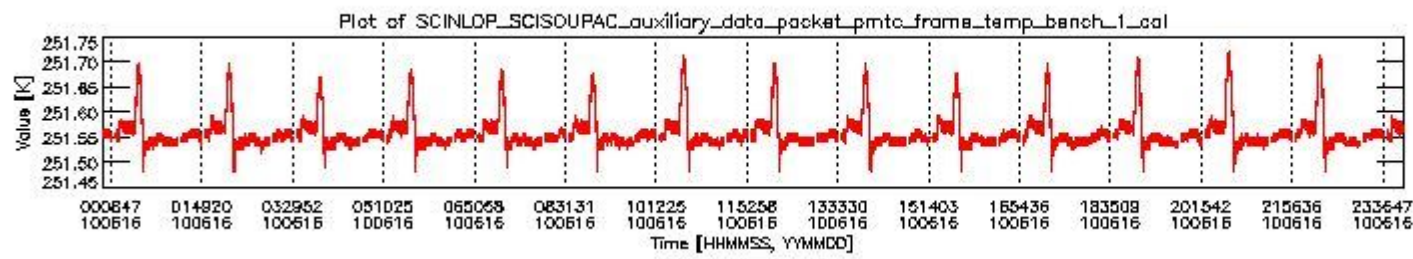
sciamachy_daily_report_level0_Any_version_20100616_0.PNG
