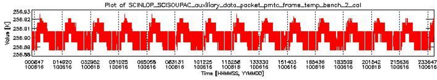
sciamachy_daily_report_level0_Any_version_20100616_1.PNG
