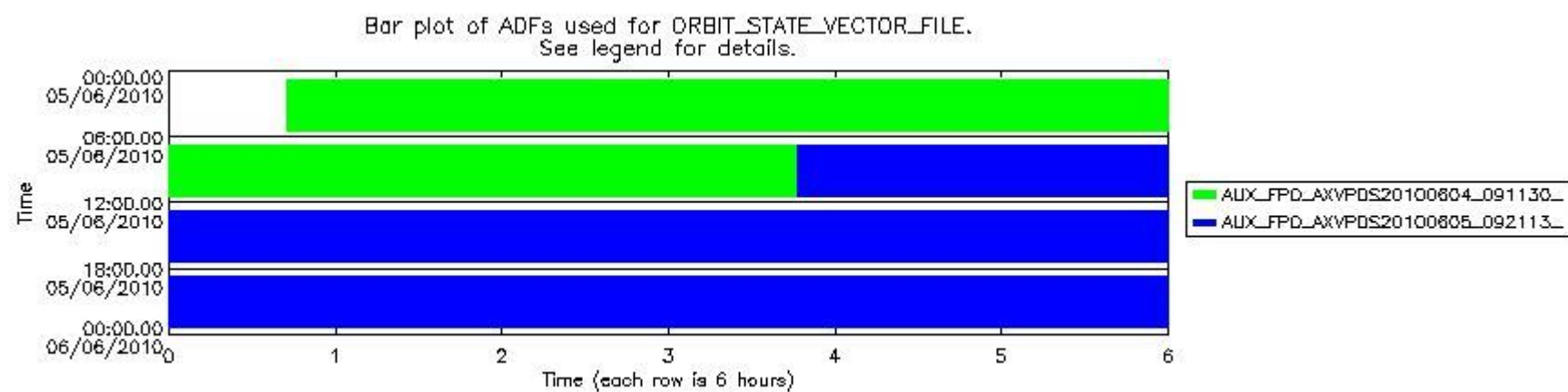
sciamachy_daily_report_level0_Any_version_20100605_8.PNG
