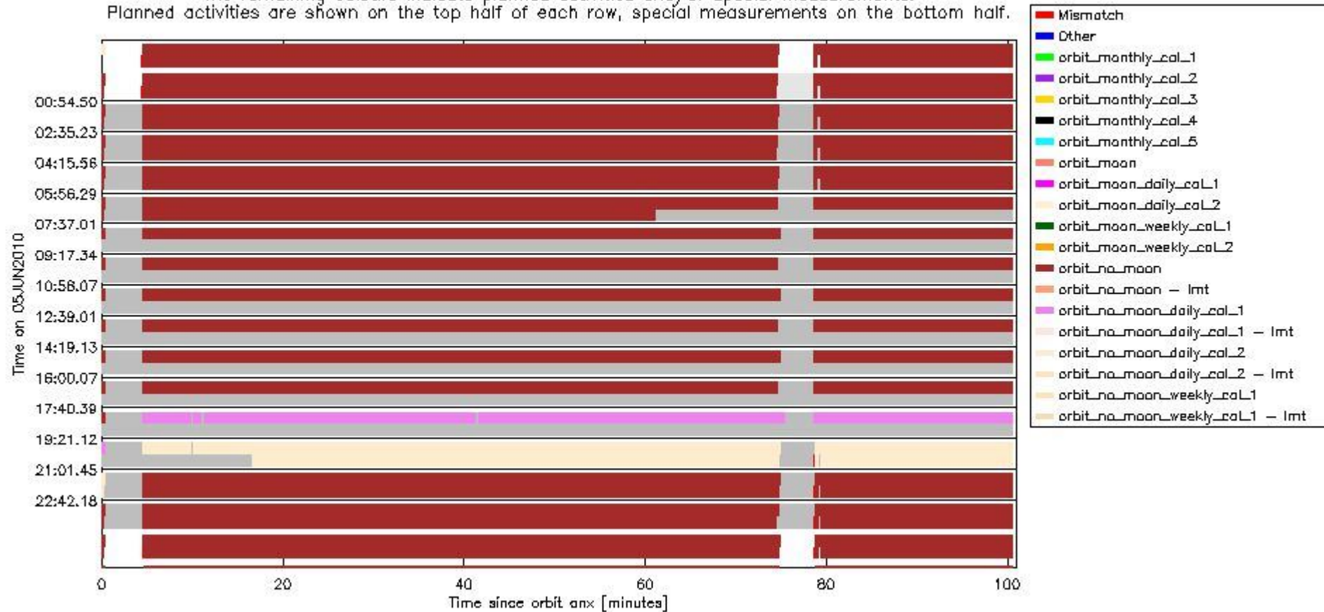
sciamachy_daily_report_level0_Any_version_20100605_6.PNG
