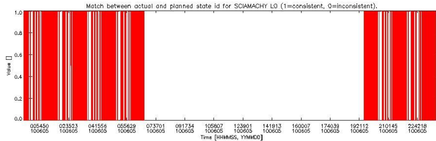
sciamachy_daily_report_level0_Any_version_20100605_5.PNG
