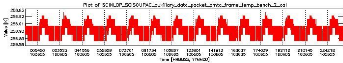
sciamachy_daily_report_level0_Any_version_20100605_1.PNG
