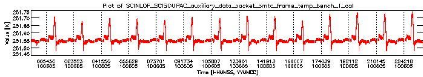
sciamachy_daily_report_level0_Any_version_20100605_0.PNG
