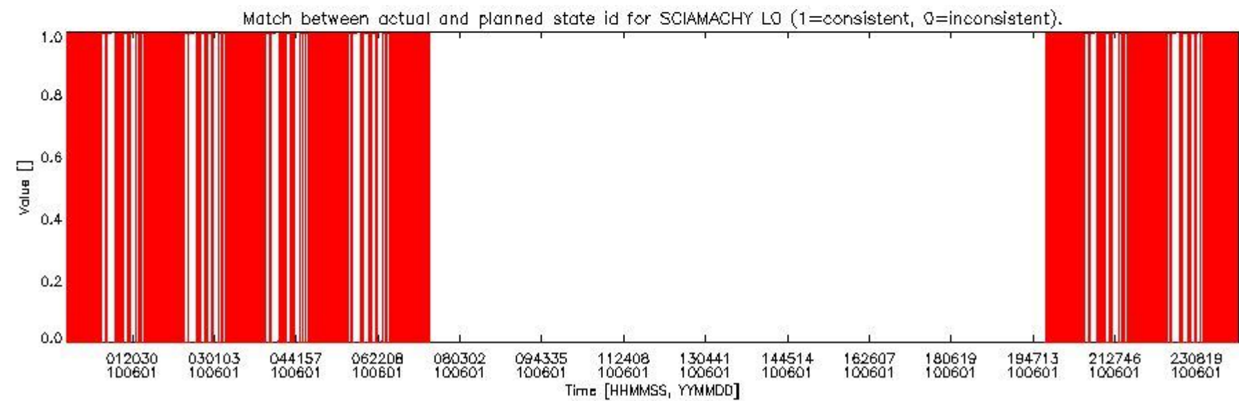
sciamachy_daily_report_level0_Any_version_20100601_5.PNG
