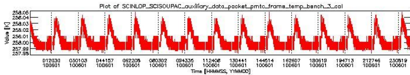
sciamachy_daily_report_level0_Any_version_20100601_2.PNG
