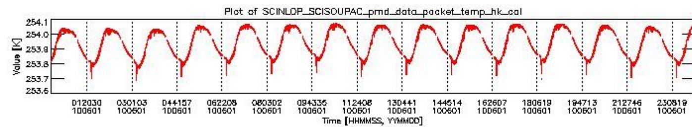
sciamachy_daily_report_level0_Any_version_20100601_3.PNG
