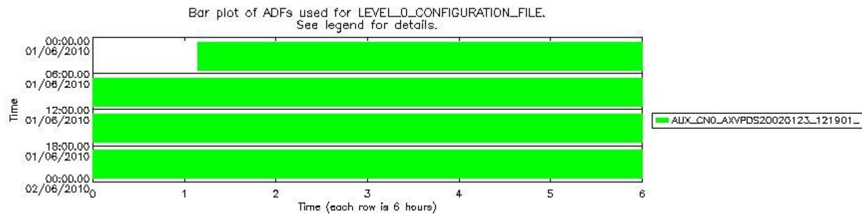
sciamachy_daily_report_level0_Any_version_20100601_7.PNG
