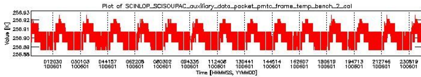
sciamachy_daily_report_level0_Any_version_20100601_1.PNG
