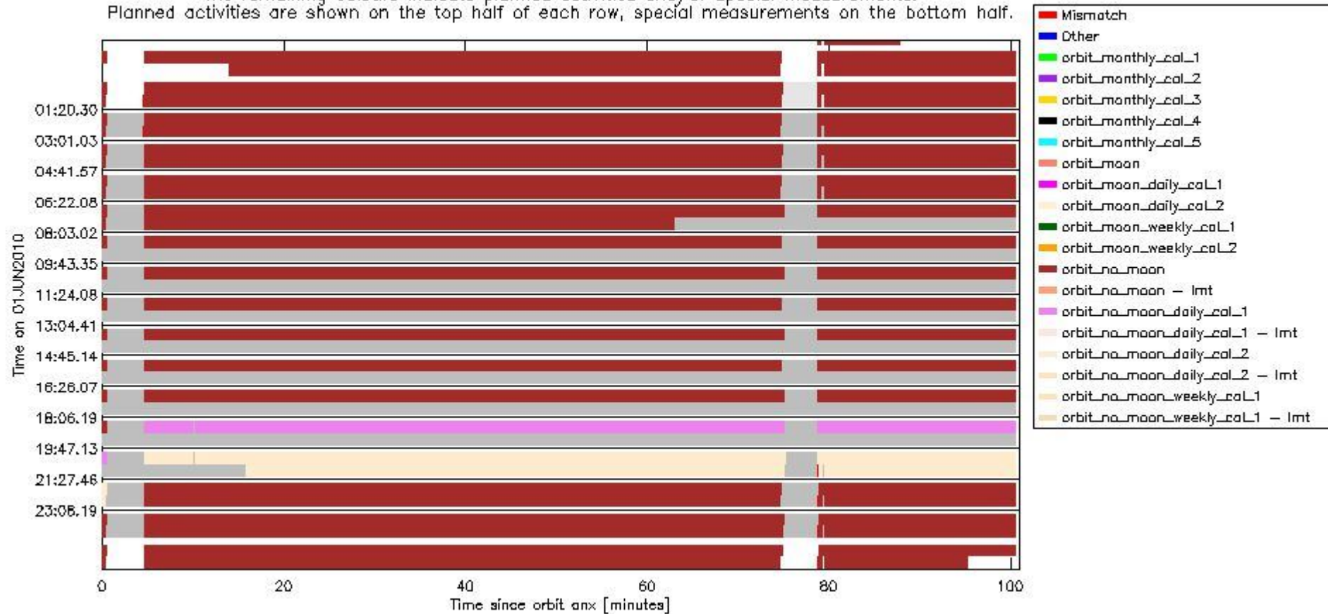
sciamachy_daily_report_level0_Any_version_20100601_6.PNG
