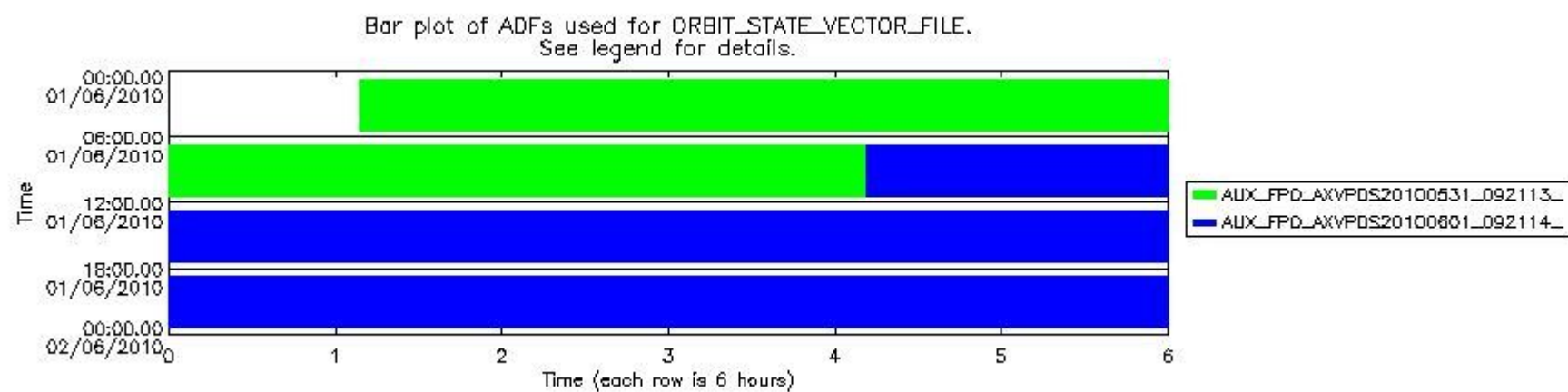
sciamachy_daily_report_level0_Any_version_20100601_8.PNG
