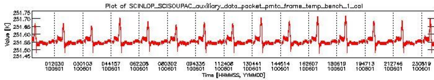
sciamachy_daily_report_level0_Any_version_20100601_0.PNG
