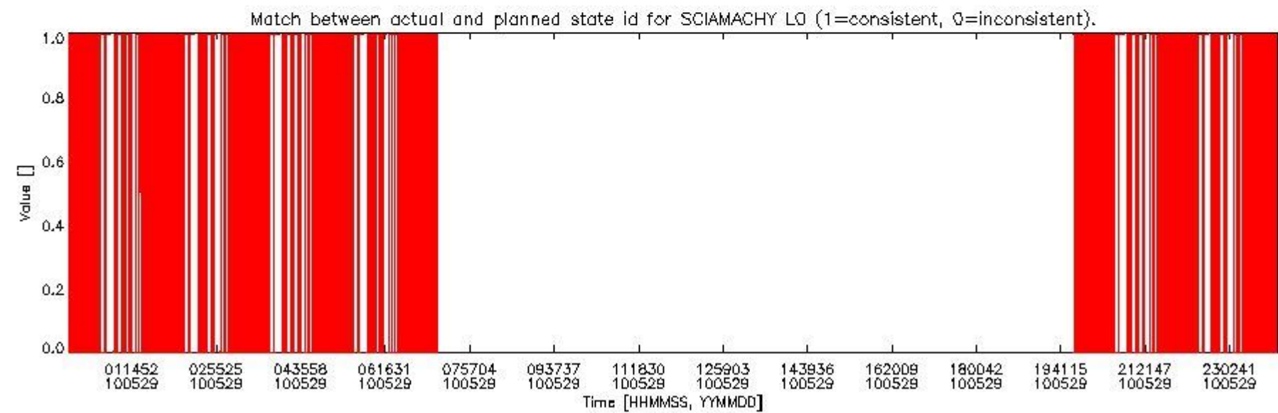
sciamachy_daily_report_level0_Any_version_20100529_5.PNG
