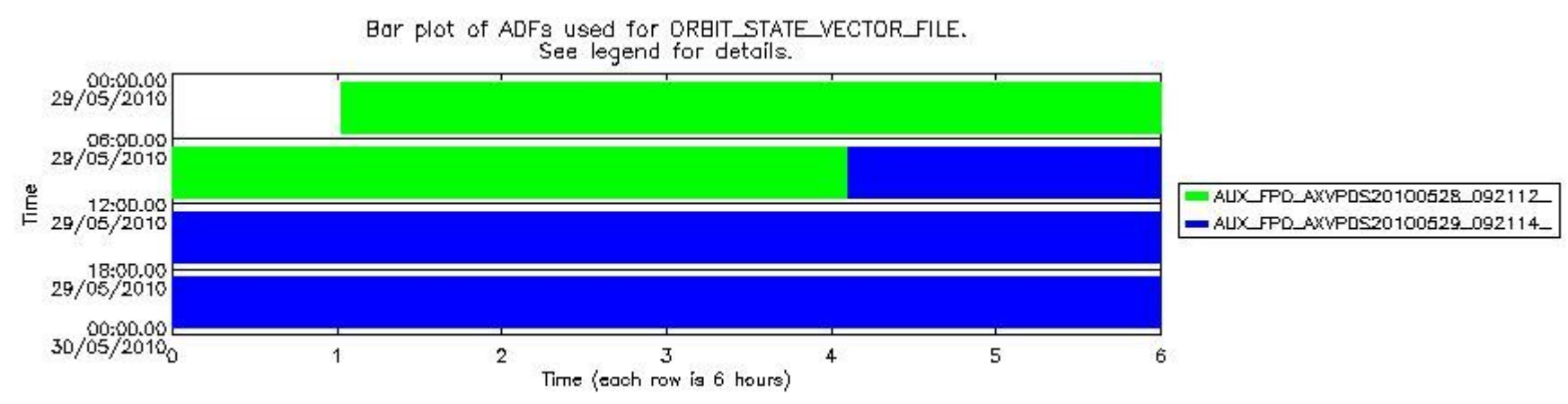
sciamachy_daily_report_level0_Any_version_20100529_8.PNG
