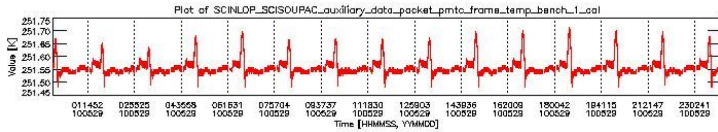
sciamachy_daily_report_level0_Any_version_20100529_0.PNG
