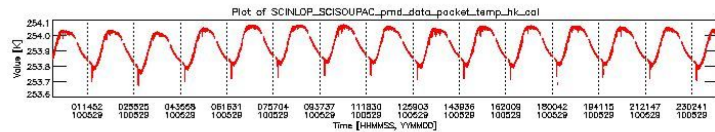
sciamachy_daily_report_level0_Any_version_20100529_3.PNG
