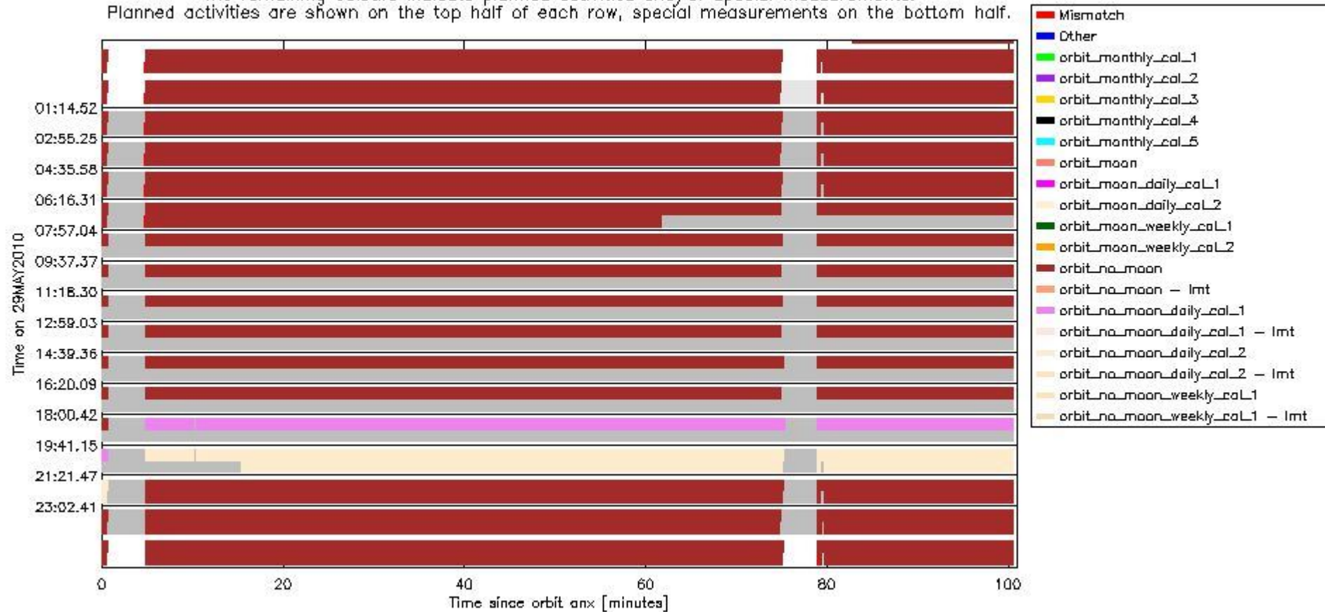
sciamachy_daily_report_level0_Any_version_20100529_6.PNG
