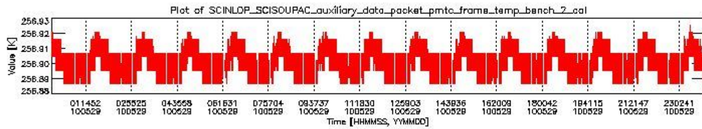
sciamachy_daily_report_level0_Any_version_20100529_1.PNG
