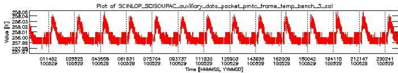
sciamachy_daily_report_level0_Any_version_20100529_2.PNG
