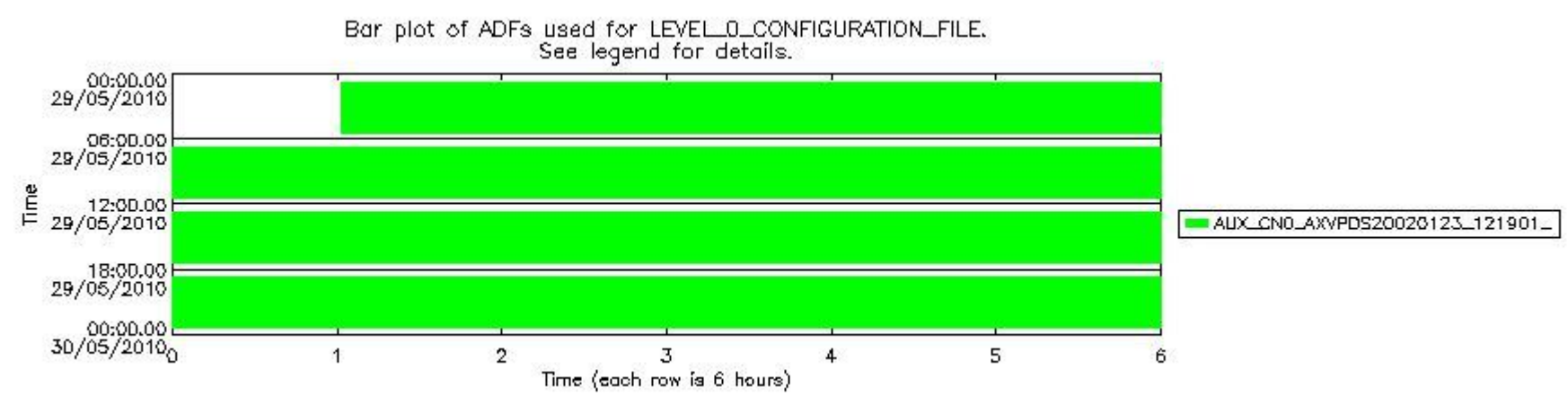
sciamachy_daily_report_level0_Any_version_20100529_7.PNG
