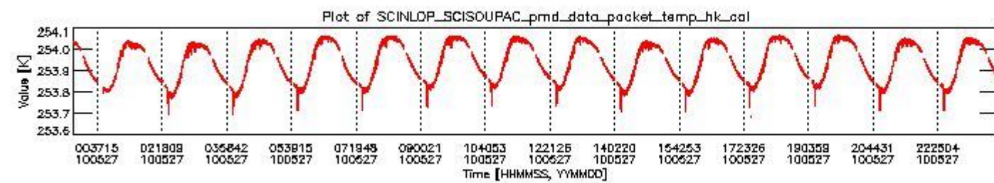
sciamachy_daily_report_level0_Any_version_20100527_3.PNG
