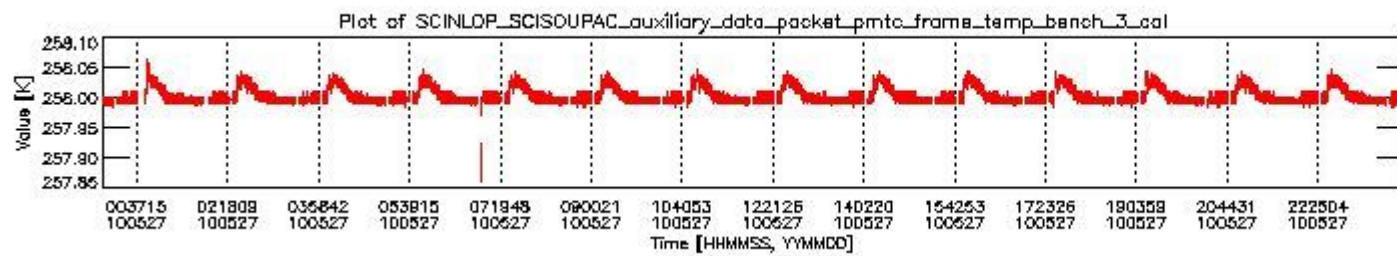
sciamachy_daily_report_level0_Any_version_20100527_2.PNG
