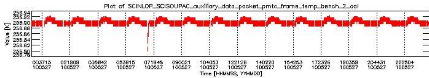
sciamachy_daily_report_level0_Any_version_20100527_1.PNG
