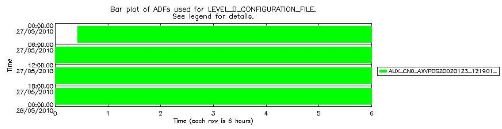
sciamachy_daily_report_level0_Any_version_20100527_7.PNG
