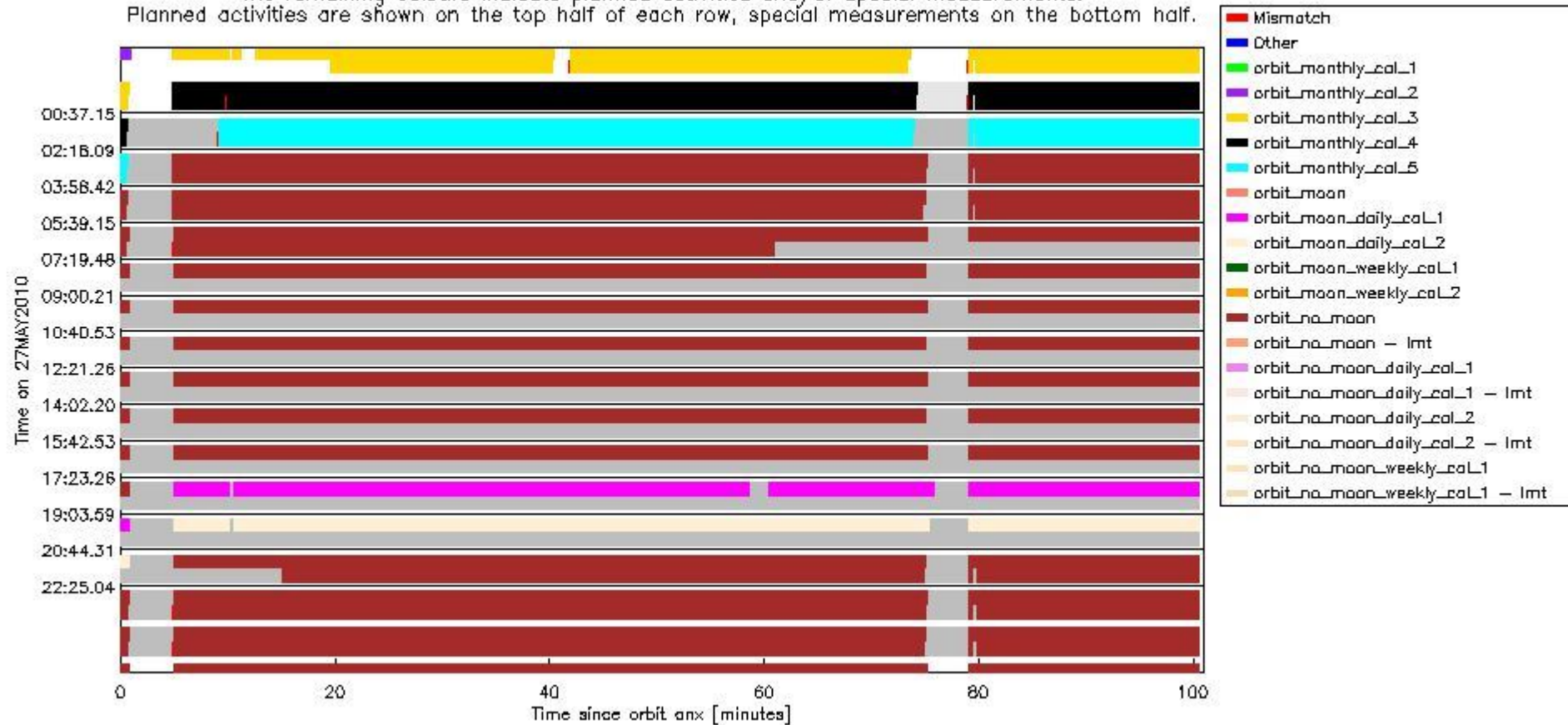
sciamachy_daily_report_level0_Any_version_20100527_6.PNG
