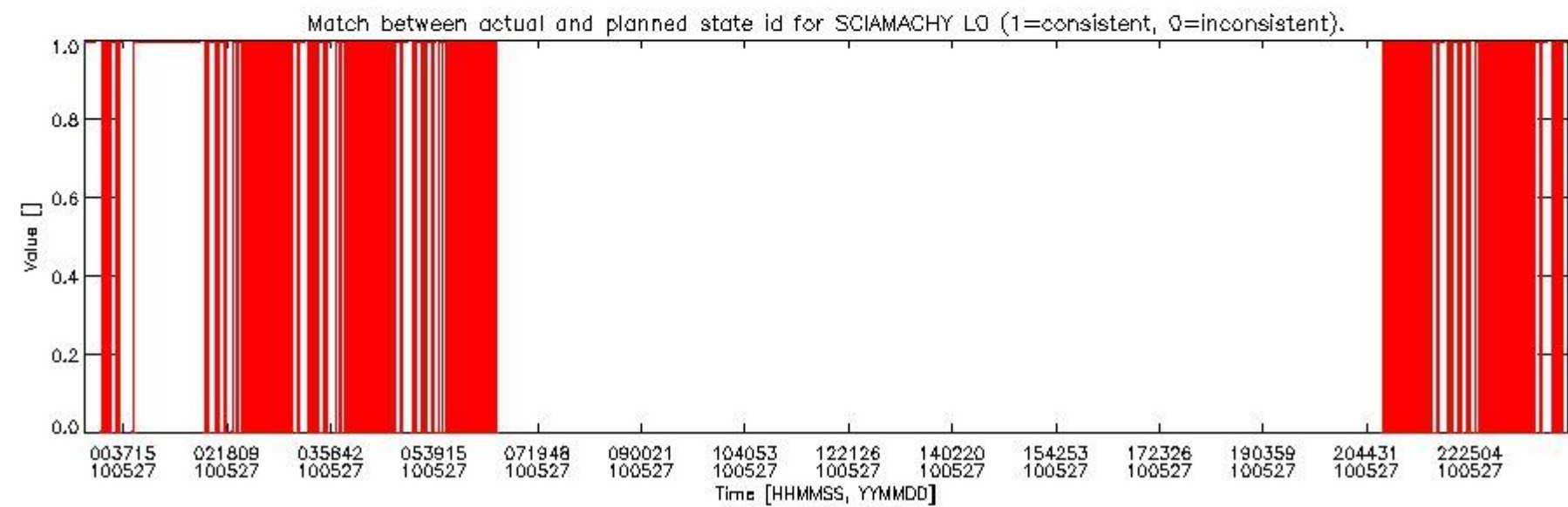
sciamachy_daily_report_level0_Any_version_20100527_5.PNG
