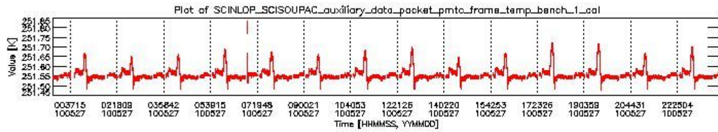
sciamachy_daily_report_level0_Any_version_20100527_0.PNG
