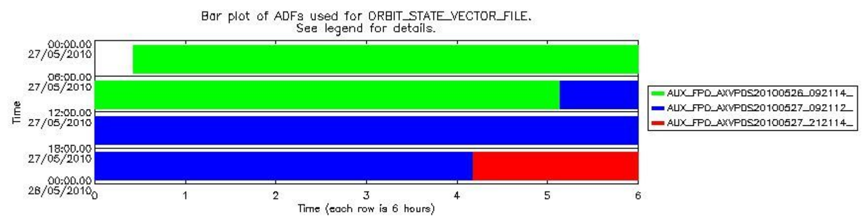
sciamachy_daily_report_level0_Any_version_20100527_8.PNG
