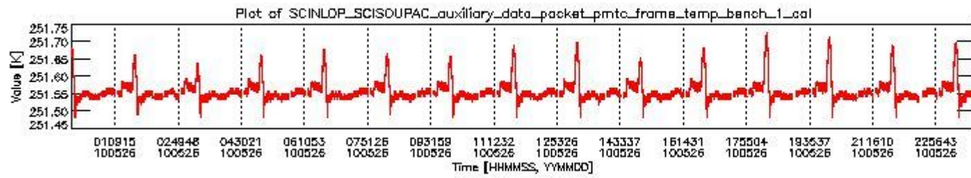
sciamachy_daily_report_level0_Any_version_20100526_0.PNG
