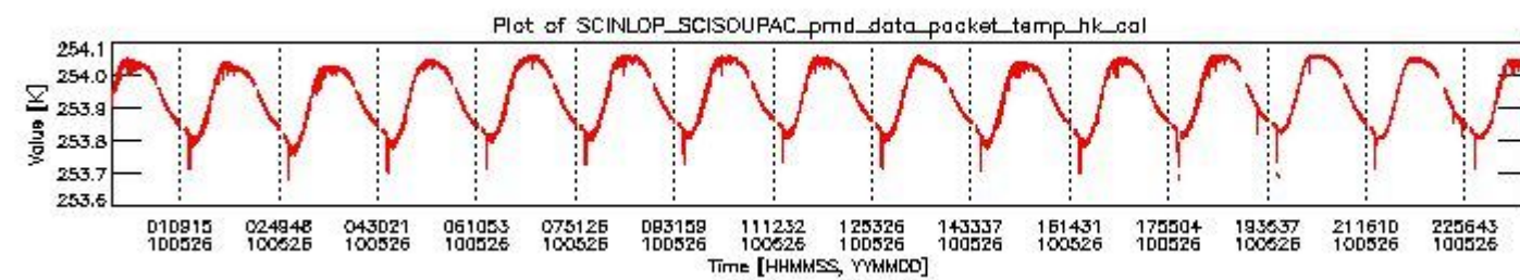
sciamachy_daily_report_level0_Any_version_20100526_3.PNG
