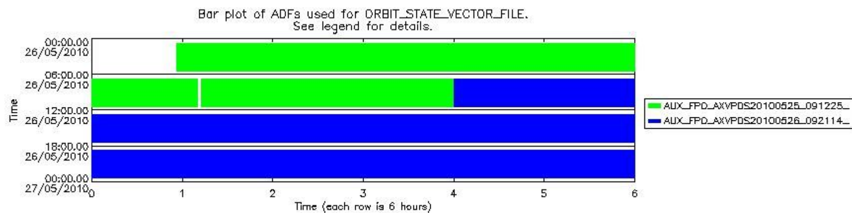
sciamachy_daily_report_level0_Any_version_20100526_8.PNG
