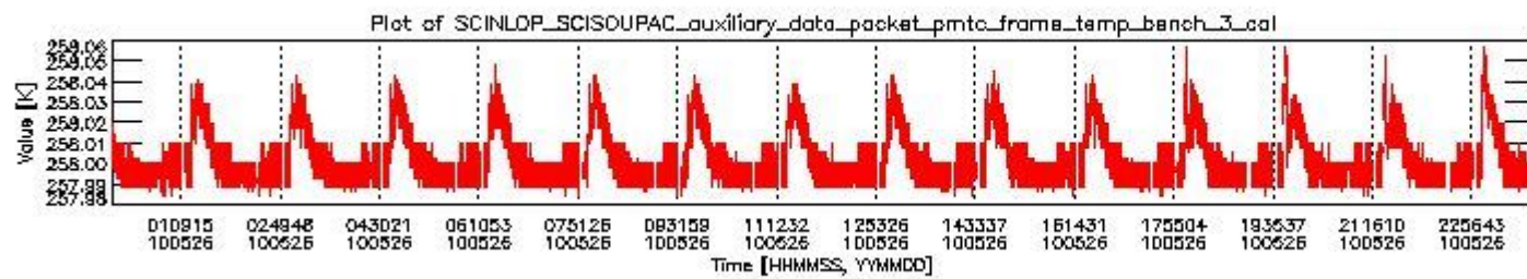
sciamachy_daily_report_level0_Any_version_20100526_2.PNG
