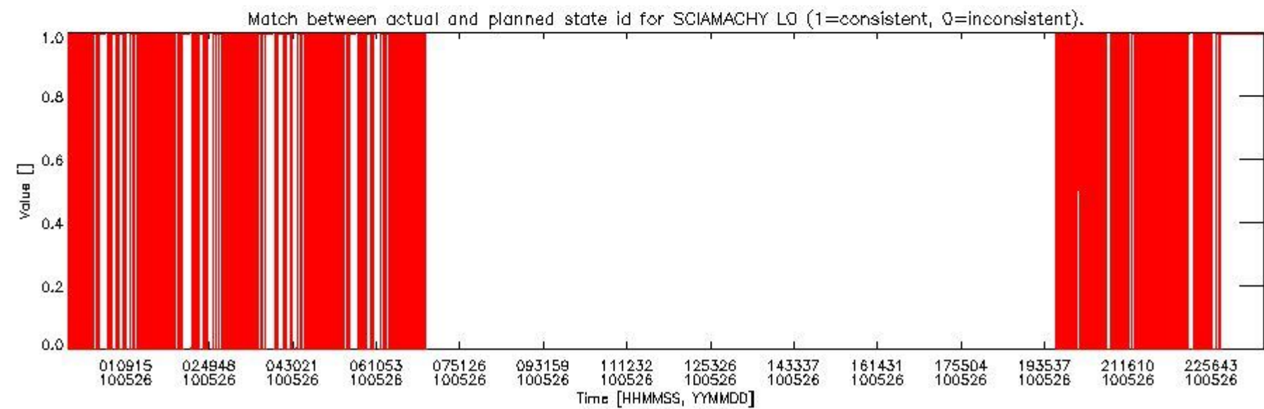
sciamachy_daily_report_level0_Any_version_20100526_5.PNG
