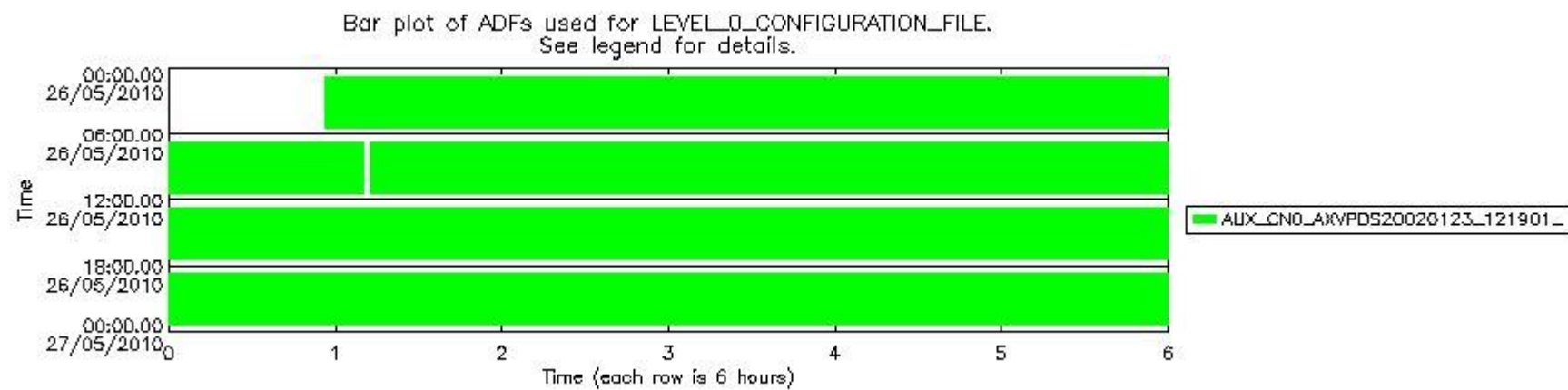
sciamachy_daily_report_level0_Any_version_20100526_7.PNG
