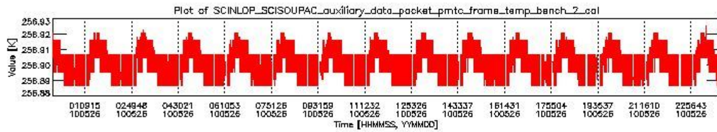
sciamachy_daily_report_level0_Any_version_20100526_1.PNG
