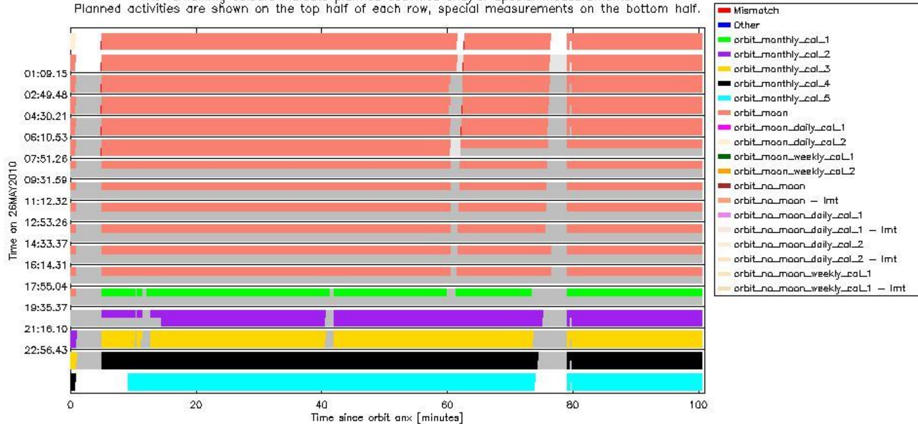
sciamachy_daily_report_level0_Any_version_20100526_6.PNG
