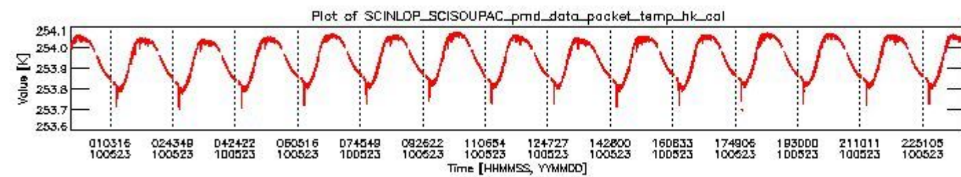
sciamachy_daily_report_level0_Any_version_20100523_3.PNG
