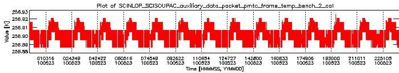
sciamachy_daily_report_level0_Any_version_20100523_1.PNG
