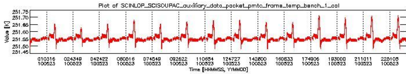
sciamachy_daily_report_level0_Any_version_20100523_0.PNG
