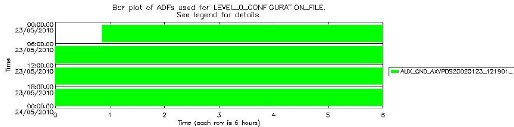
sciamachy_daily_report_level0_Any_version_20100523_7.PNG
