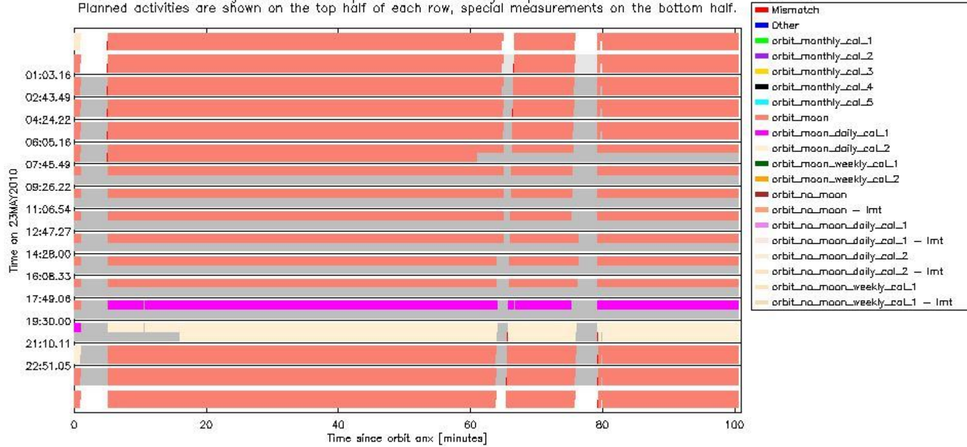
sciamachy_daily_report_level0_Any_version_20100523_6.PNG
