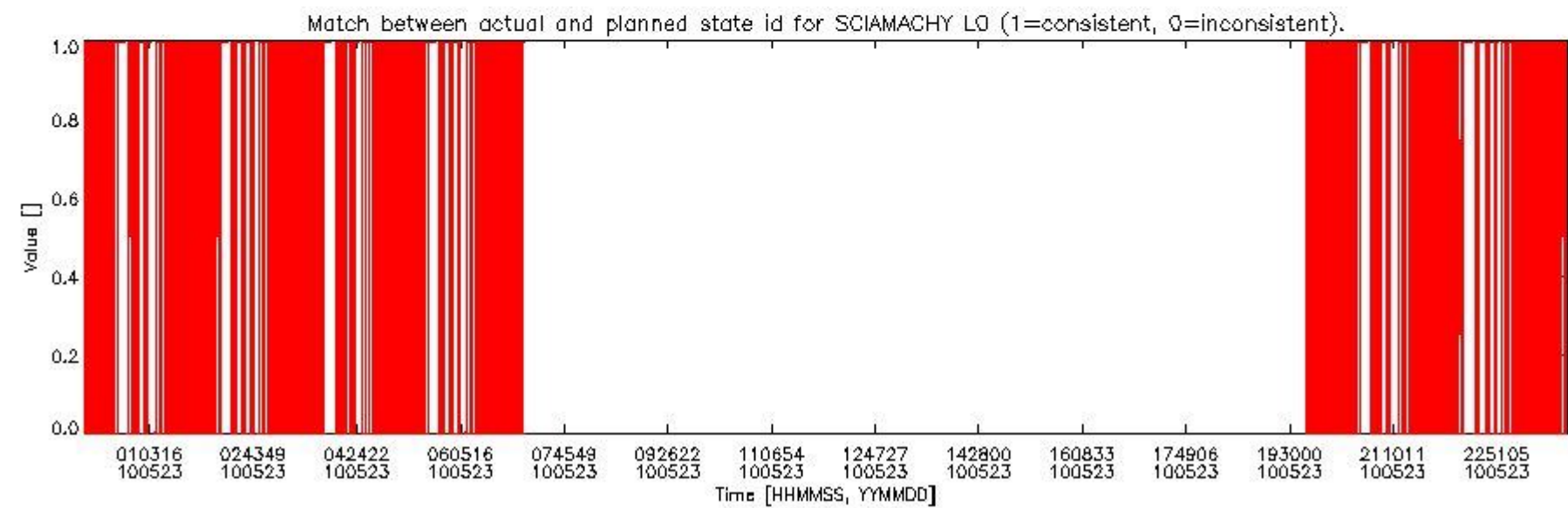
sciamachy_daily_report_level0_Any_version_20100523_5.PNG
