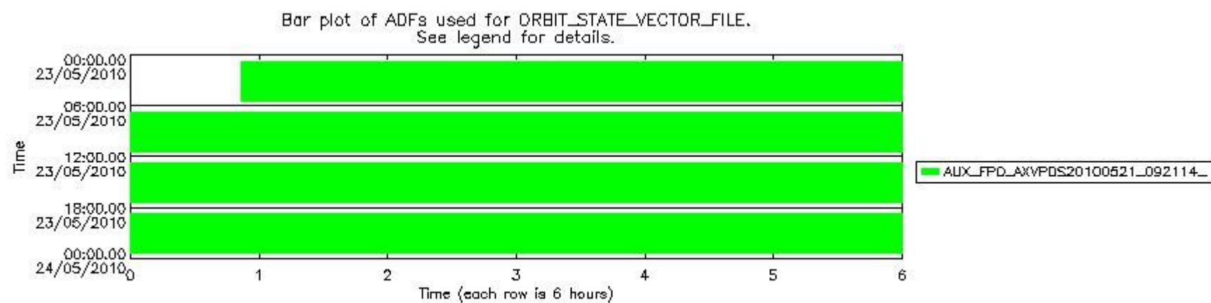
sciamachy_daily_report_level0_Any_version_20100523_8.PNG
