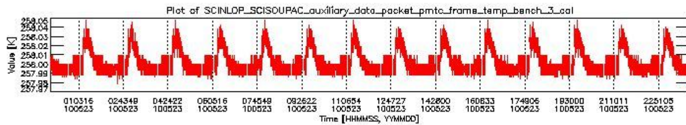
sciamachy_daily_report_level0_Any_version_20100523_2.PNG
