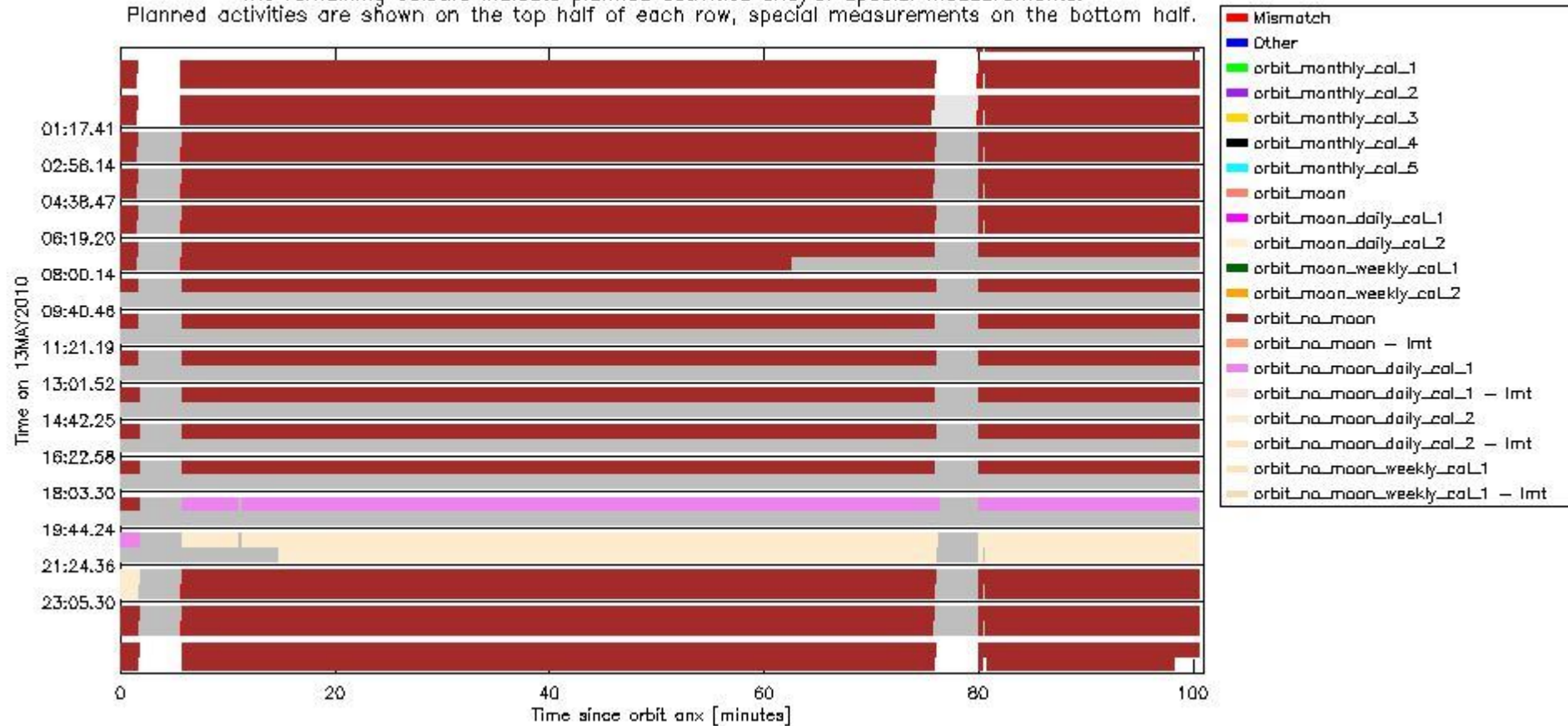
sciamachy_daily_report_level0_Any_version_20100513_6.PNG
