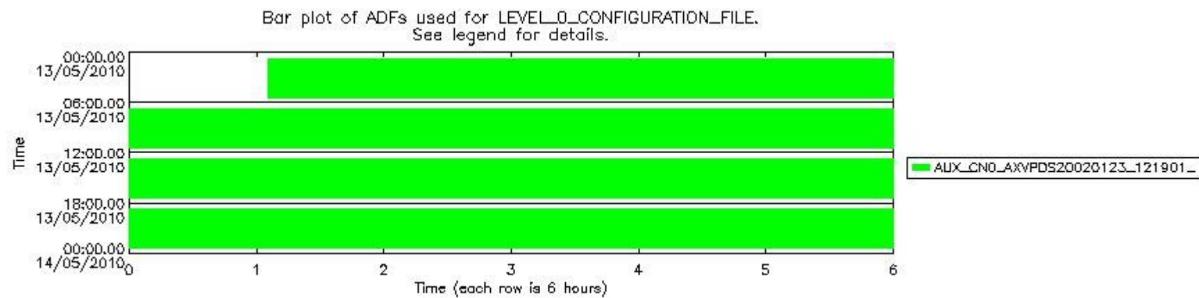
sciamachy_daily_report_level0_Any_version_20100513_7.PNG
