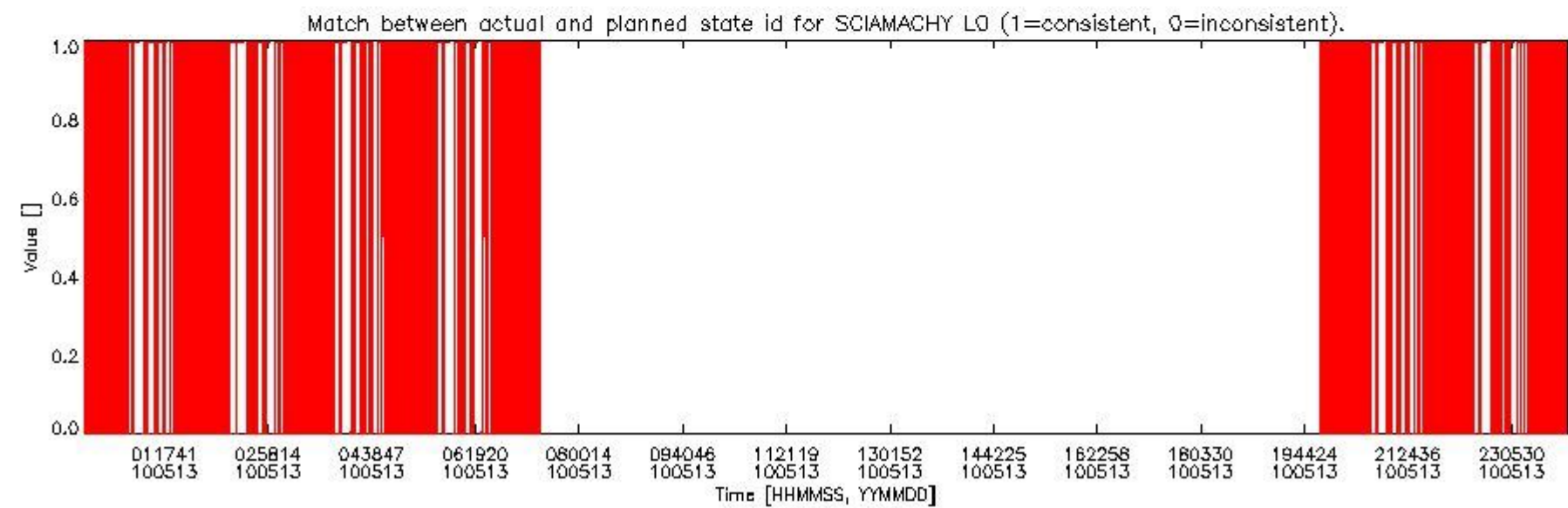
sciamachy_daily_report_level0_Any_version_20100513_5.PNG
