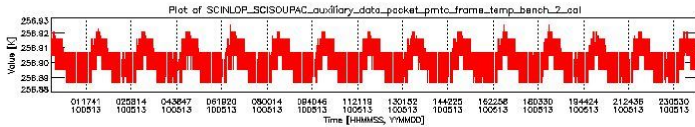
sciamachy_daily_report_level0_Any_version_20100513_1.PNG
