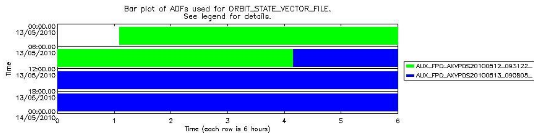
sciamachy_daily_report_level0_Any_version_20100513_8.PNG
