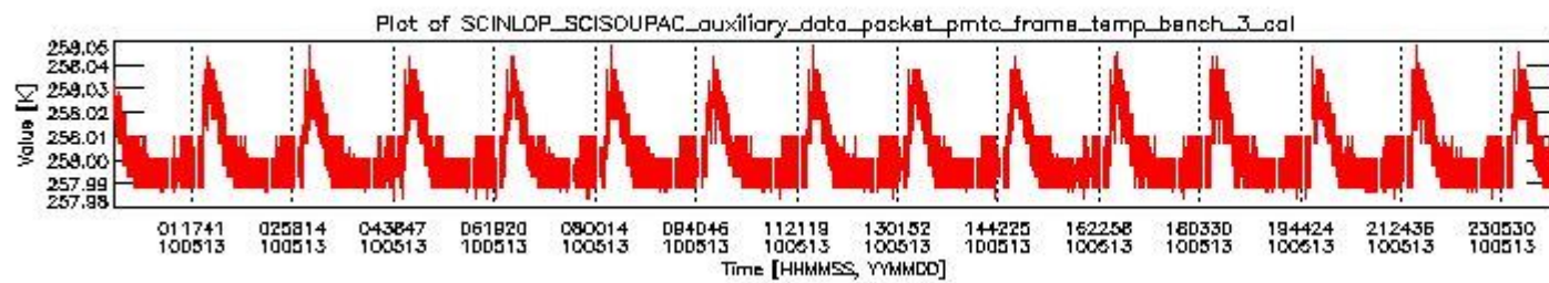
sciamachy_daily_report_level0_Any_version_20100513_2.PNG
