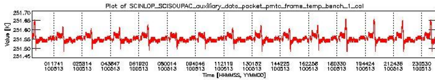
sciamachy_daily_report_level0_Any_version_20100513_0.PNG
