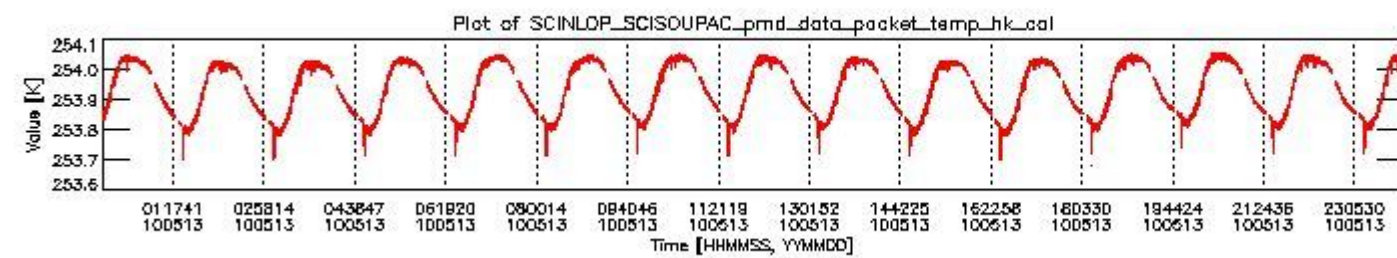
sciamachy_daily_report_level0_Any_version_20100513_3.PNG
