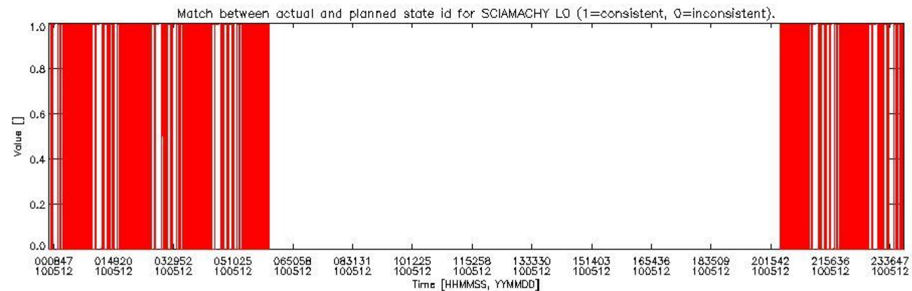
sciamachy_daily_report_level0_Any_version_20100512_5.PNG
