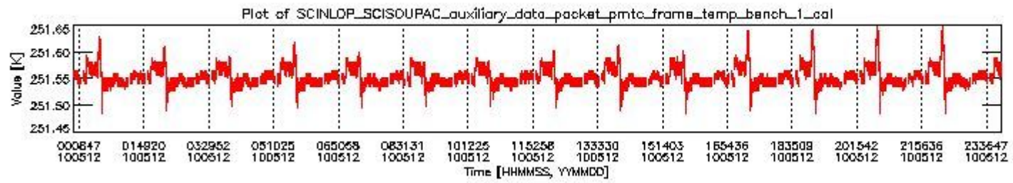
sciamachy_daily_report_level0_Any_version_20100512_0.PNG
