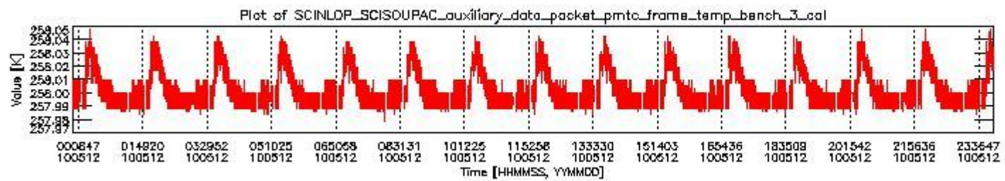
sciamachy_daily_report_level0_Any_version_20100512_2.PNG
