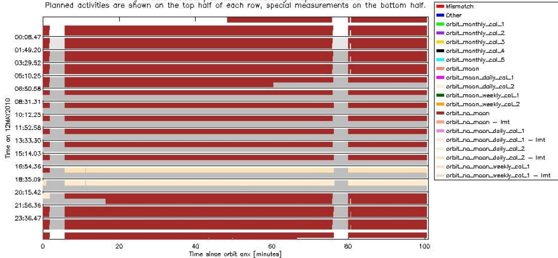
sciamachy_daily_report_level0_Any_version_20100512_6.PNG
