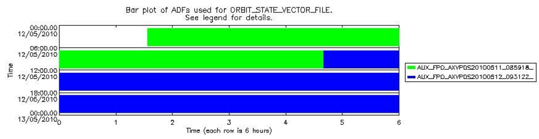
sciamachy_daily_report_level0_Any_version_20100512_8.PNG
