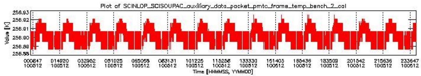
sciamachy_daily_report_level0_Any_version_20100512_1.PNG
