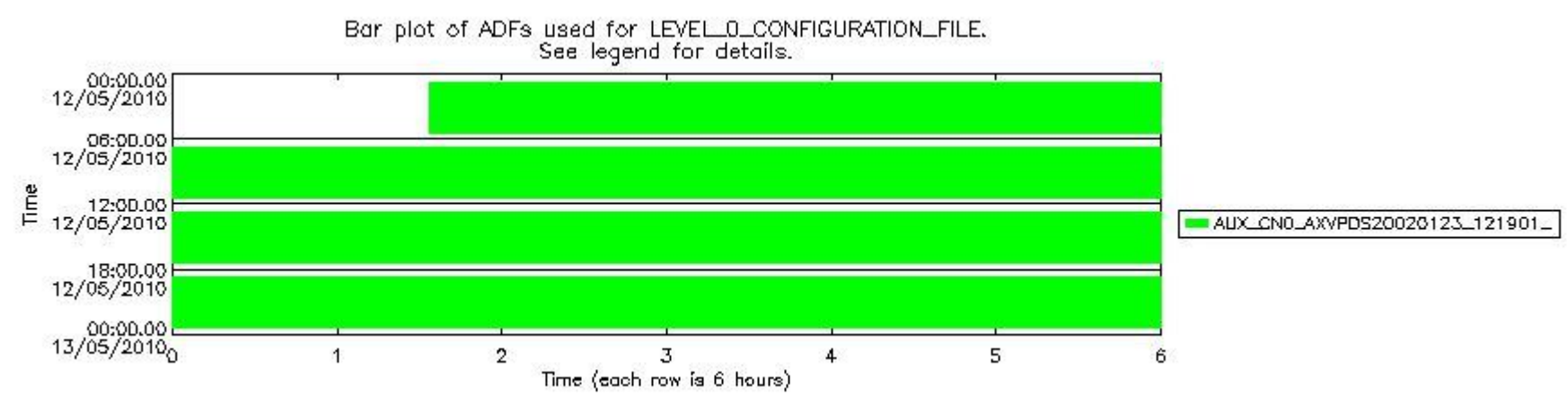
sciamachy_daily_report_level0_Any_version_20100512_7.PNG
