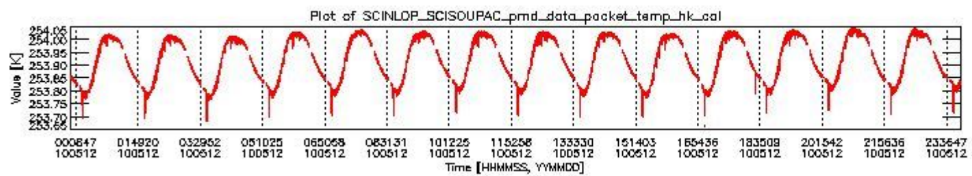
sciamachy_daily_report_level0_Any_version_20100512_3.PNG
