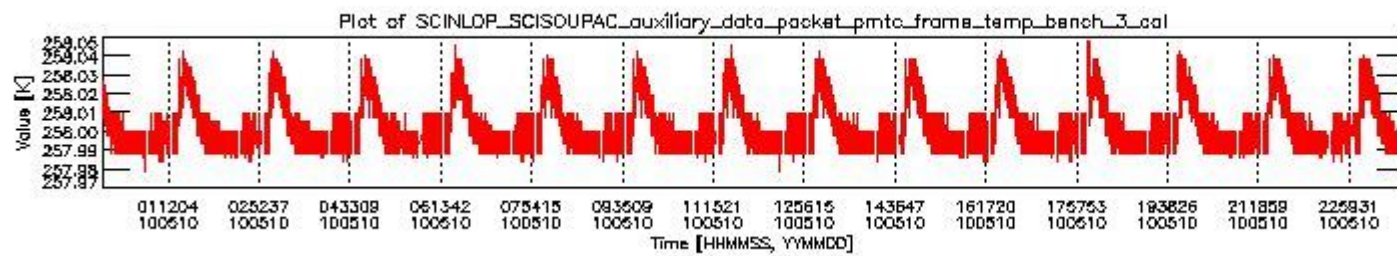
sciamachy_daily_report_level0_Any_version_20100510_2.PNG
