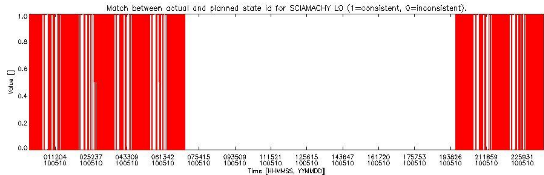
sciamachy_daily_report_level0_Any_version_20100510_5.PNG
