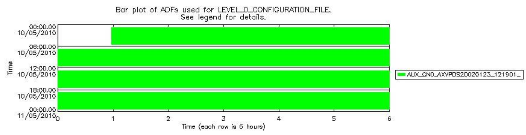
sciamachy_daily_report_level0_Any_version_20100510_7.PNG
