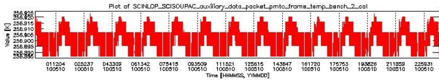
sciamachy_daily_report_level0_Any_version_20100510_1.PNG
