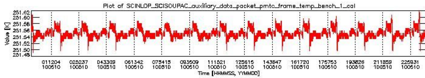
sciamachy_daily_report_level0_Any_version_20100510_0.PNG
