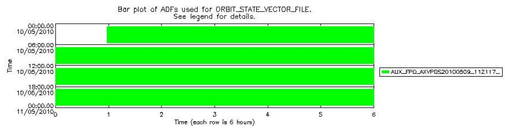
sciamachy_daily_report_level0_Any_version_20100510_8.PNG
