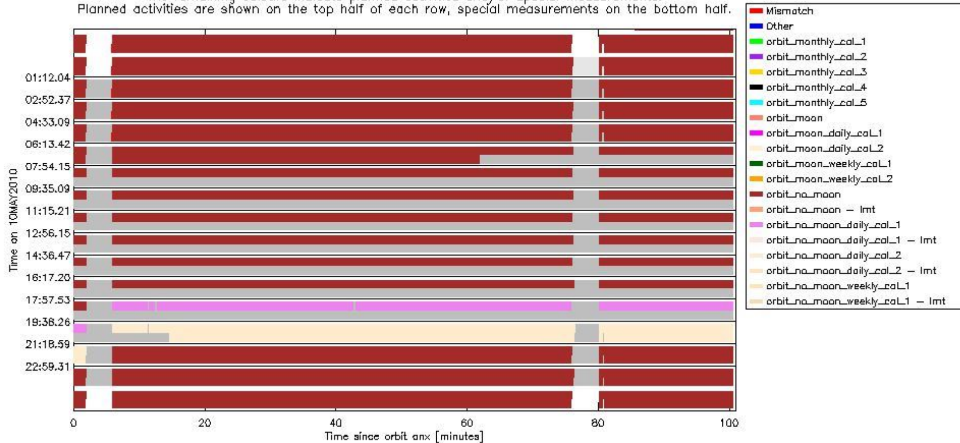
sciamachy_daily_report_level0_Any_version_20100510_6.PNG
