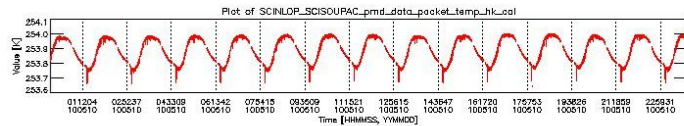
sciamachy_daily_report_level0_Any_version_20100510_3.PNG
