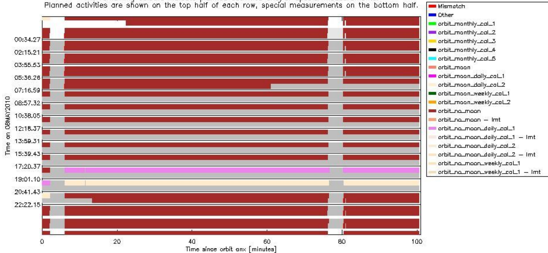
sciamachy_daily_report_level0_Any_version_20100508_6.PNG
