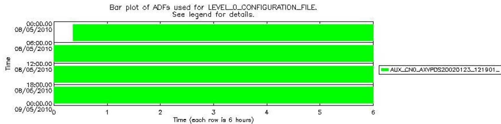
sciamachy_daily_report_level0_Any_version_20100508_7.PNG
