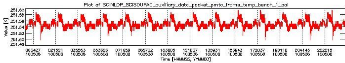
sciamachy_daily_report_level0_Any_version_20100508_0.PNG
