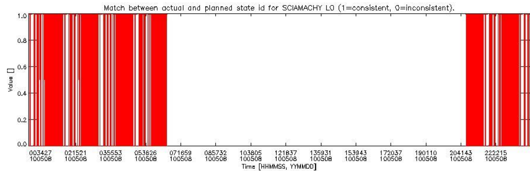
sciamachy_daily_report_level0_Any_version_20100508_5.PNG
