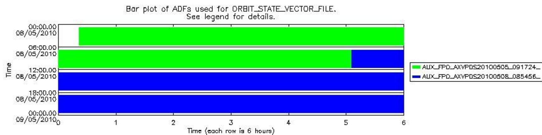
sciamachy_daily_report_level0_Any_version_20100508_8.PNG
