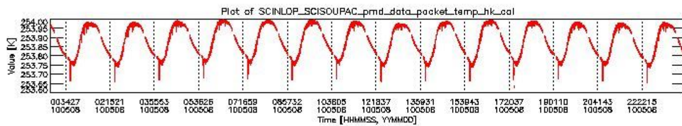
sciamachy_daily_report_level0_Any_version_20100508_3.PNG
