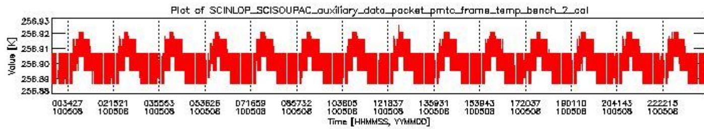
sciamachy_daily_report_level0_Any_version_20100508_1.PNG
