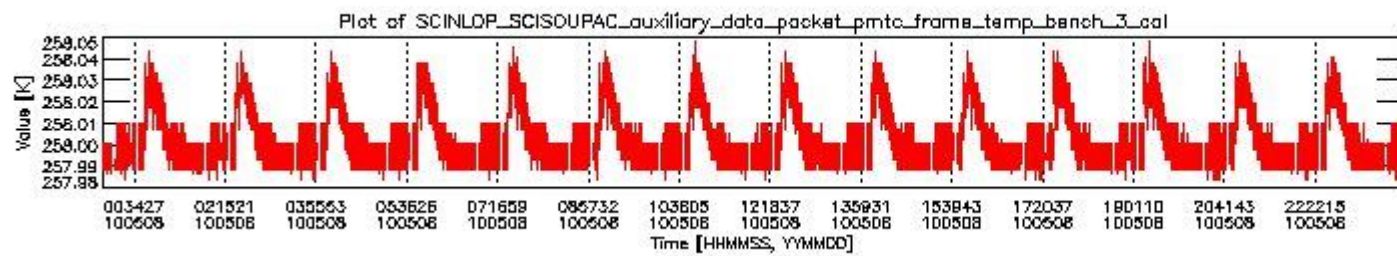
sciamachy_daily_report_level0_Any_version_20100508_2.PNG
