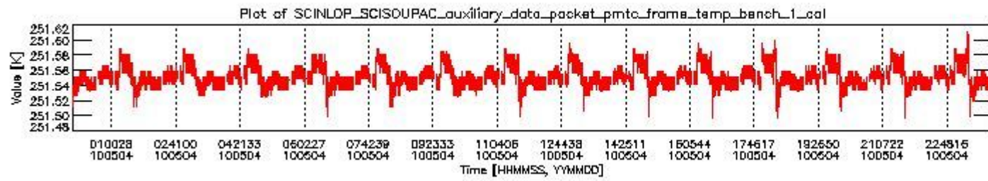
sciamachy_daily_report_level0_Any_version_20100504_0.PNG
