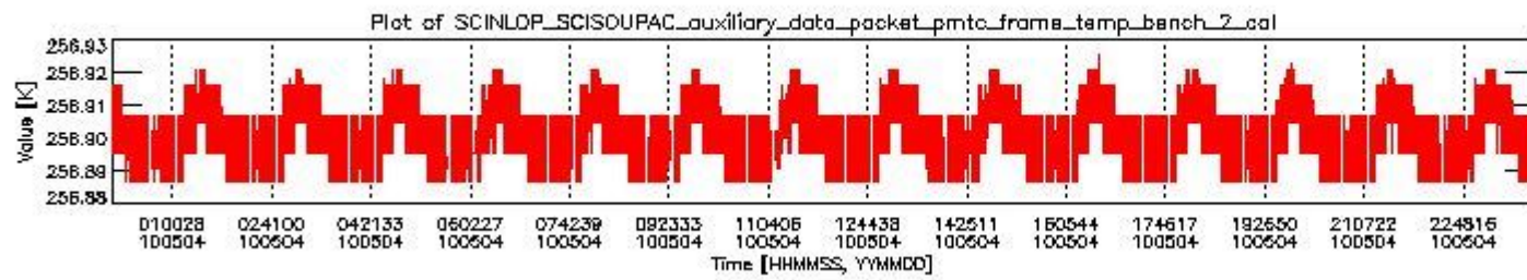
sciamachy_daily_report_level0_Any_version_20100504_1.PNG
