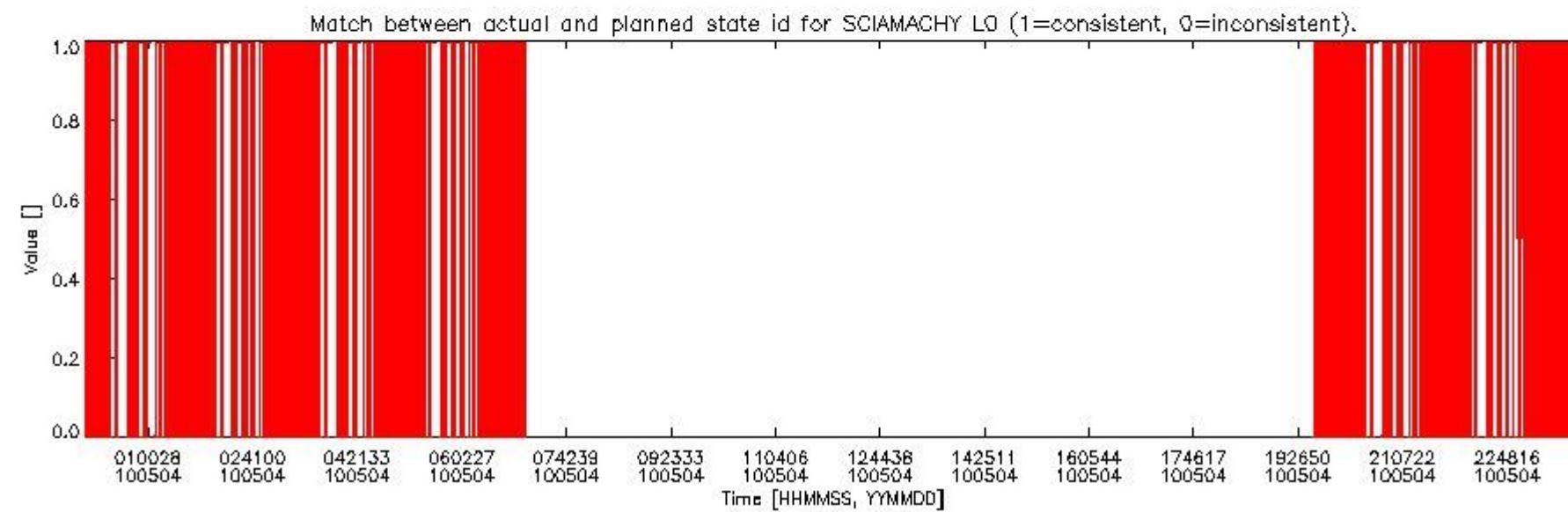
sciamachy_daily_report_level0_Any_version_20100504_5.PNG
