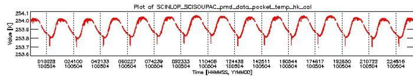
sciamachy_daily_report_level0_Any_version_20100504_3.PNG
