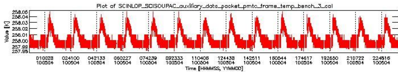
sciamachy_daily_report_level0_Any_version_20100504_2.PNG
