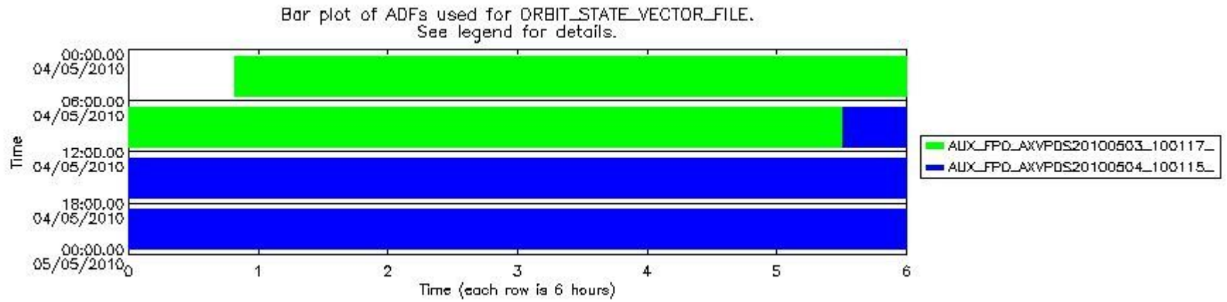
sciamachy_daily_report_level0_Any_version_20100504_8.PNG
