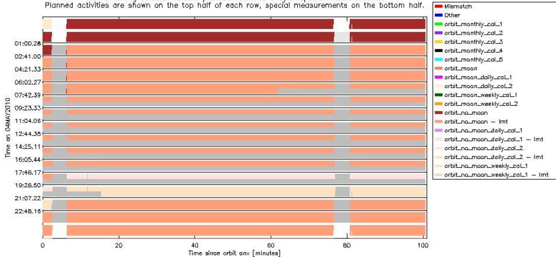
sciamachy_daily_report_level0_Any_version_20100504_6.PNG
