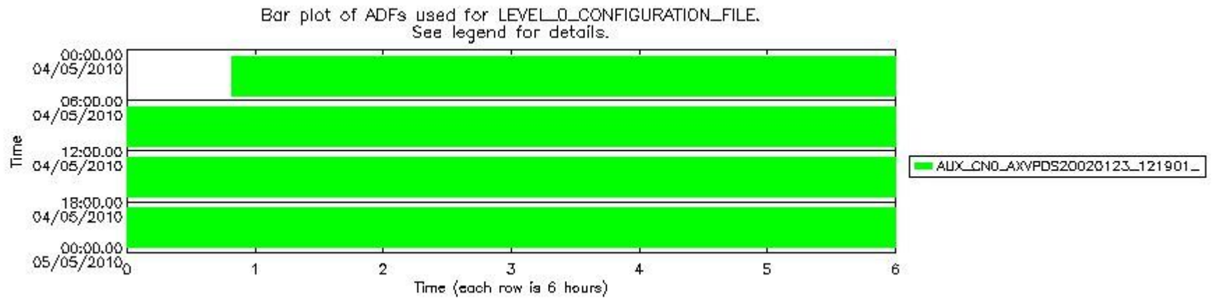
sciamachy_daily_report_level0_Any_version_20100504_7.PNG
