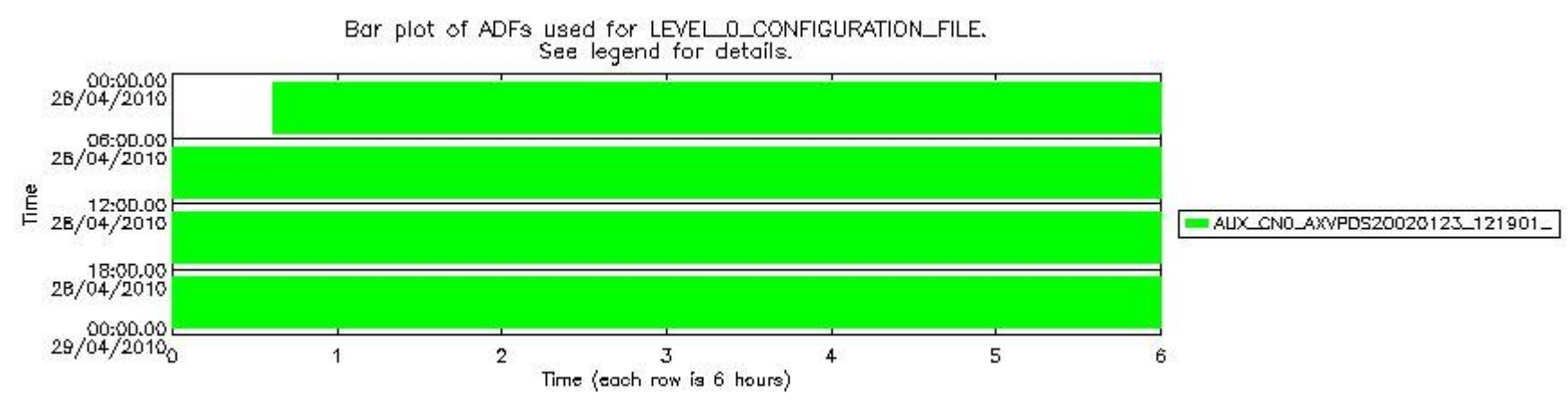
sciamachy_daily_report_level0_Any_version_20100428_7.PNG
