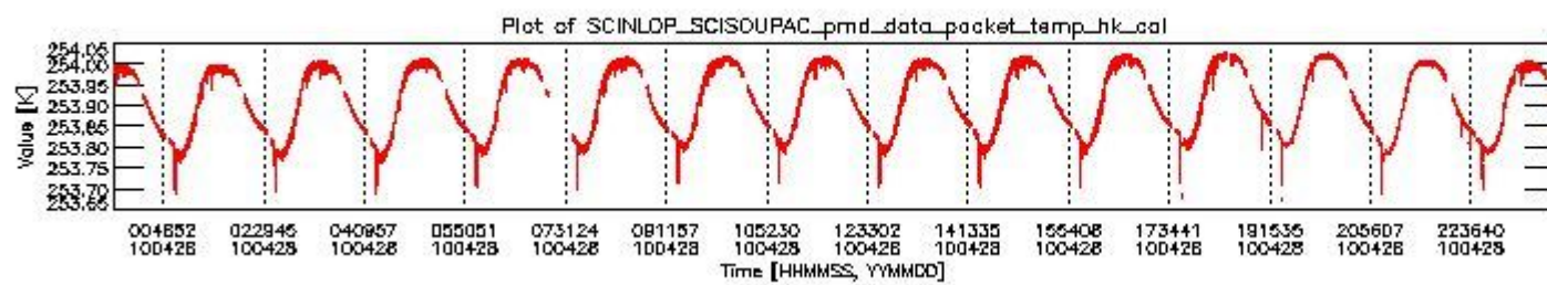
sciamachy_daily_report_level0_Any_version_20100428_3.PNG
