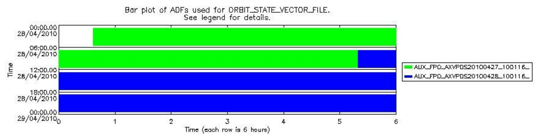
sciamachy_daily_report_level0_Any_version_20100428_8.PNG
