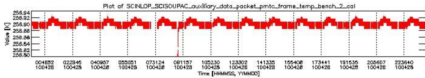
sciamachy_daily_report_level0_Any_version_20100428_1.PNG
