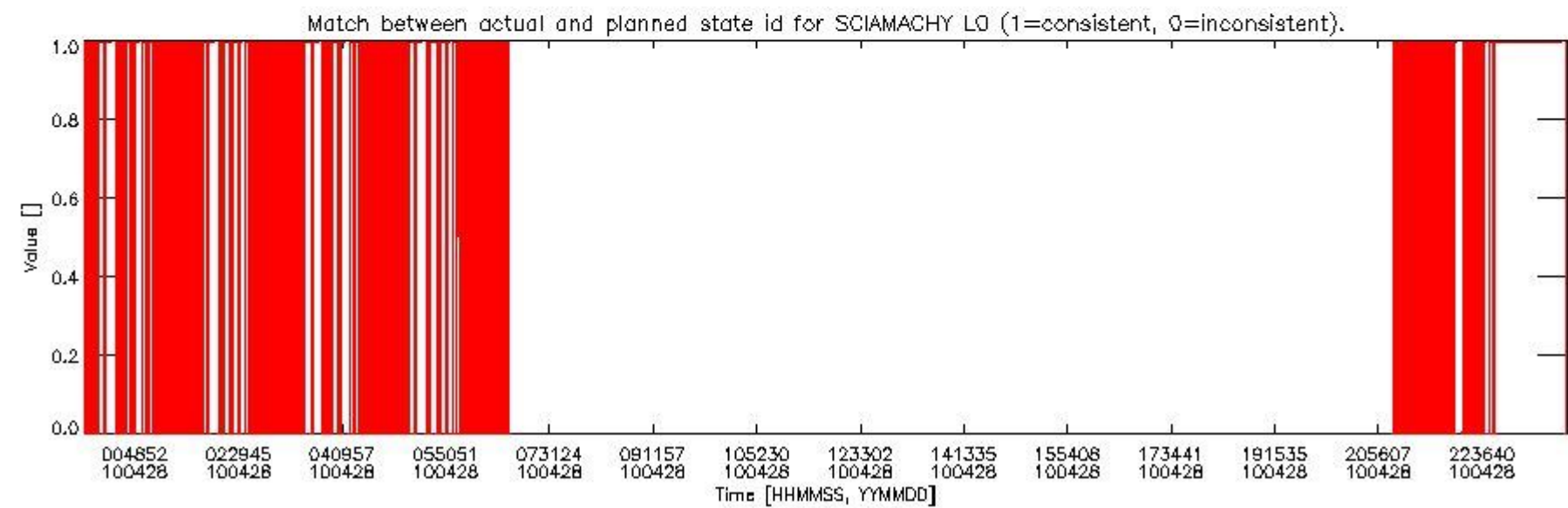
sciamachy_daily_report_level0_Any_version_20100428_5.PNG
