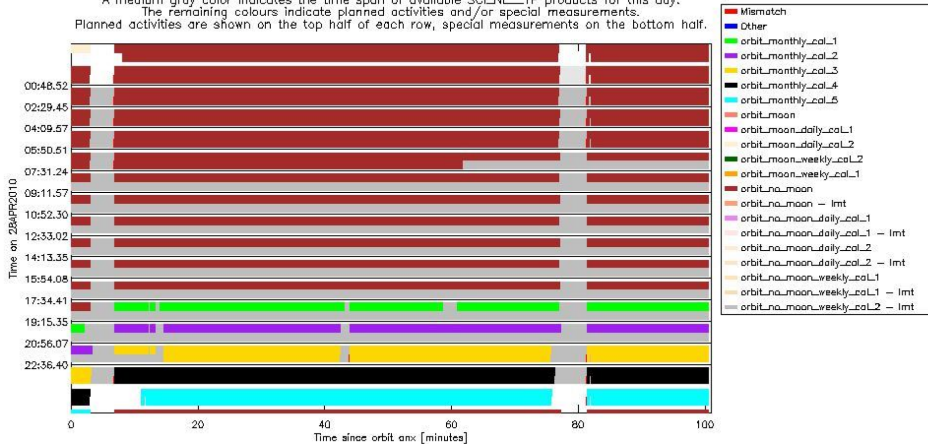
sciamachy_daily_report_level0_Any_version_20100428_6.PNG
