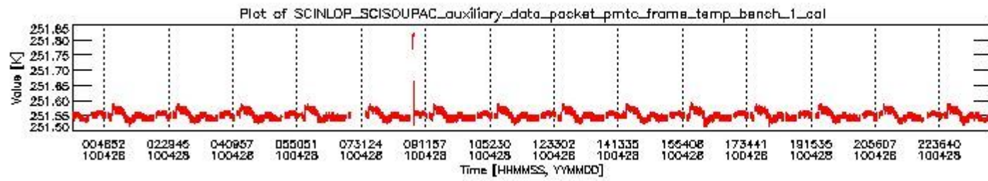
sciamachy_daily_report_level0_Any_version_20100428_0.PNG
