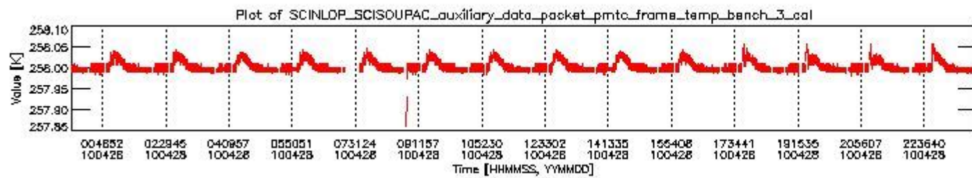
sciamachy_daily_report_level0_Any_version_20100428_2.PNG
