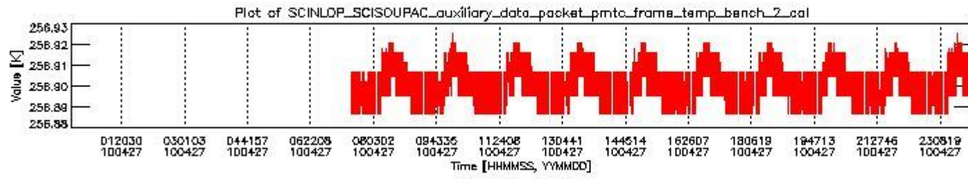
sciamachy_daily_report_level0_Any_version_20100427_1.PNG
