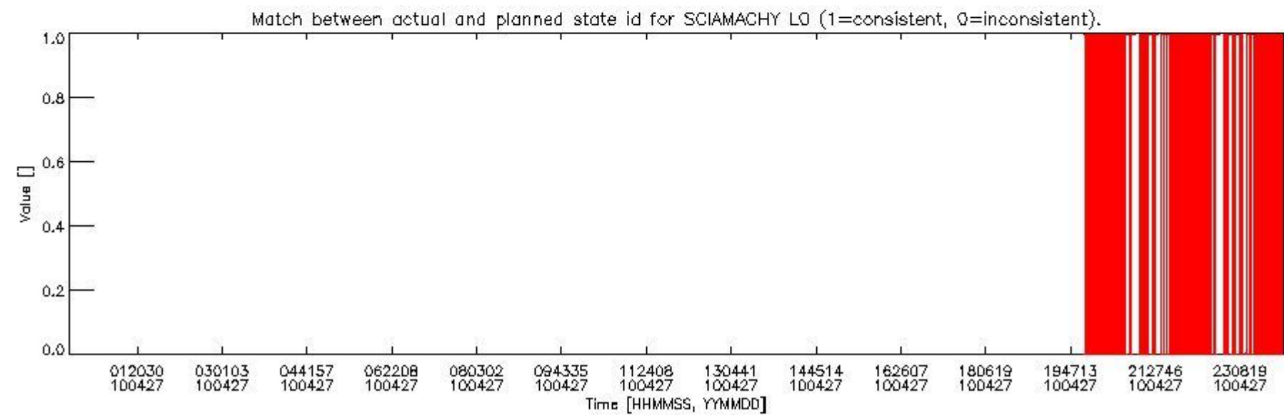
sciamachy_daily_report_level0_Any_version_20100427_5.PNG
