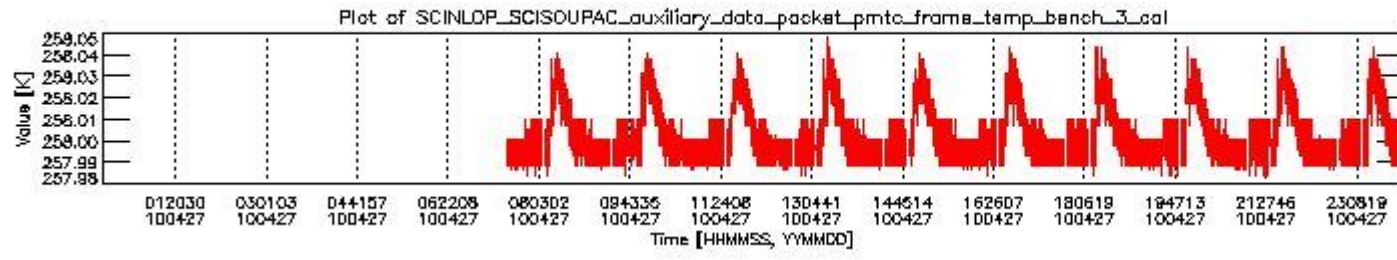
sciamachy_daily_report_level0_Any_version_20100427_2.PNG
