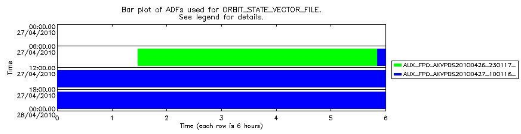
sciamachy_daily_report_level0_Any_version_20100427_8.PNG
