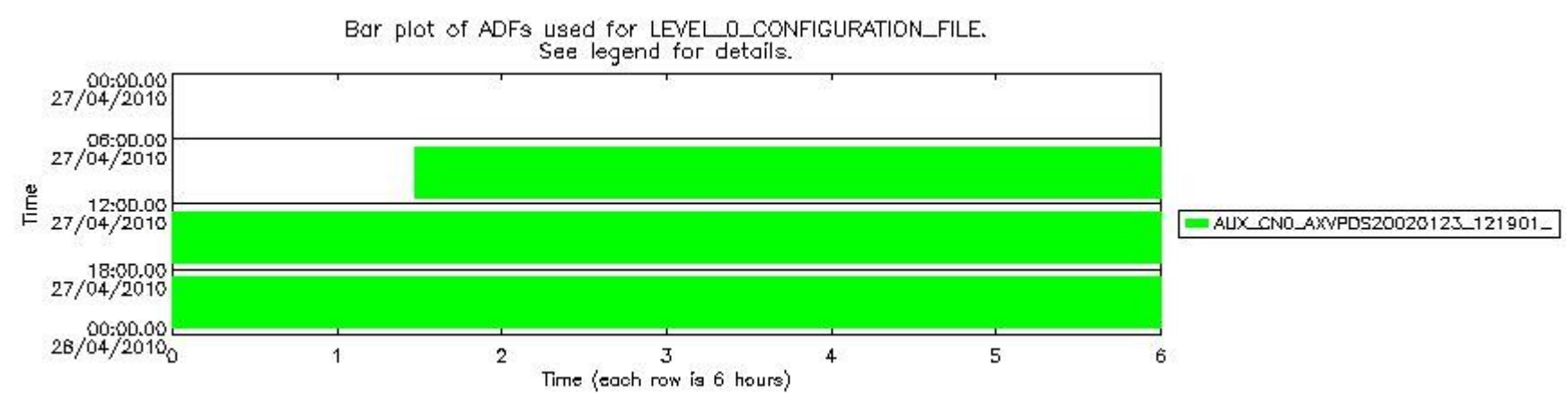
sciamachy_daily_report_level0_Any_version_20100427_7.PNG
