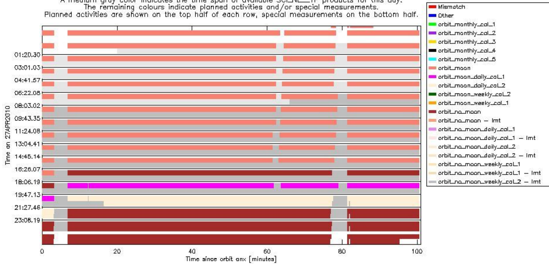
sciamachy_daily_report_level0_Any_version_20100427_6.PNG
