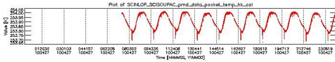
sciamachy_daily_report_level0_Any_version_20100427_3.PNG
