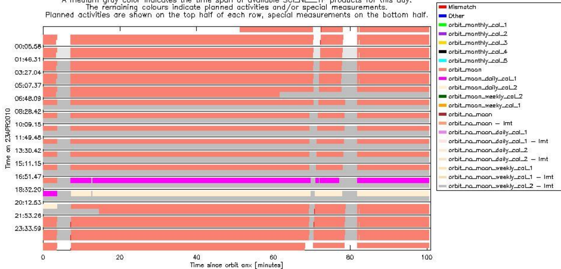
sciamachy_daily_report_level0_Any_version_20100423_6.PNG
