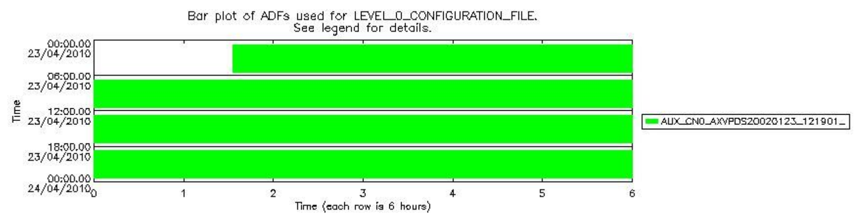
sciamachy_daily_report_level0_Any_version_20100423_7.PNG
