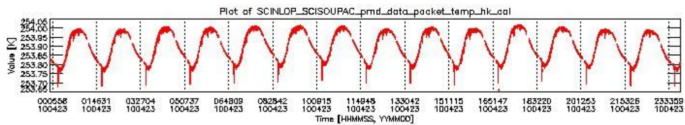
sciamachy_daily_report_level0_Any_version_20100423_3.PNG
