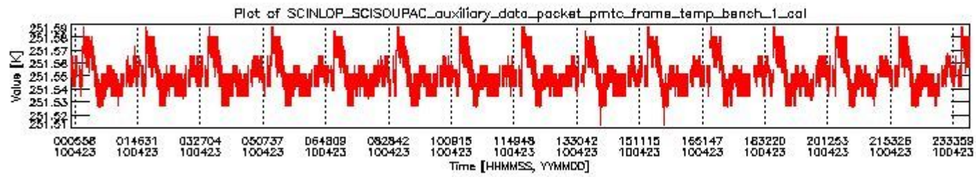
sciamachy_daily_report_level0_Any_version_20100423_0.PNG
