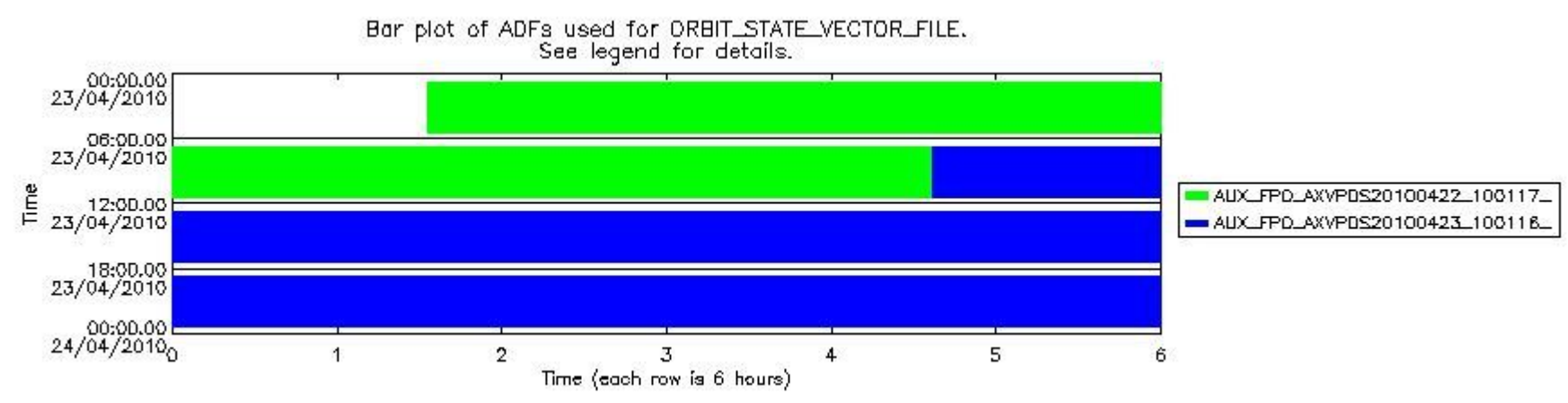
sciamachy_daily_report_level0_Any_version_20100423_8.PNG
