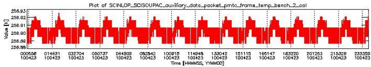
sciamachy_daily_report_level0_Any_version_20100423_1.PNG
