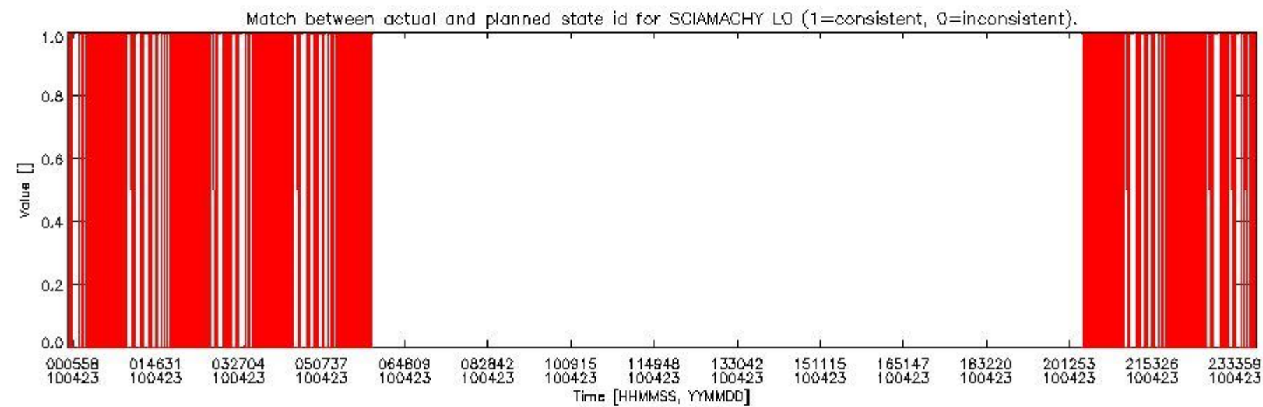
sciamachy_daily_report_level0_Any_version_20100423_5.PNG
