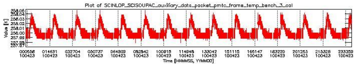
sciamachy_daily_report_level0_Any_version_20100423_2.PNG
