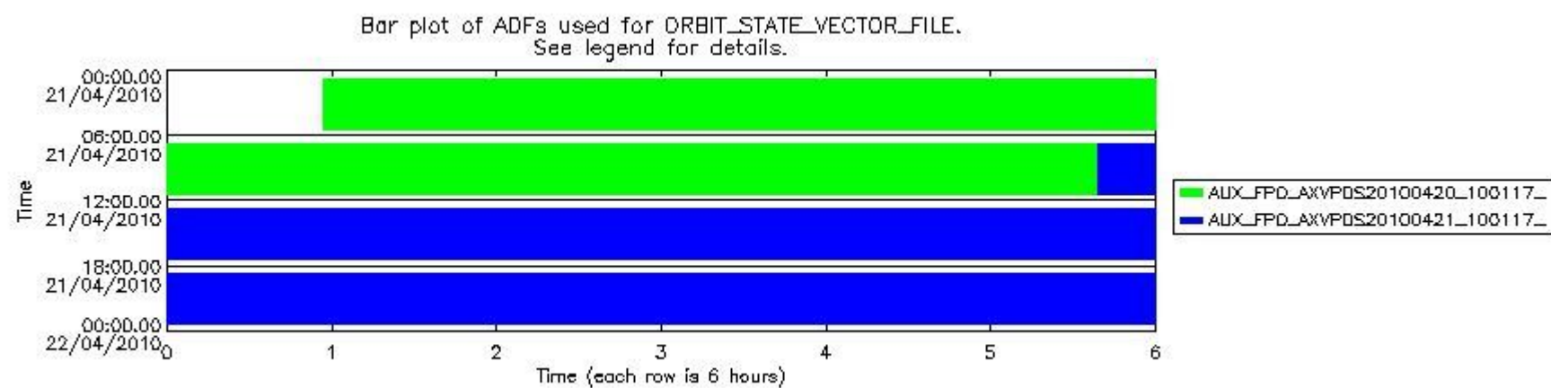
sciamachy_daily_report_level0_Any_version_20100421_8.PNG
