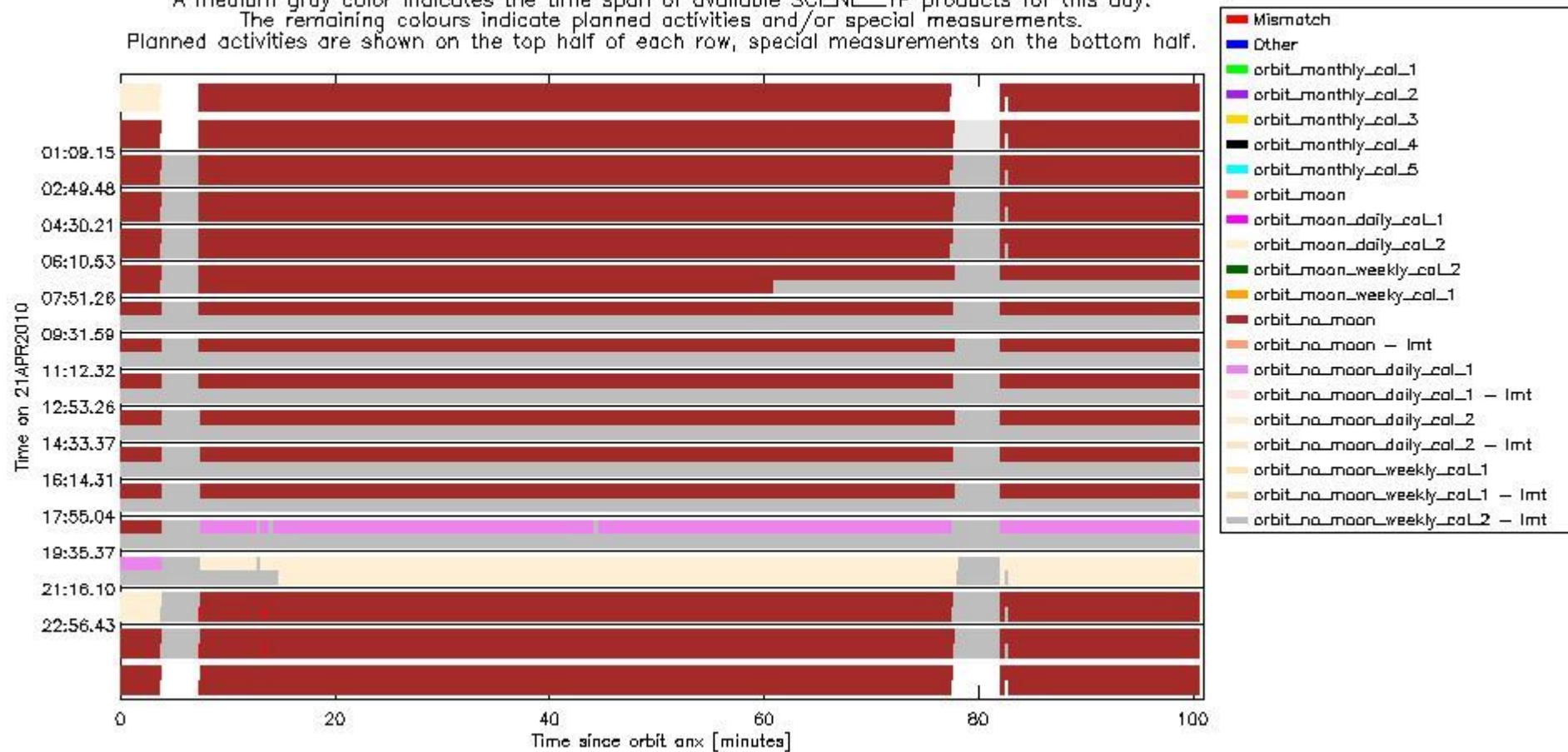
sciamachy_daily_report_level0_Any_version_20100421_6.PNG
