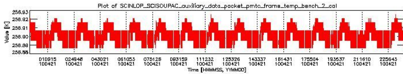
sciamachy_daily_report_level0_Any_version_20100421_1.PNG
