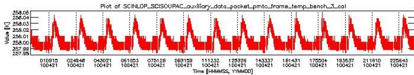
sciamachy_daily_report_level0_Any_version_20100421_2.PNG
