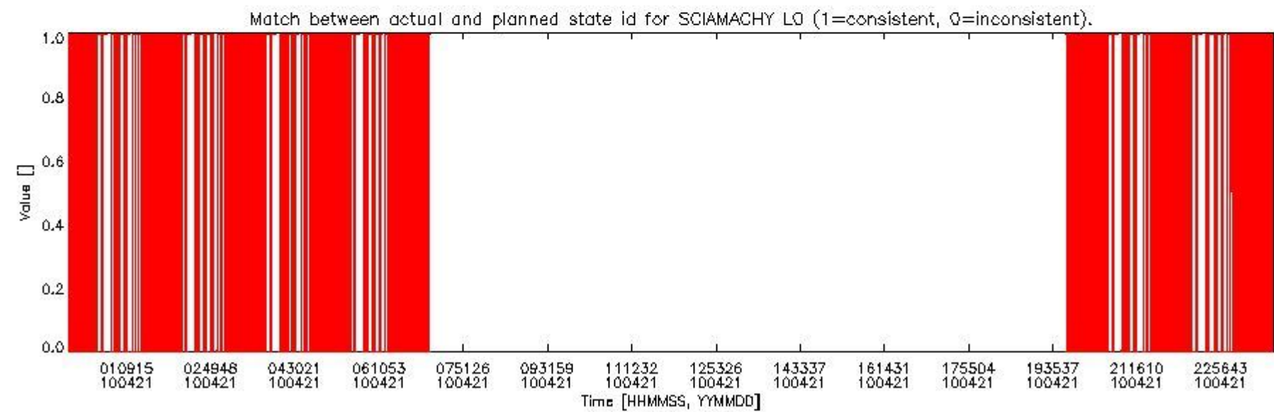
sciamachy_daily_report_level0_Any_version_20100421_5.PNG
