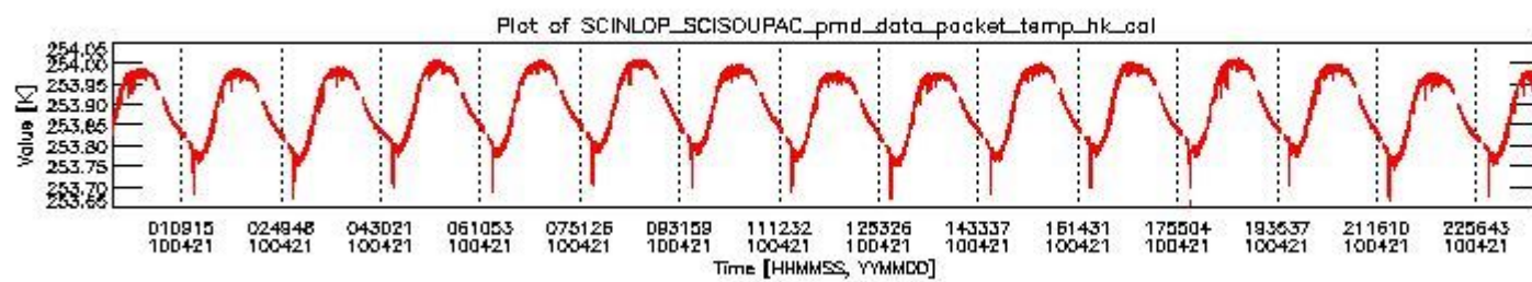
sciamachy_daily_report_level0_Any_version_20100421_3.PNG
