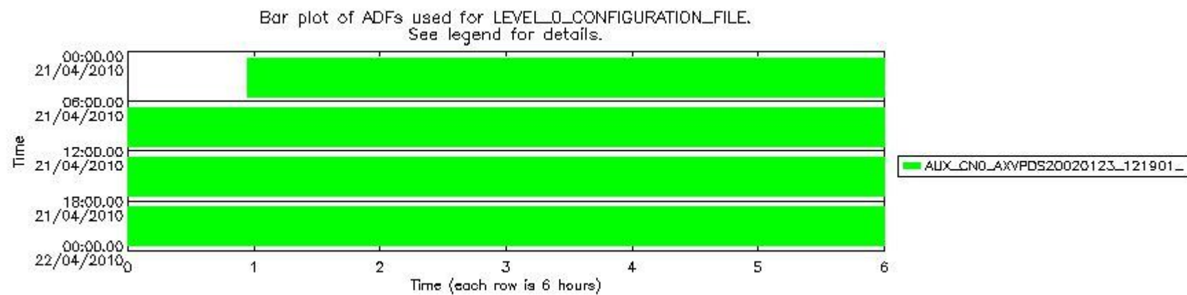
sciamachy_daily_report_level0_Any_version_20100421_7.PNG
