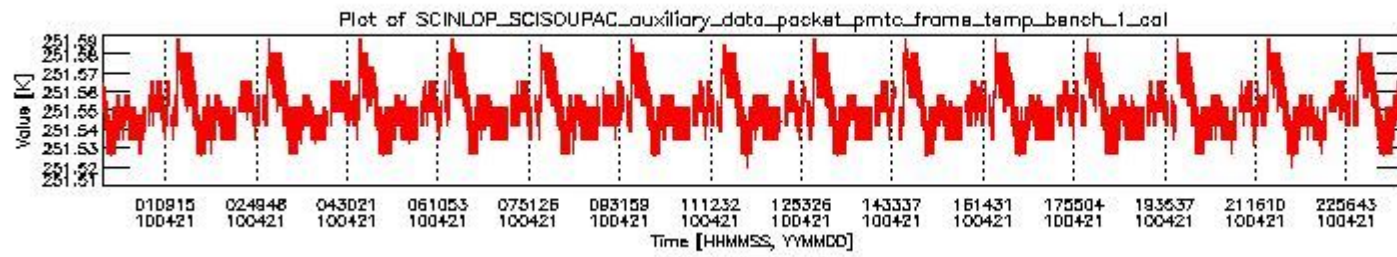
sciamachy_daily_report_level0_Any_version_20100421_0.PNG
