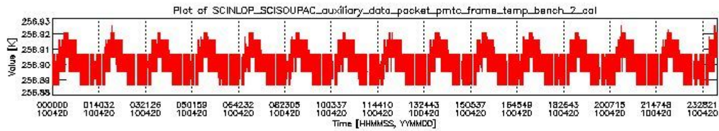
sciamachy_daily_report_level0_Any_version_20100420_1.PNG
