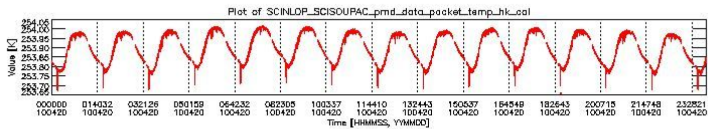
sciamachy_daily_report_level0_Any_version_20100420_3.PNG
