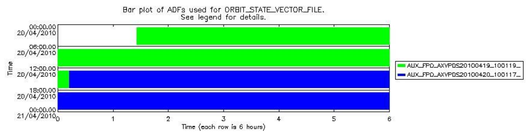
sciamachy_daily_report_level0_Any_version_20100420_8.PNG
