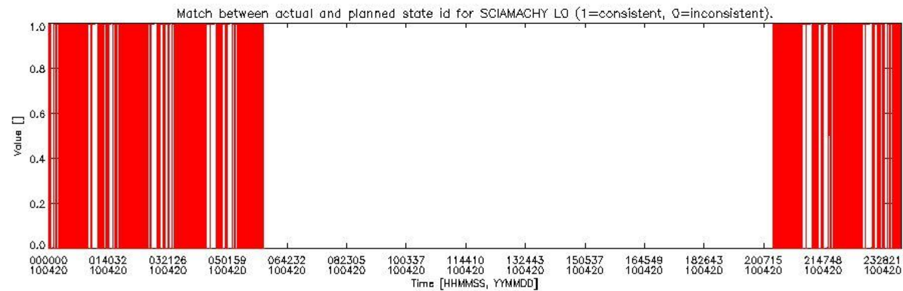
sciamachy_daily_report_level0_Any_version_20100420_5.PNG
