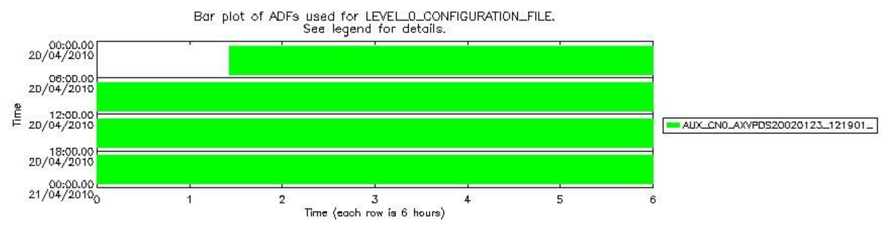
sciamachy_daily_report_level0_Any_version_20100420_7.PNG
