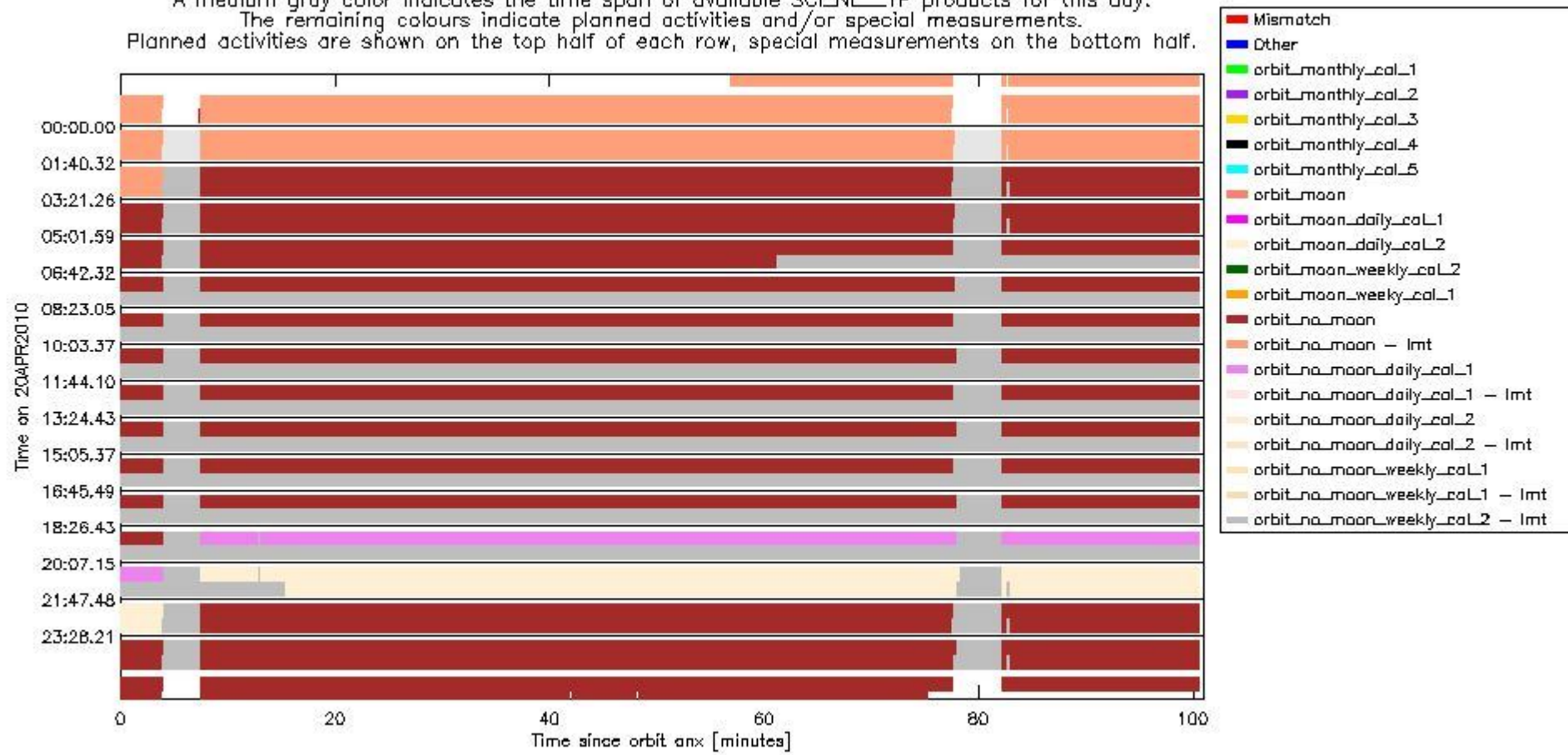
sciamachy_daily_report_level0_Any_version_20100420_6.PNG
