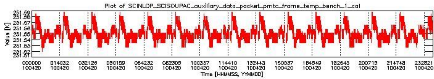
sciamachy_daily_report_level0_Any_version_20100420_0.PNG
