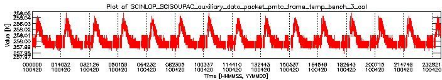
sciamachy_daily_report_level0_Any_version_20100420_2.PNG
