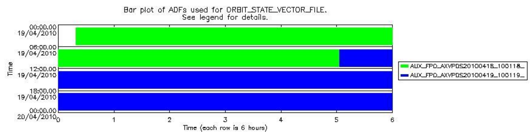
sciamachy_daily_report_level0_Any_version_20100419_8.PNG
