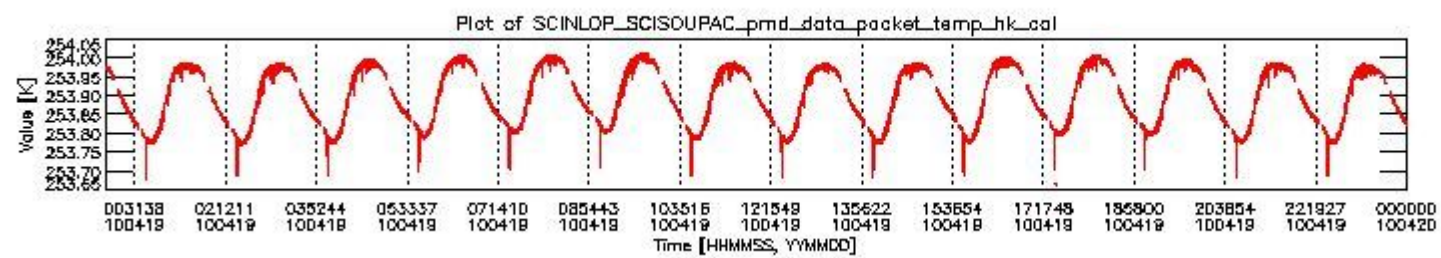
sciamachy_daily_report_level0_Any_version_20100419_3.PNG
