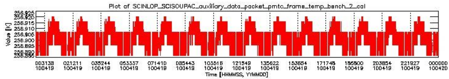
sciamachy_daily_report_level0_Any_version_20100419_1.PNG
