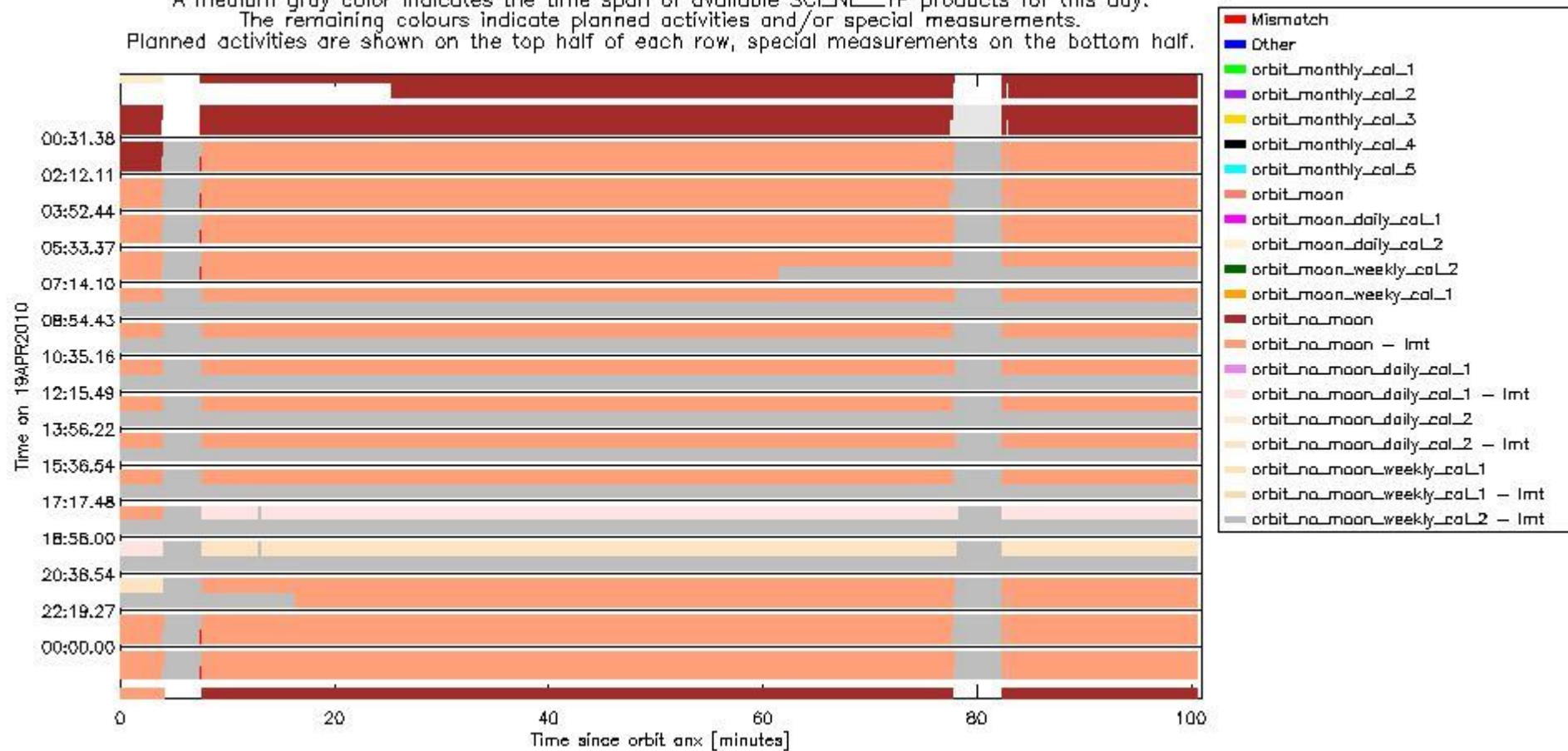
sciamachy_daily_report_level0_Any_version_20100419_6.PNG
