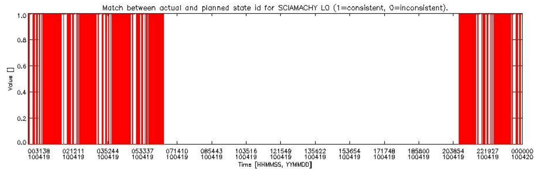
sciamachy_daily_report_level0_Any_version_20100419_5.PNG
