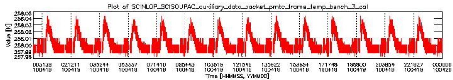
sciamachy_daily_report_level0_Any_version_20100419_2.PNG
