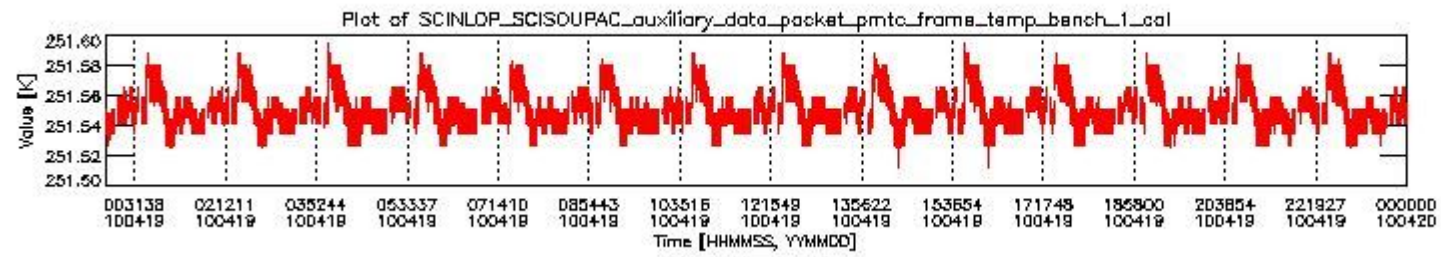
sciamachy_daily_report_level0_Any_version_20100419_0.PNG
