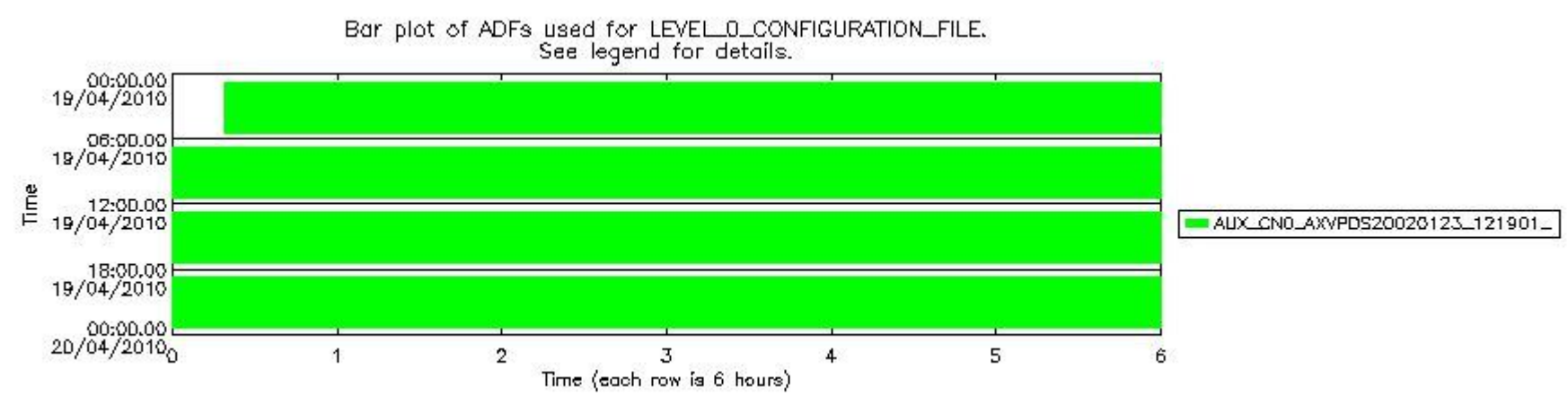
sciamachy_daily_report_level0_Any_version_20100419_7.PNG
