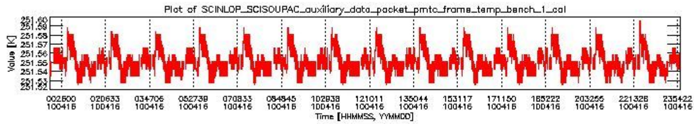
sciamachy_daily_report_level0_Any_version_20100416_0.PNG
