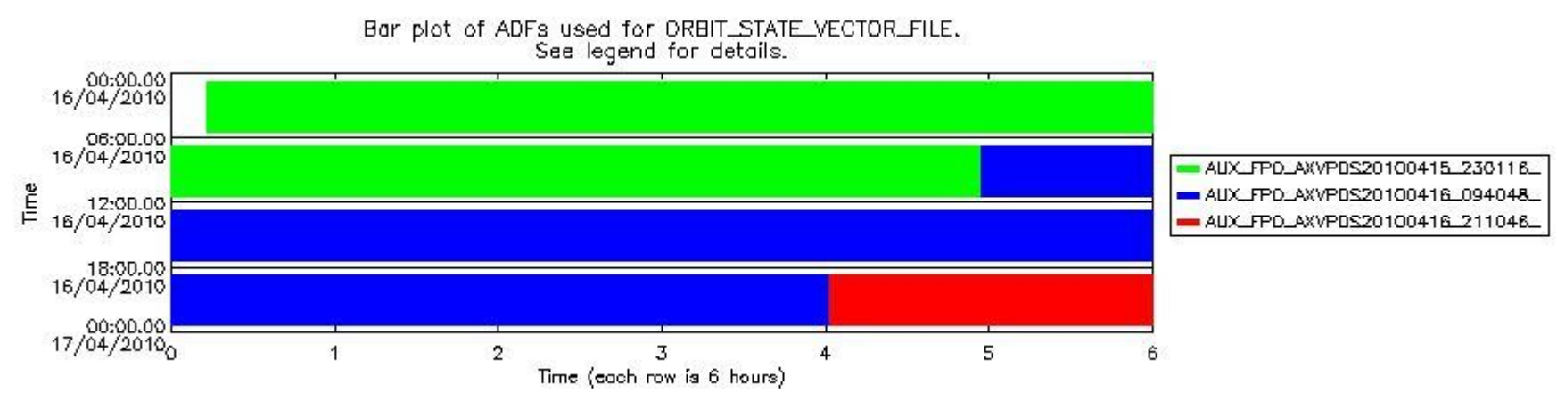
sciamachy_daily_report_level0_Any_version_20100416_8.PNG
