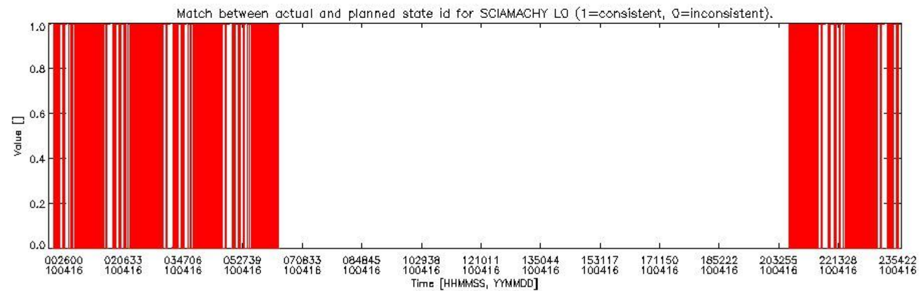
sciamachy_daily_report_level0_Any_version_20100416_5.PNG
