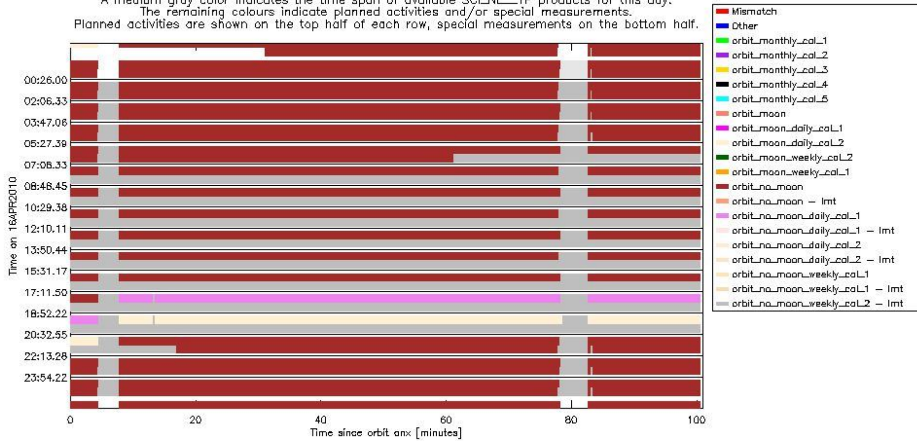
sciamachy_daily_report_level0_Any_version_20100416_6.PNG
