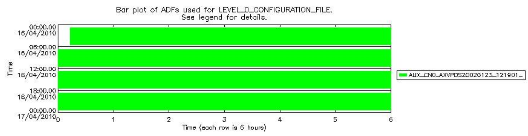
sciamachy_daily_report_level0_Any_version_20100416_7.PNG
