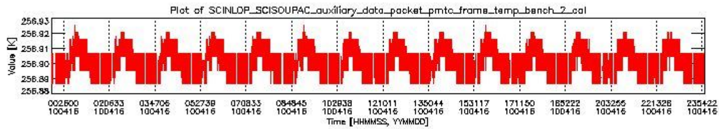
sciamachy_daily_report_level0_Any_version_20100416_1.PNG
