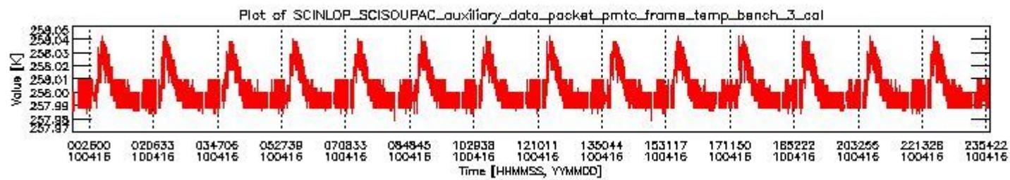
sciamachy_daily_report_level0_Any_version_20100416_2.PNG
