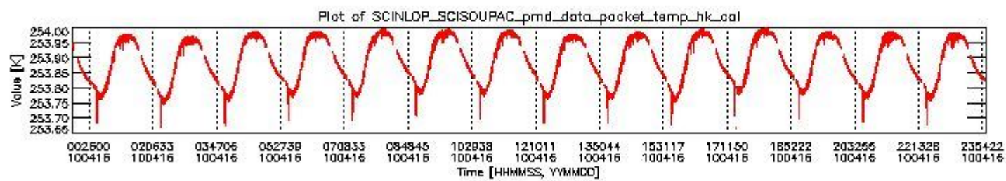
sciamachy_daily_report_level0_Any_version_20100416_3.PNG
