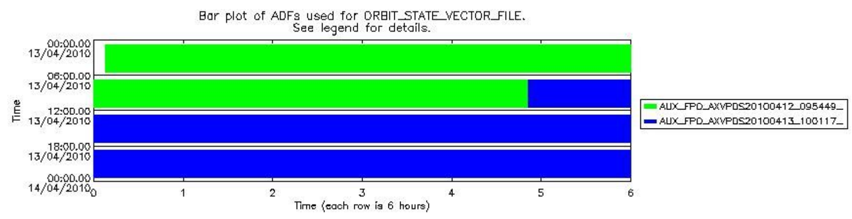
sciamachy_daily_report_level0_Any_version_20100413_8.PNG
