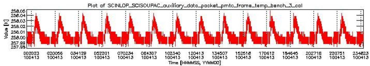
sciamachy_daily_report_level0_Any_version_20100413_2.PNG
