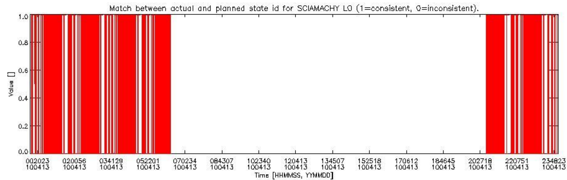
sciamachy_daily_report_level0_Any_version_20100413_5.PNG
