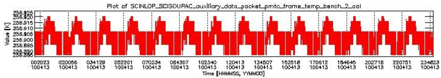
sciamachy_daily_report_level0_Any_version_20100413_1.PNG
