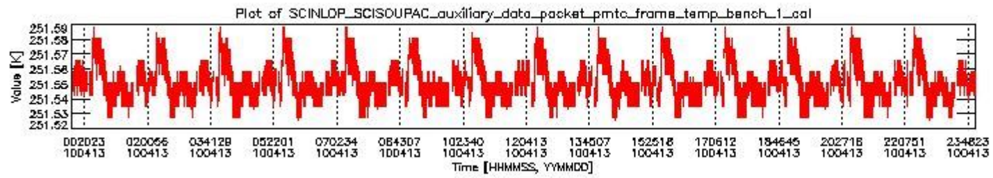
sciamachy_daily_report_level0_Any_version_20100413_0.PNG
