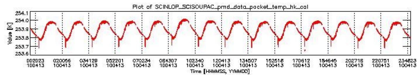
sciamachy_daily_report_level0_Any_version_20100413_3.PNG
