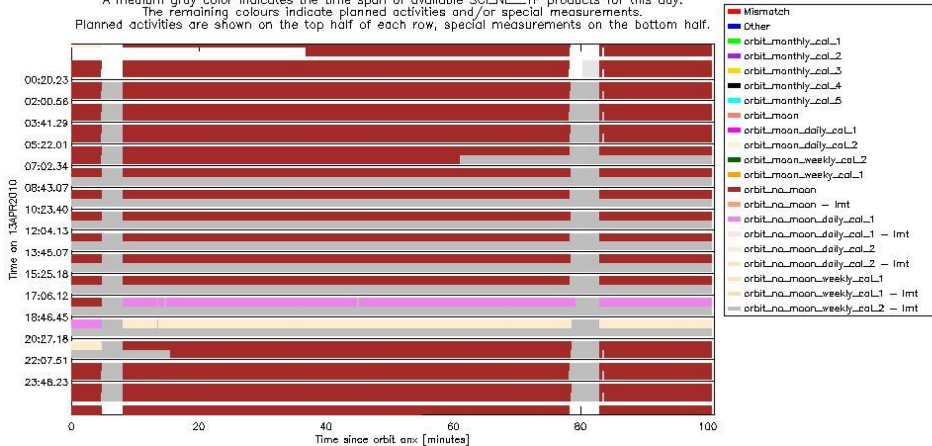
sciamachy_daily_report_level0_Any_version_20100413_6.PNG
