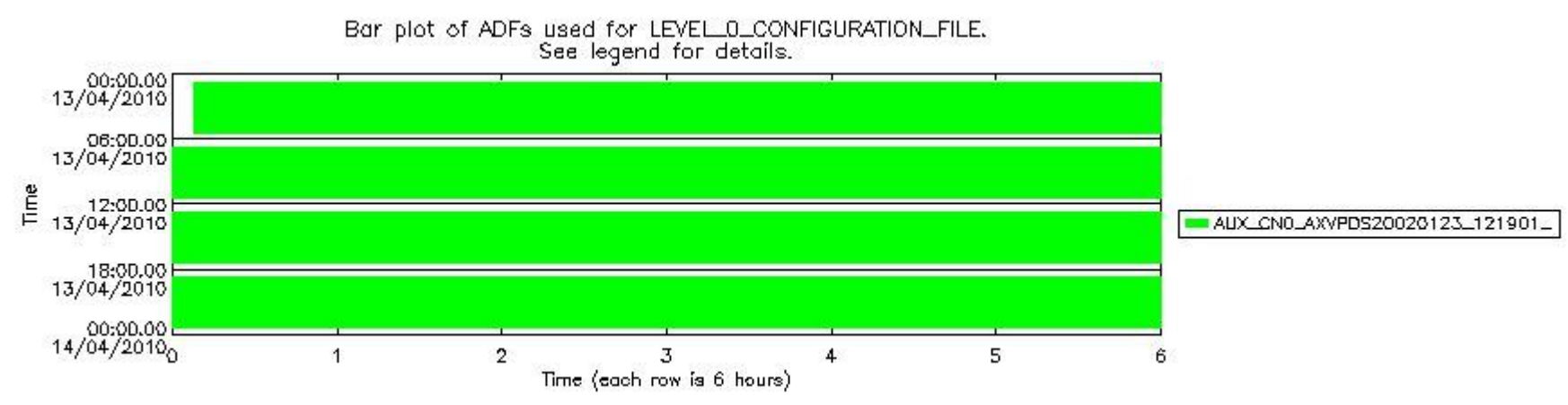
sciamachy_daily_report_level0_Any_version_20100413_7.PNG
